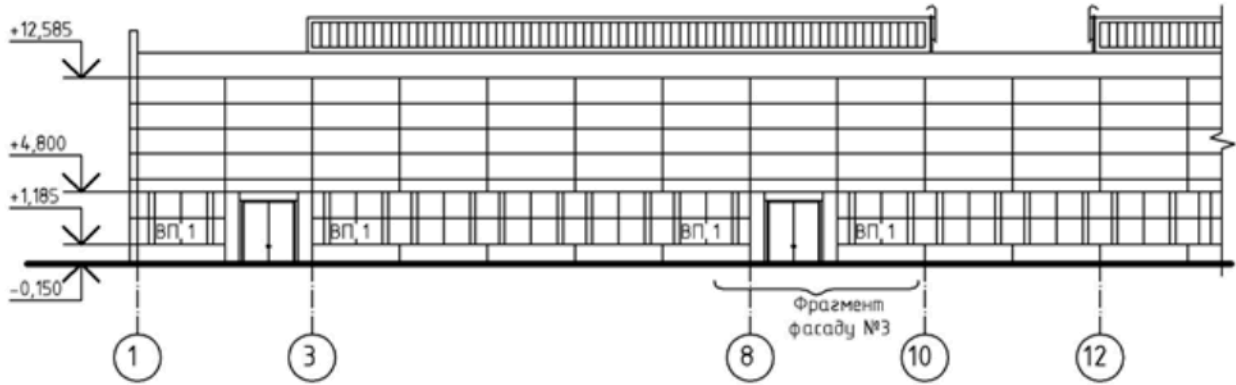
Фрагмент фасаду №3
