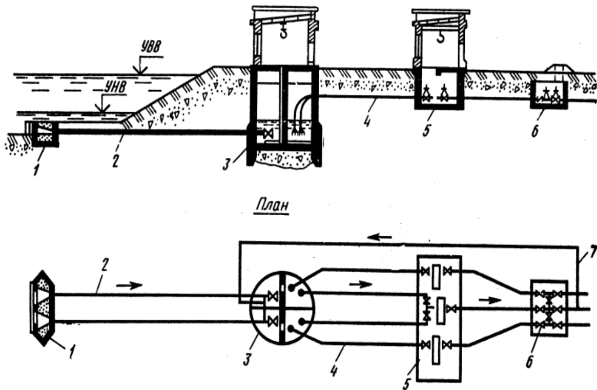
Рисунок 4.1 – Схема руслового водозабору з роз'єднаною компоновкою
