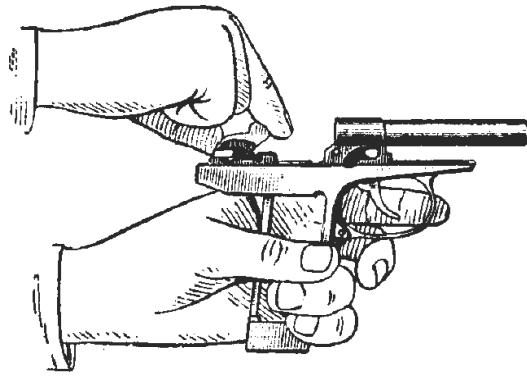
Мал. 21. Приєднання курка до рамки
