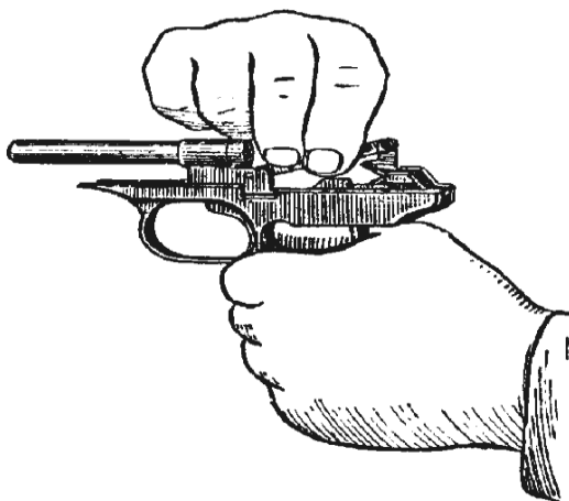
Мал. 14. Відділення спускової тяги з важелем зводу від рамки
