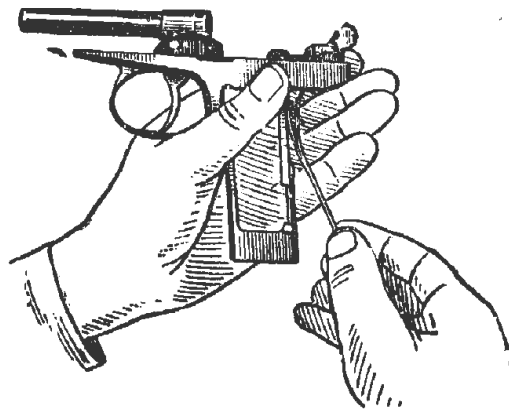
Мал. 22. Приєднання бойової пружини до рамки
