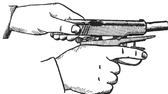
Мал. 5. Відділення затвора від рамки
