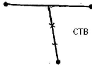
Мал. 51. Визначення середньої точки влучення по трьох пробоїнах
