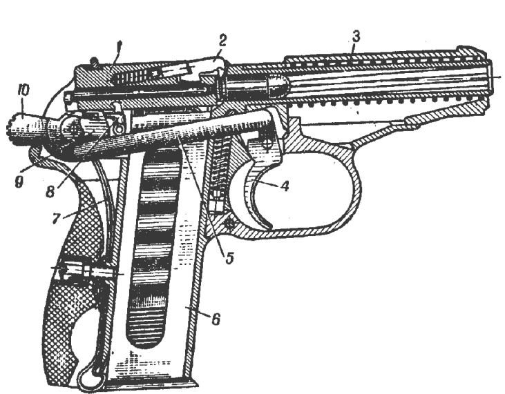
Мал. 46. Положення частин і механізмів пістолета перед пострілом:
