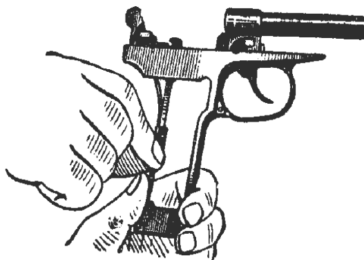
Мал. 23. Закріплення бойової пружини здвижки
