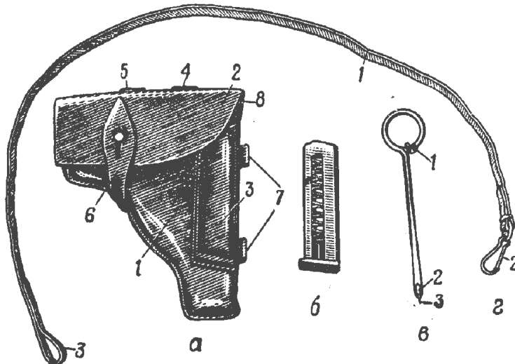
Мал. 44. Приладдя до пістолета
