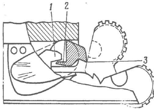
Мал. 48. Схема блокування курка виступом запобіжника:
