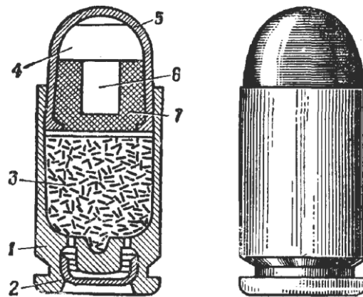
Мал. 45. Загальний вигляд 9-мм пістолетного патрону та його будова:
