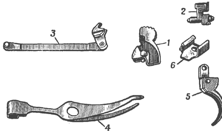
Мал. 31. Ударно-спусковий механізм:
