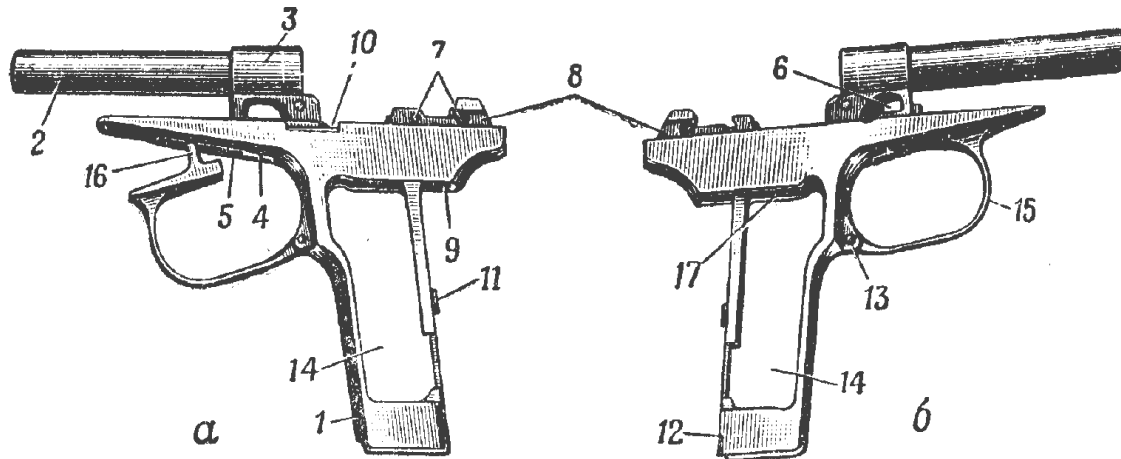
Мал. 25. Рамка зі стволом і спусковою скобою:
