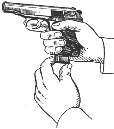
Мал. 8. Вставлення магазину в основу рукоятки
