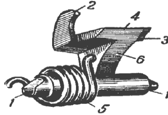
Мал. 33. Шептало:
