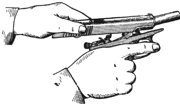
Мал. 7. Приєднання затвора до рамки
