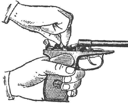
Мал. 10. Відділення шептала і затворної затримки від рамки
