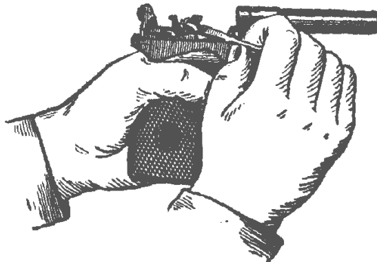
Мал. 9. Зняття гачка пружини шептала з затворної затримки
