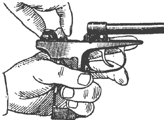
Мал. 13. Відділення курка від рамки
