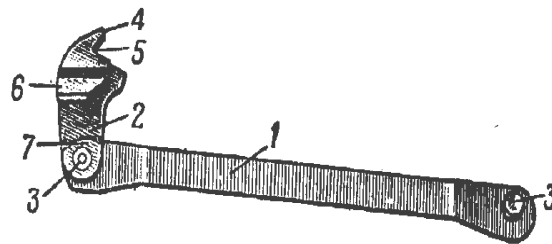
Мал. 34. Спускова тяга з важелем зводу:
