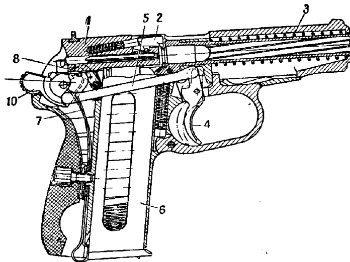
Мал. 47. Положення частин і механізмів пістолета перед пострілом самовзводом:
