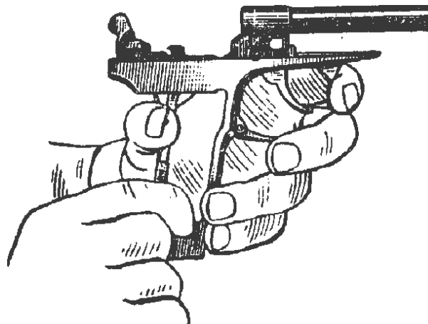
Мал. 12. Відділення бойової пружини від рамки
