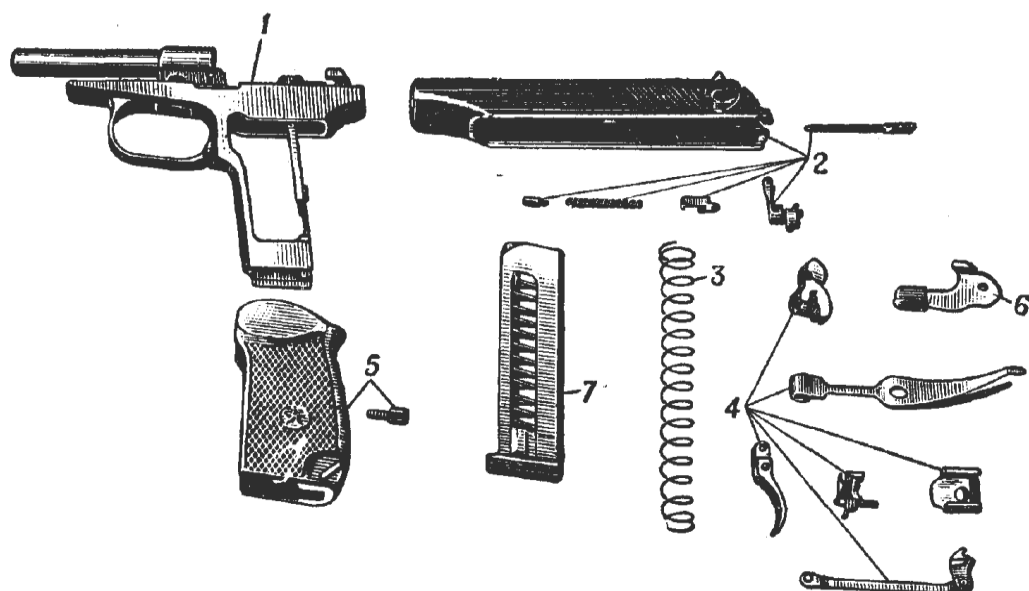
Мал. 2. Основні частини і механізми пістолета:
