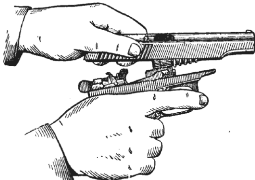
Мал. 6. Введення вільного кінця зворотньої пружини в канал ствола
