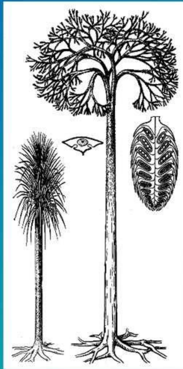
Лепідодендрон
