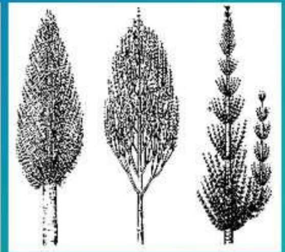
Викопні хвоці
