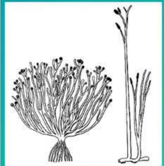
Риніюфіти
