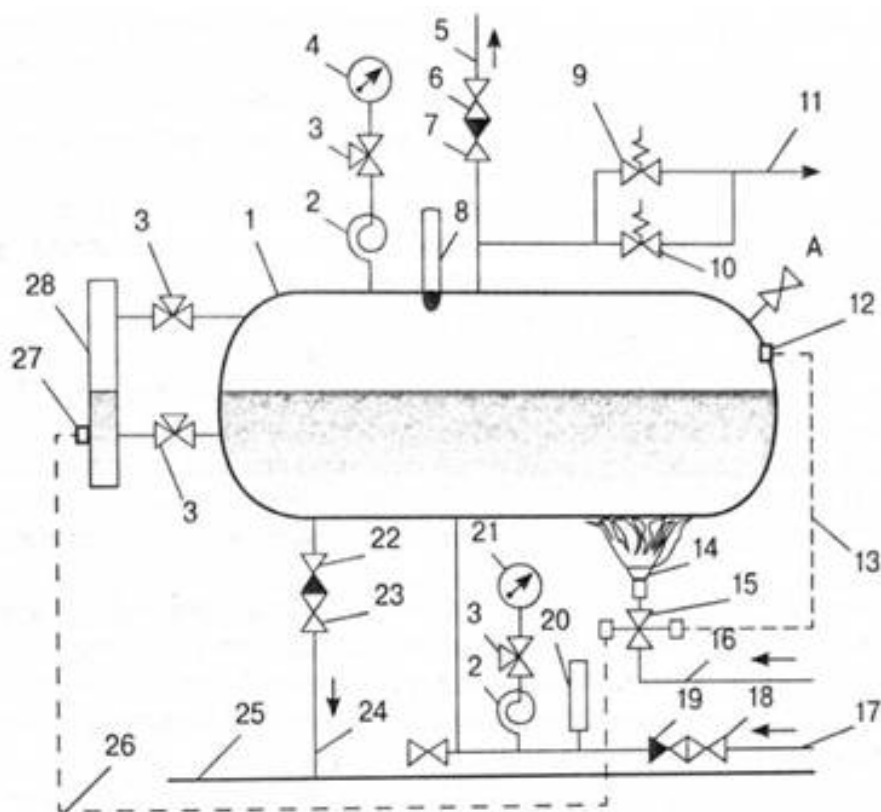
Рисунок 2.1 – Схема установки, що працює під тиском
