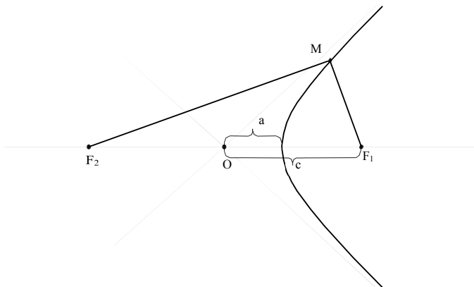
Рис. 3.4. Схематичне зображення гіперболи
