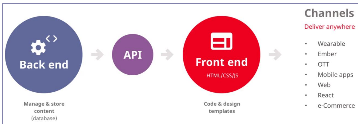
Рис. 2 – Загальна архітектура розділених (decoupled) CMS
