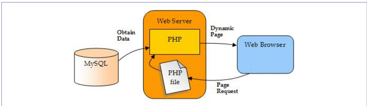
Рис. 15. Загальна структура внутрішньої організації системи керування контентом
