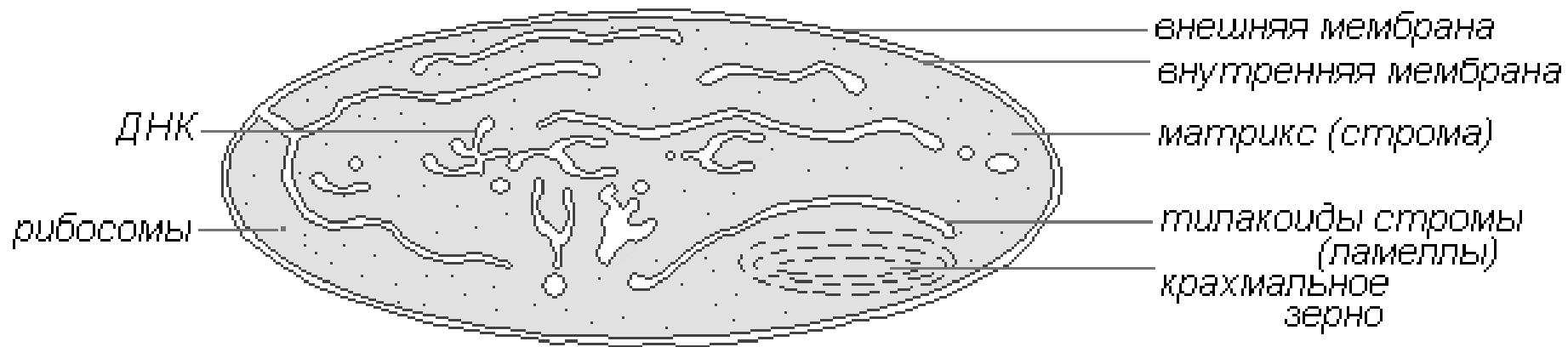
Строение лейкопласта
