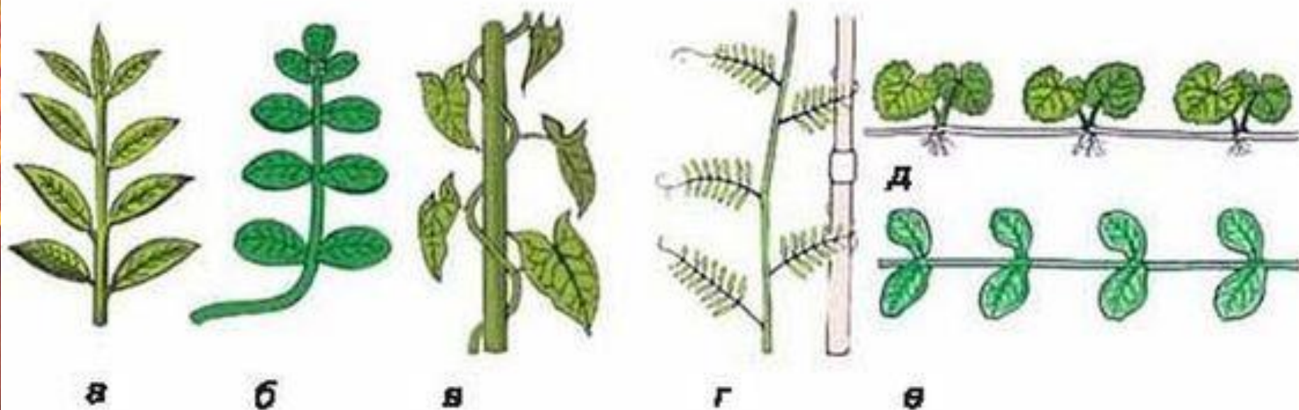
Мал. 94. Типи пагонів: а — прямостоячий; б — висхідний; в — витюй; г — чіпкий; д — повзучий; е — сланкий
