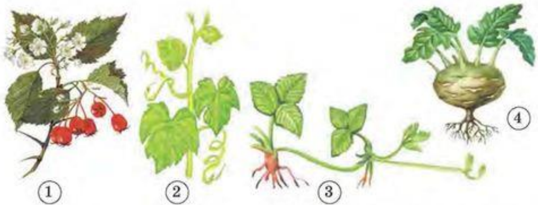
Мал. 114. Видозміни надземних пагонів:
