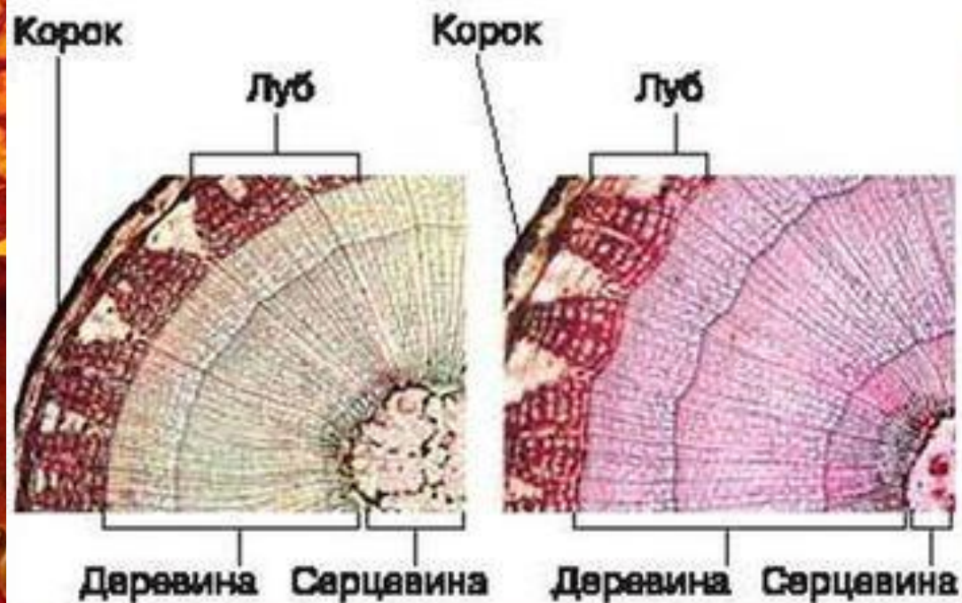
Мал. 100. Поперечні зрізи гілок липи різного віку
