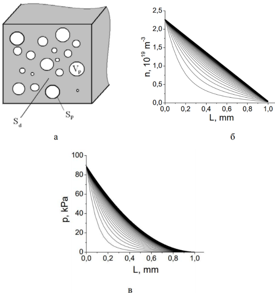
Рисунок 3.2 - Модель розрахунку проникності в полі пор (а) і профілі концентрації у розчині (б) і тиску в порах (б) у різні моменти часу
