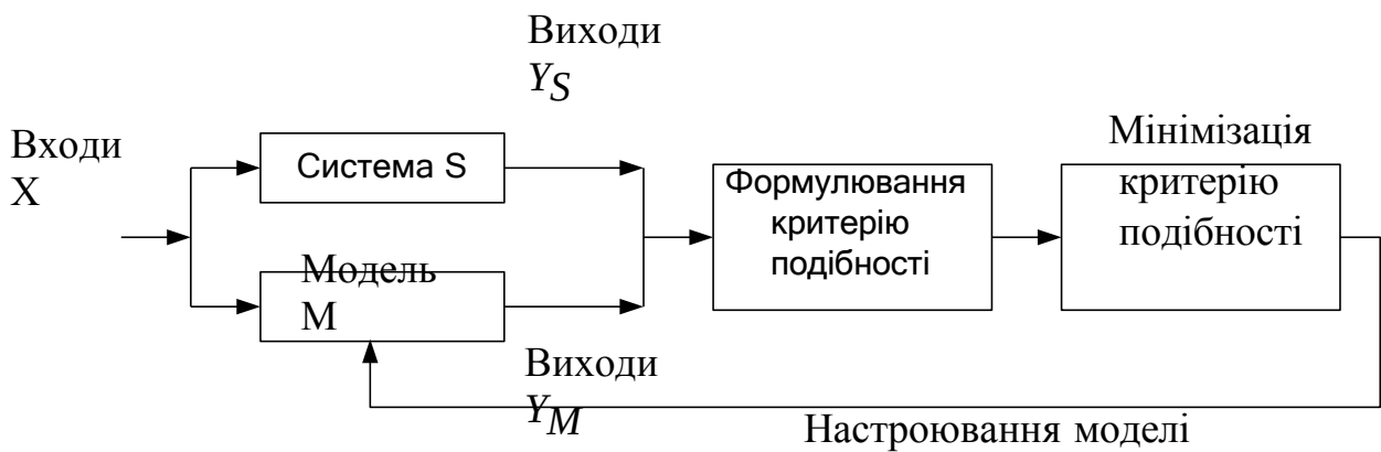
Рис. 4.1. Загальна схема ідентифікації моделі
