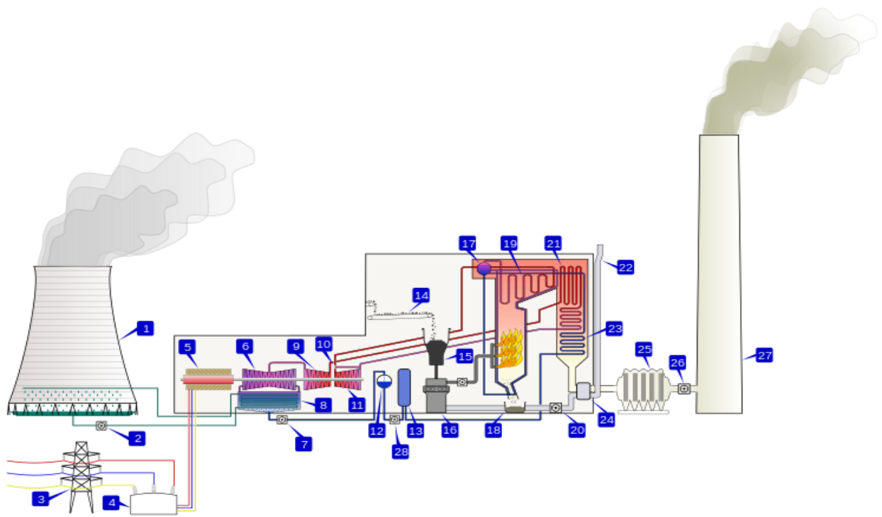
Типова схема теплової електричної станції, що працює на вугіллі
