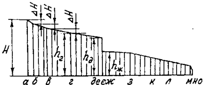
Рисунок 1.1.8 – Епюра фільтраційних напорів на флютбет, побудована за допомогою гідродинамічної сітки
