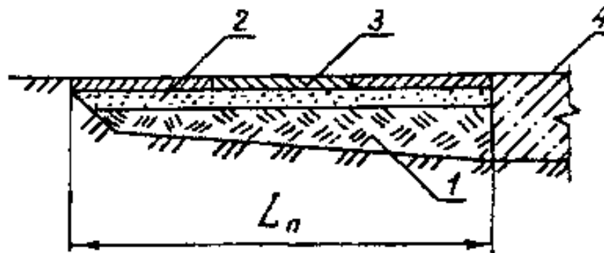
1 – ущільнений ґрунт; 2 – шар піску; 3 – залізобетонні плити; 4 – водобій
