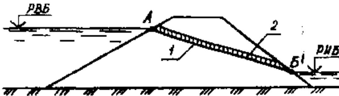
1 – крива депресії; 2 – капілярна зона.
