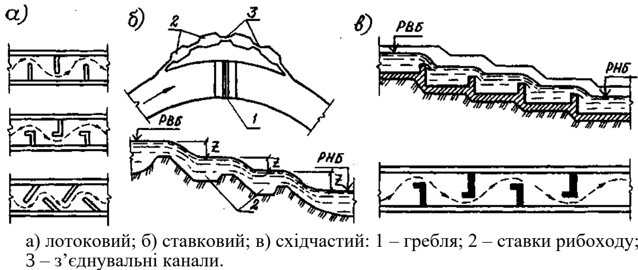
Рисунок 1.6.9 – Схеми рибоходів
