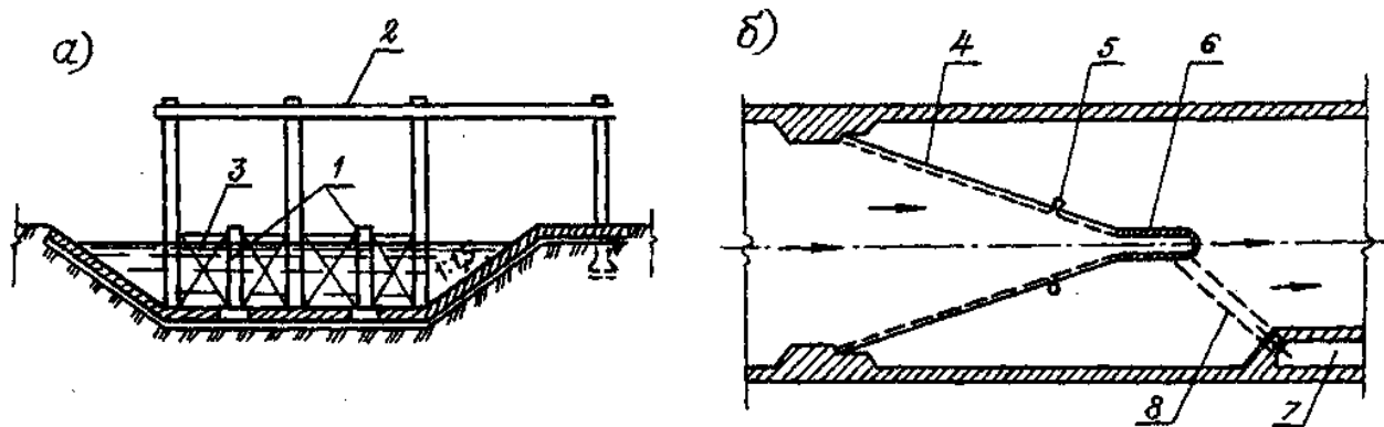
а) касетні фільтри; б) плоска сітка: 1 – естакада; 2 – монорейка; 3 – сіткові касети; 4 – сітка; 5 – флейта; 6 – рибонакопичувач; 7 – скидний лотік; 8 – рибовідвід.
