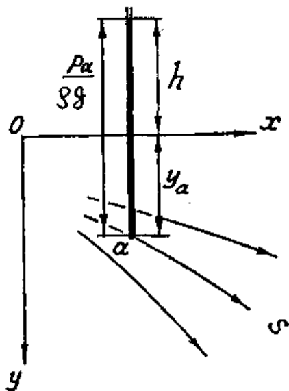
Рисунок 1.1.6 – Плоска картина руху ґрунтового потоку
