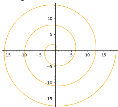
Рисунок 8.4 – Спіраль Архімеда
