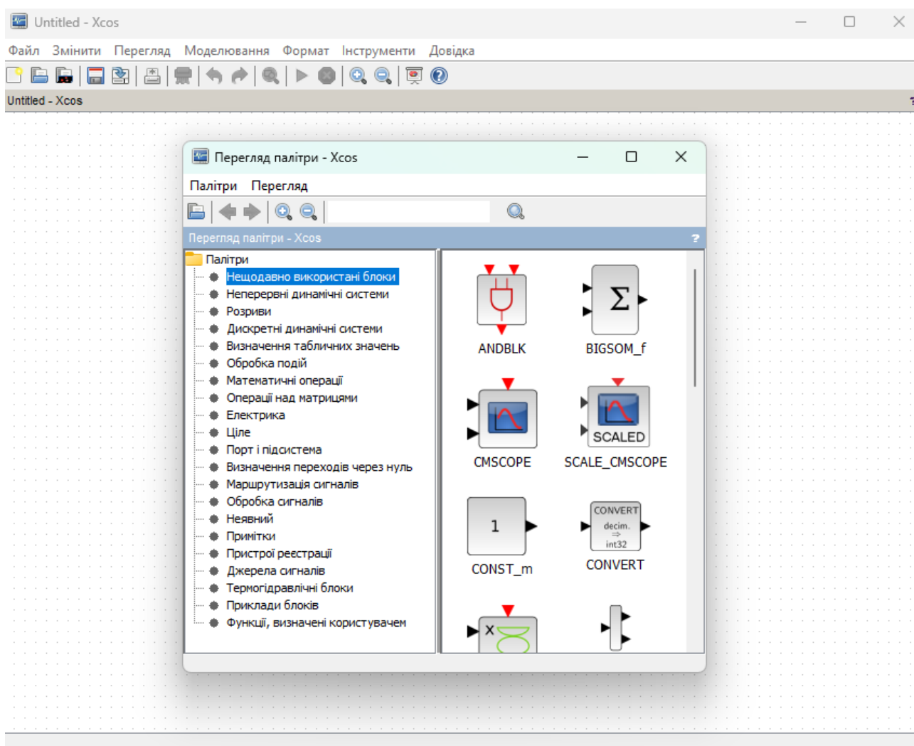
Рисунок 9.2 – Інтерфейс Xcos
