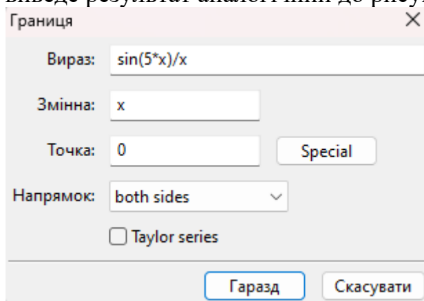
Рисунок 2.7 – Вікно «Границя»
