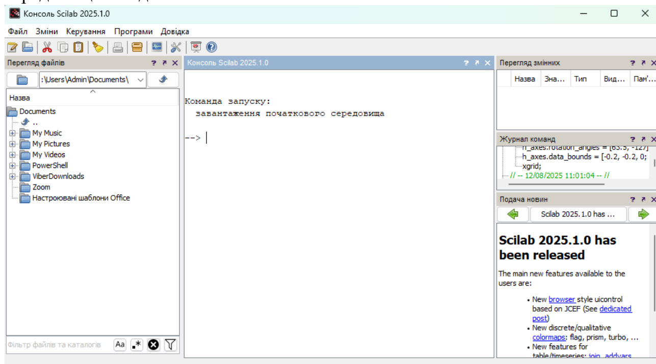
Рисунок 9.1 – Інтерфейс Scilab
