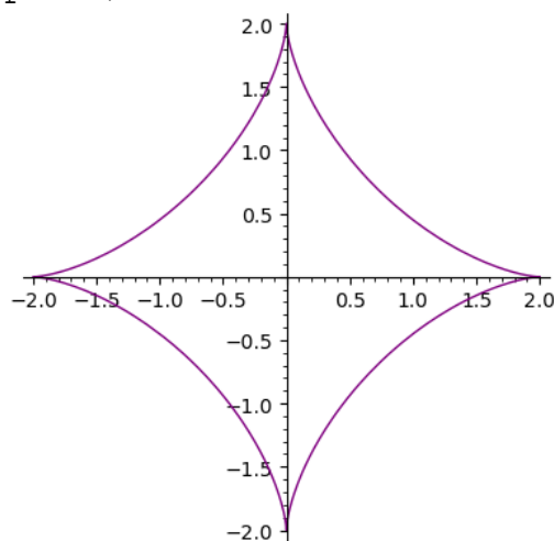
Рисунок 8.3 – Астроїда
