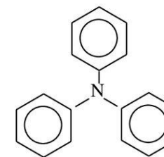
Трифеніламін (третинний)
