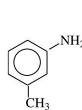
м-Толуїдин (первинний)
