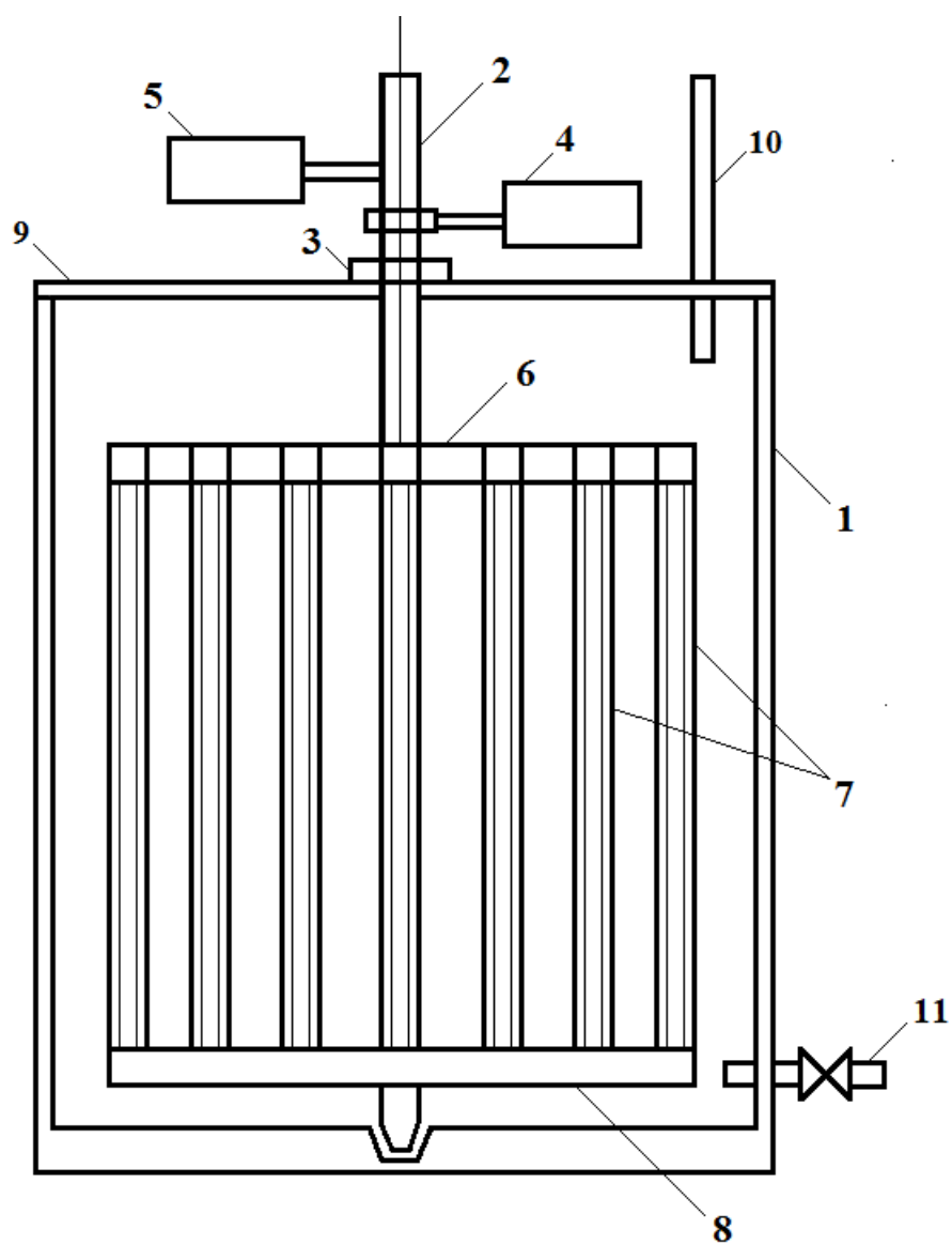
Фіг.1. Пристрій для інтенсифікації процесу утворення газу в реакторі
