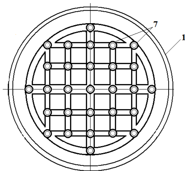
Фіг. 2. Пристрій для інтенсифікації процесу утворення газу в реакторі
