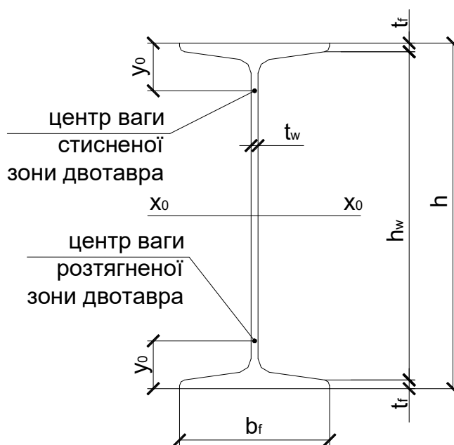
Схема А.1 – Переріз балки, яка підсилюється
