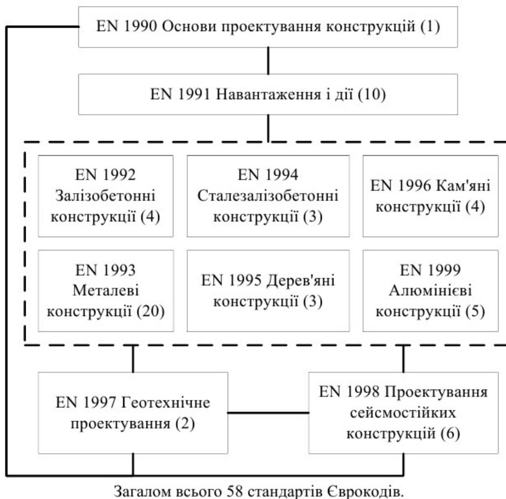
Рисунок 1.2 – Система Єврокодів
