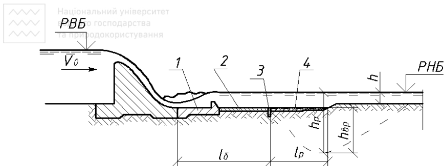
Рис. 4.29. Схема до розрахунку глибини розмиву русла в нижньому б'єфі 1 – водобій; 2 – рисберма; 3 – зуб; 4 – кінцеве кріплення у вигляді гнучкої рисберми
