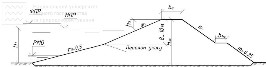
Рис. 1.4. Схема до вибору коефіцієнтів закладання укусів
