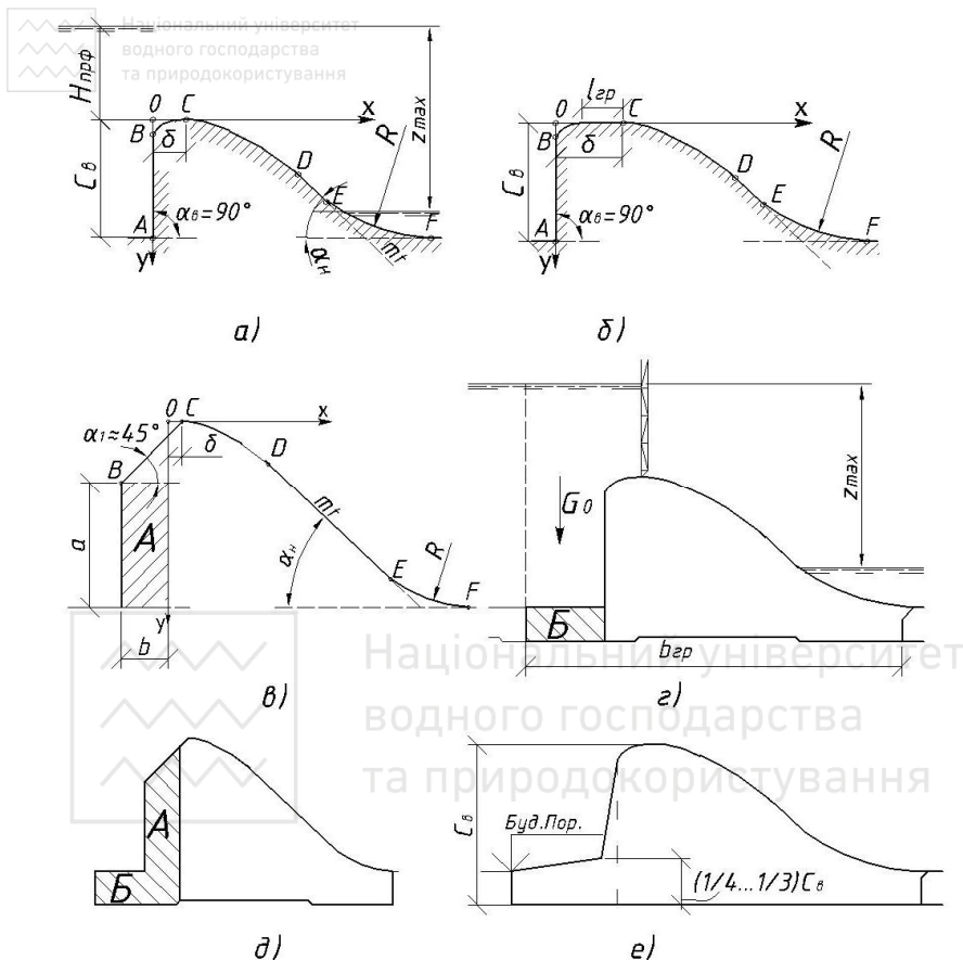
Рис. 4.4. Приклади практичних профілів без вакуумної водозливної стінки а) з вертикальною гранню; б) з горизонтальною вставкою; в) збільшеного перерізу з похилою вставкою; г) з консоллю фундаментної плити; д) при поєднанні прийомів в, г; е) при влаштуванні тимчасового будівельного порогу
