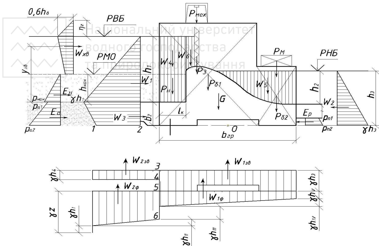
Рис. 4.32. Схема силових дій на греблю з ґрунтовим понуrom
