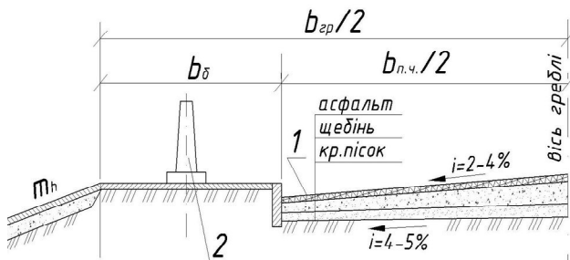
Рис. 1.5. Гребінь греблі: 1 – покриття гребеня; 2 – надовбні
