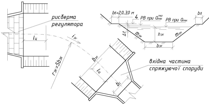
Рис. 2.13. З'єднувальний канал
