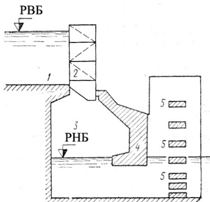
Рис. 5.1. Головна система з камерою гасіння: 1 – поріг; 2 – затвор; 3 – камера гасіння; 4 – екран; 5 – балкові гасителі
