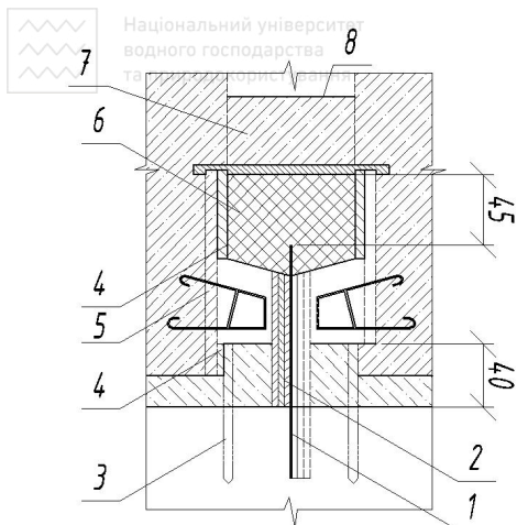
Рис. 4.11. З'єднання шпунта з фундаментною плитою за допомогою шпонки
