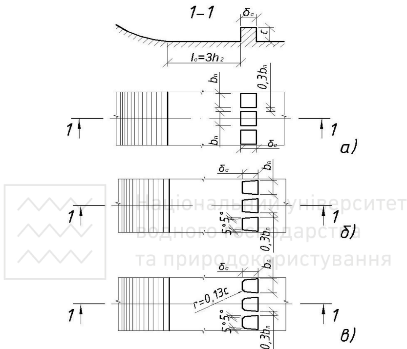
Рис. 4.23. Прорізна водобійна стінка
