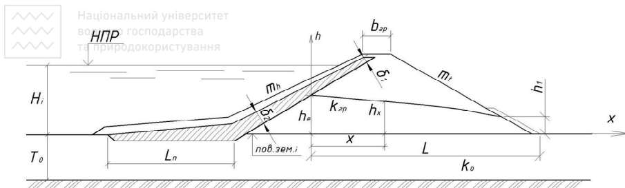
Рис. 1.29. Схема до розрахунку фільтрації через неоднорідну греблю з екраном і понуrom та приставним дренажем
