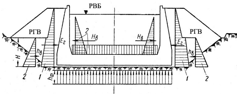
Рис. 5.3. Схема до статичного розрахунку камери:
