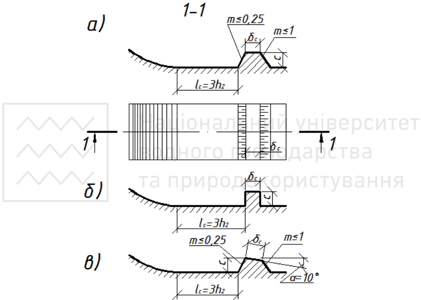
Рис. 4.18. Суцільна водобійна стінка
