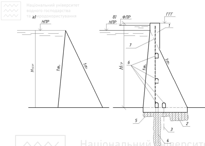
Рис. 3.2. Перетворення теоретичного профілю греблі в реальний:
