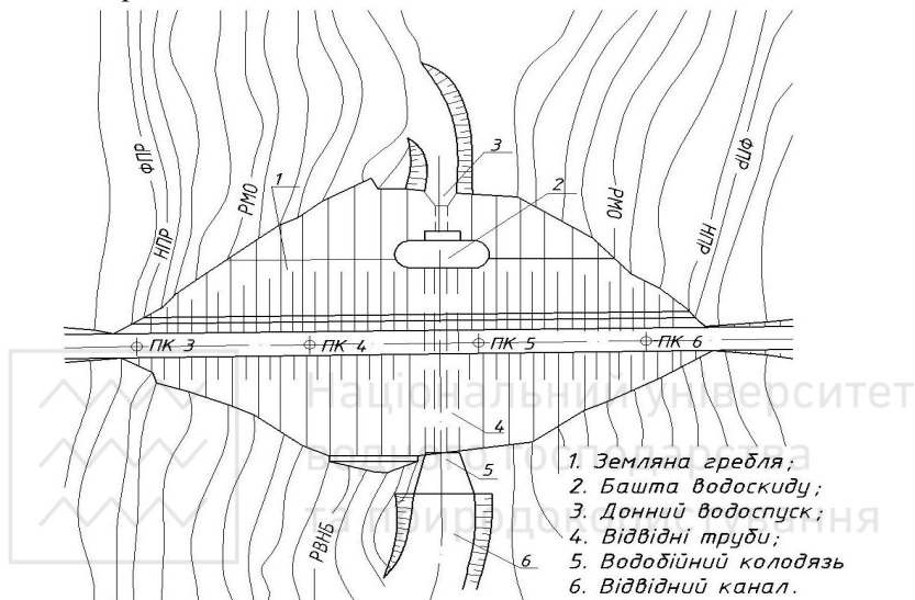
Рис. 1.1. План гідровузла з баштовим водоскидом
