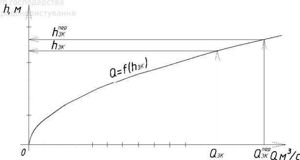
Рис. 2.14. Крива залежності Q=f(h_{зк}) для з'єднувального каналу
