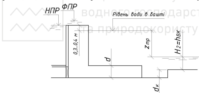
Рис. 2.27. Схема до розрахунку відвідних труб водоскиду
