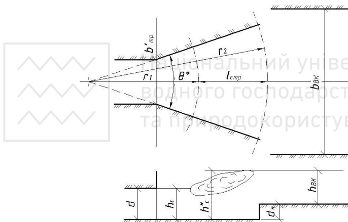
Рис. 2.28. Схема до розрахунку спряження б'єфів
