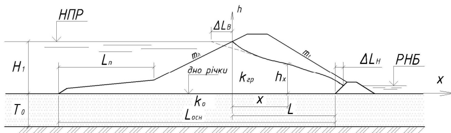
Рис. 1.26. Схема до розрахунку фільтрації через однорідну греблю з понуrom
