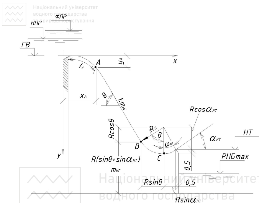
Рис. 3.9. Схема до побудови профілю водозливної греблі. Розміри вказані в метрах
