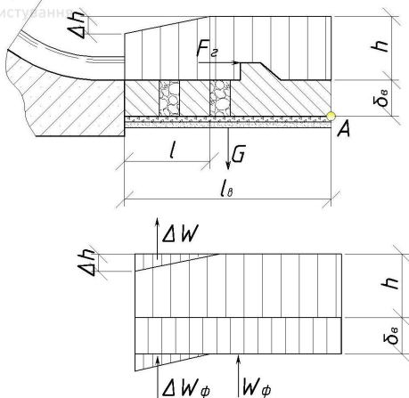
Рис. 4.34. Схема до визначення товщини водобійної плити
