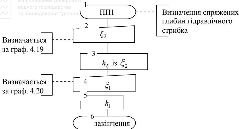
Рис. 4.22. Блок-схема підпрограми ППІ визначення спряжених глибин гідравлічного стрибка
