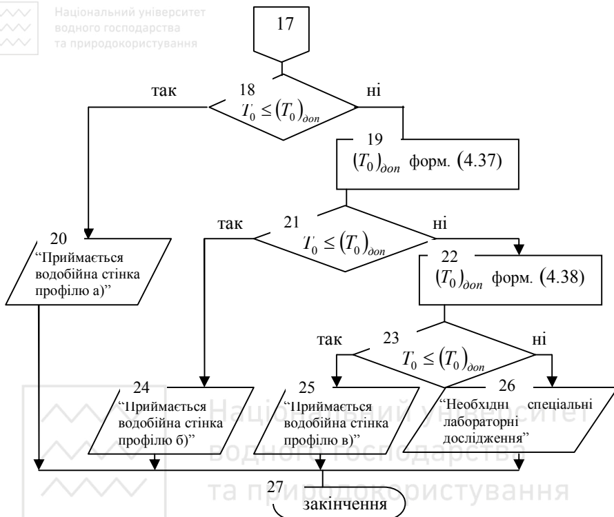
Рис. 4.25. Блок – схема алгоритму розрахунку прорізної водобійної стінки
