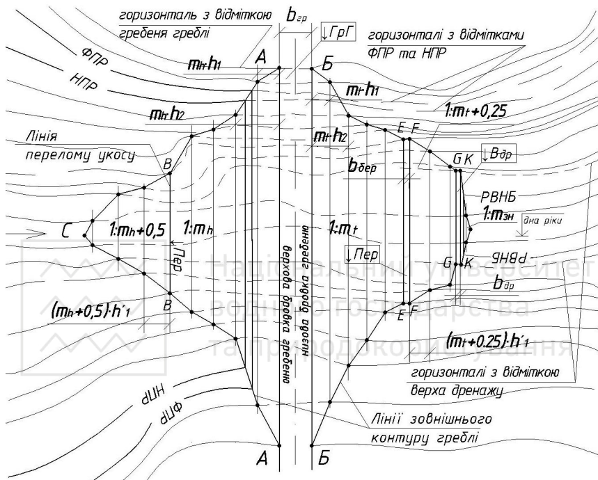
Рис. 1.19. Побудова греблі на плані
