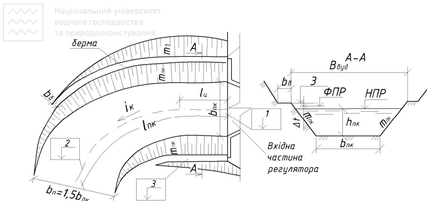
Рис. 2.12. Підвідний канал
