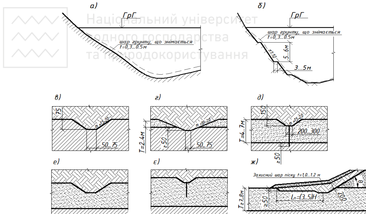
Рис. 1.17. Спряження греблі з берегами і основою а) при пологих берегах; б) при крутих берегах та скельній основі; в) зуб; г) замок; д) зуб з шпунтом; е) “вісячий” зуб; є) “вісячий” шпунт; ж) понур
