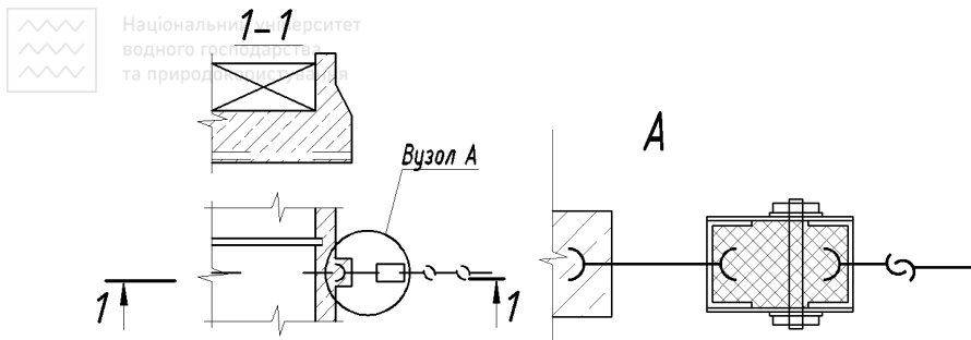
Рис. 4.15. Спряження діафрагми (шпори) із стояном
