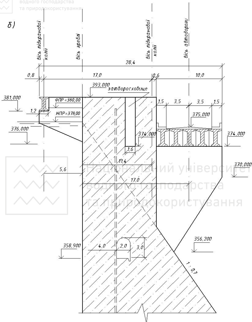
Рис. 3.3, б. Приклад конструкції гребня глухої греблі з затворосховищем і автодорогою, яка проходить за гребенем. Розміри вказано в метрах
