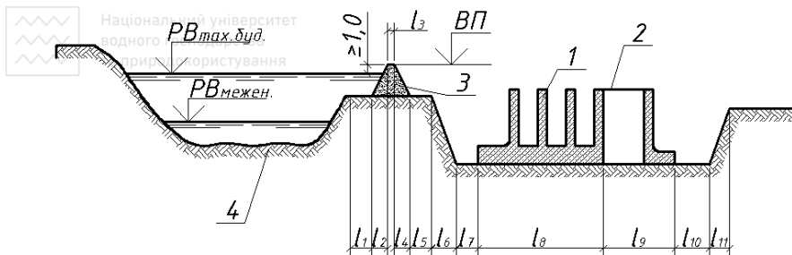
Рис. 4.3. Схема розташування водоскидних споруд гідровузла на заплаві річки 1 – водозливна гребля; 2 – будівля ГЕС; 3 – поздовжня перемичка; 4 – русло річки
