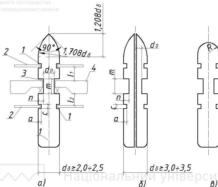
Рис. 3.11. Схеми биків в плані:
