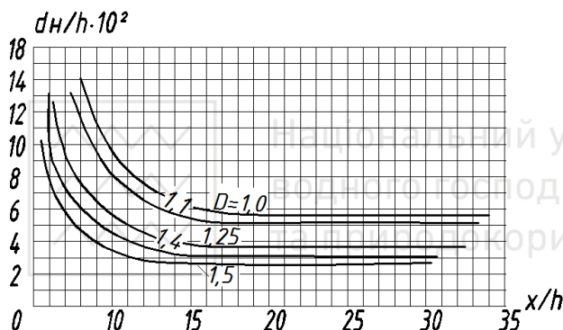
Рис. 4.27. Графіки для визначення крупності каменя гнучкої рисберми у випадку суцільної або прорізної водобійної стінки
