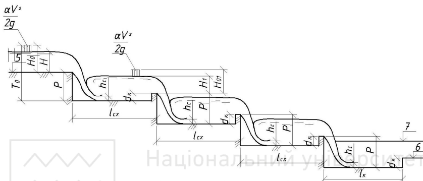
Рис. 2.18. Схема до гідралічного розрахунку багатосхідчастого перепаду
