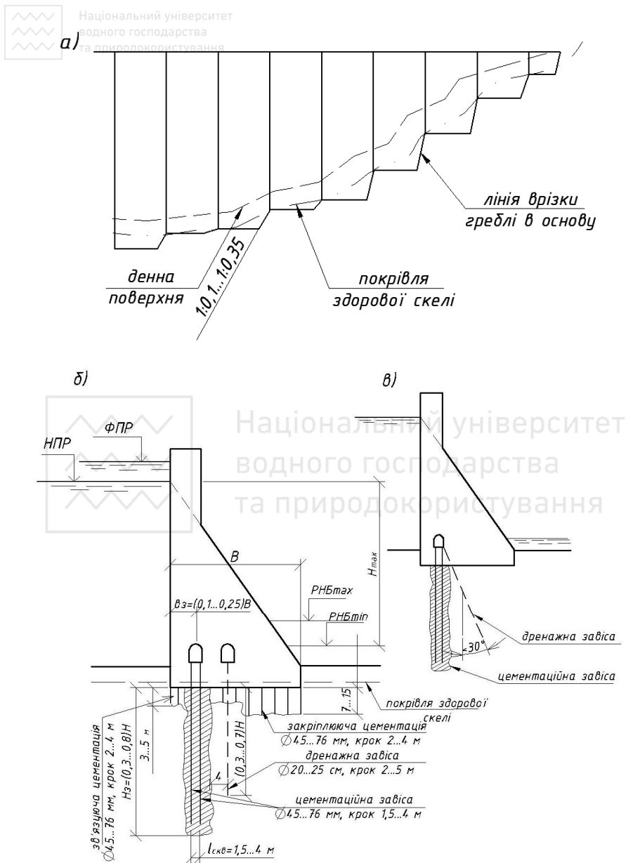
Рис. 3.8. Спряження греблі з основою і берегами:
