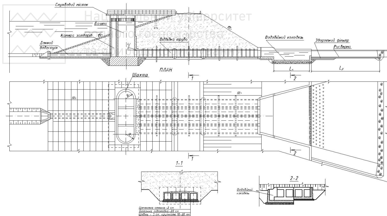
Рис. 2.26. Баштовий водоскид
