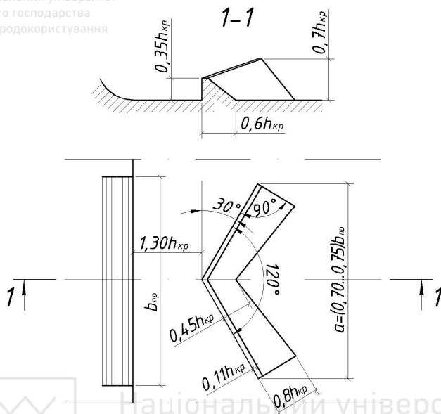
Рис. 4.26. Гаситель-розтікач Куміна
