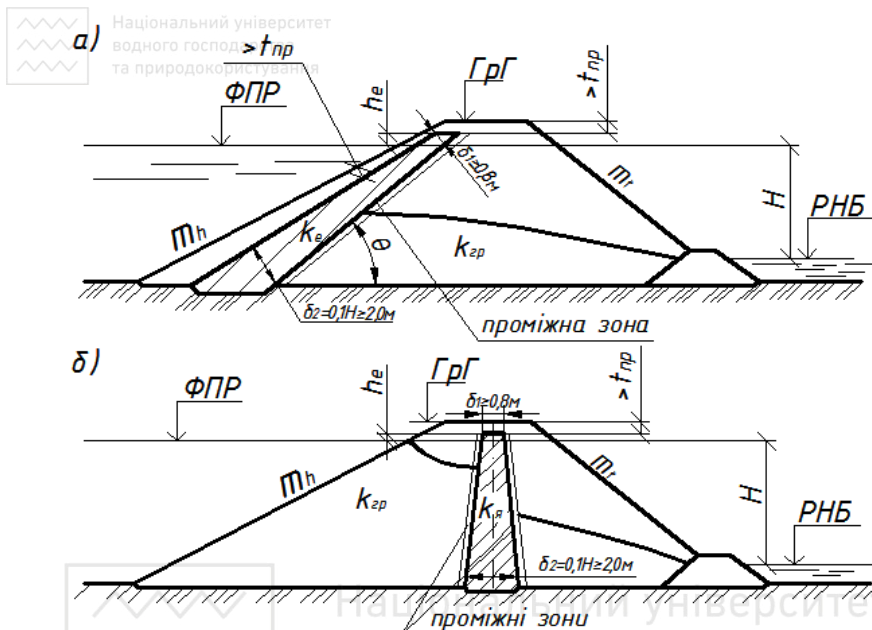
Рис. 1.16. Конструкція протифільтраційних пристроїв в тілі греблі а) екрану, б) ядра
