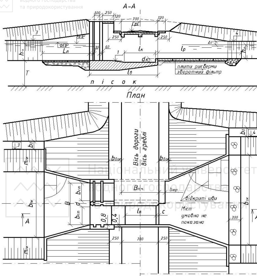
Рис. 2.7. Конструкція відкритого регулятора
