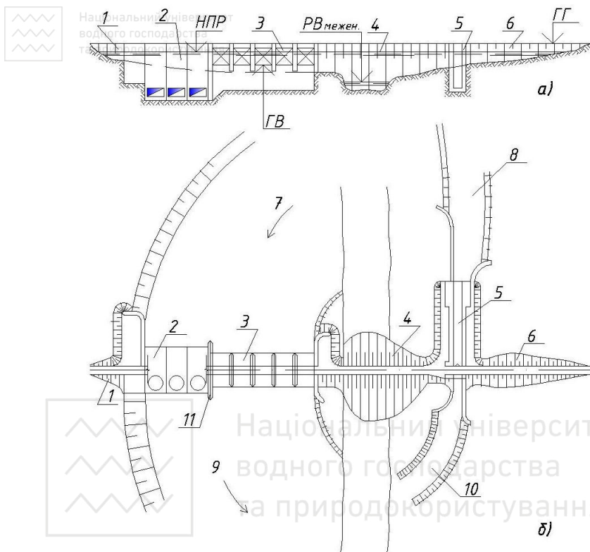
Рис. 4.2. Схема заплавної компоновки середньонапірного гідровузла: а) профіль по осі гідровузла; б) план 1, 4, 6 – ґрунтові греблі; 2 – будівля ГЕС; 3 – водозливна бетонна гребля; 5 – судноплавний шлюз; 7, 9 – підвідний і відвідний канали ГЕС; 8, 10 – підхідні канали до шлюзу; 11 – роздільна стінка
