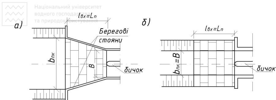
Рис. 2.4. Схеми спряження підвідного каналу із регулятором
