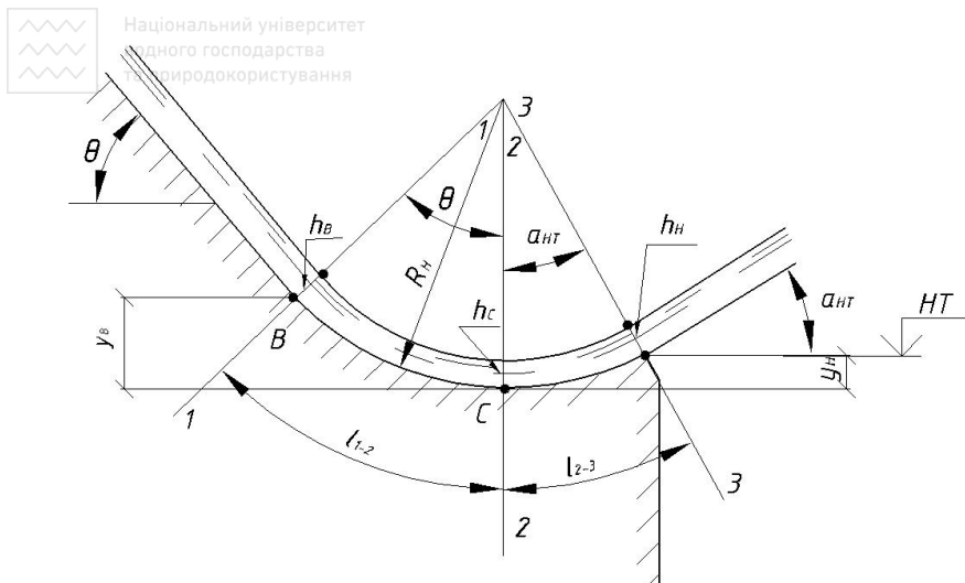
Рис. 3.17. Схема до визначення глибин потоку на носку-трампліні
