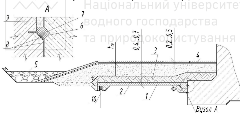
Рис. 4.10. Анкерний понур
