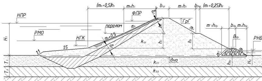
Рис. 1.18. Поперечний переріз греблі
