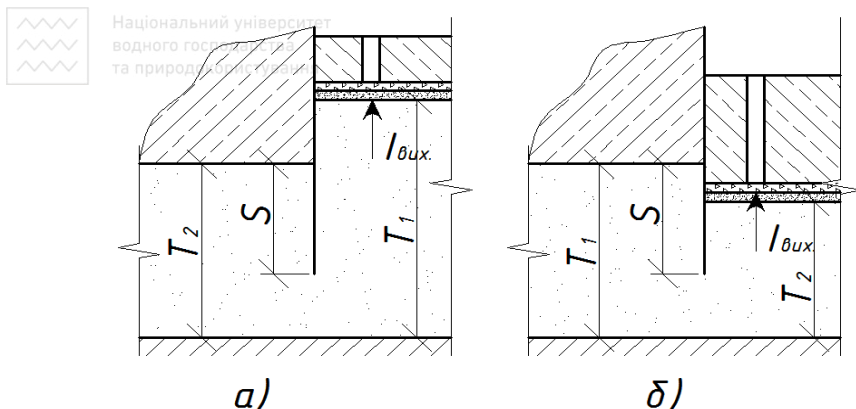
Рис. 4.31. Схеми виходу фільтраційного потоку в нижній б'єф
