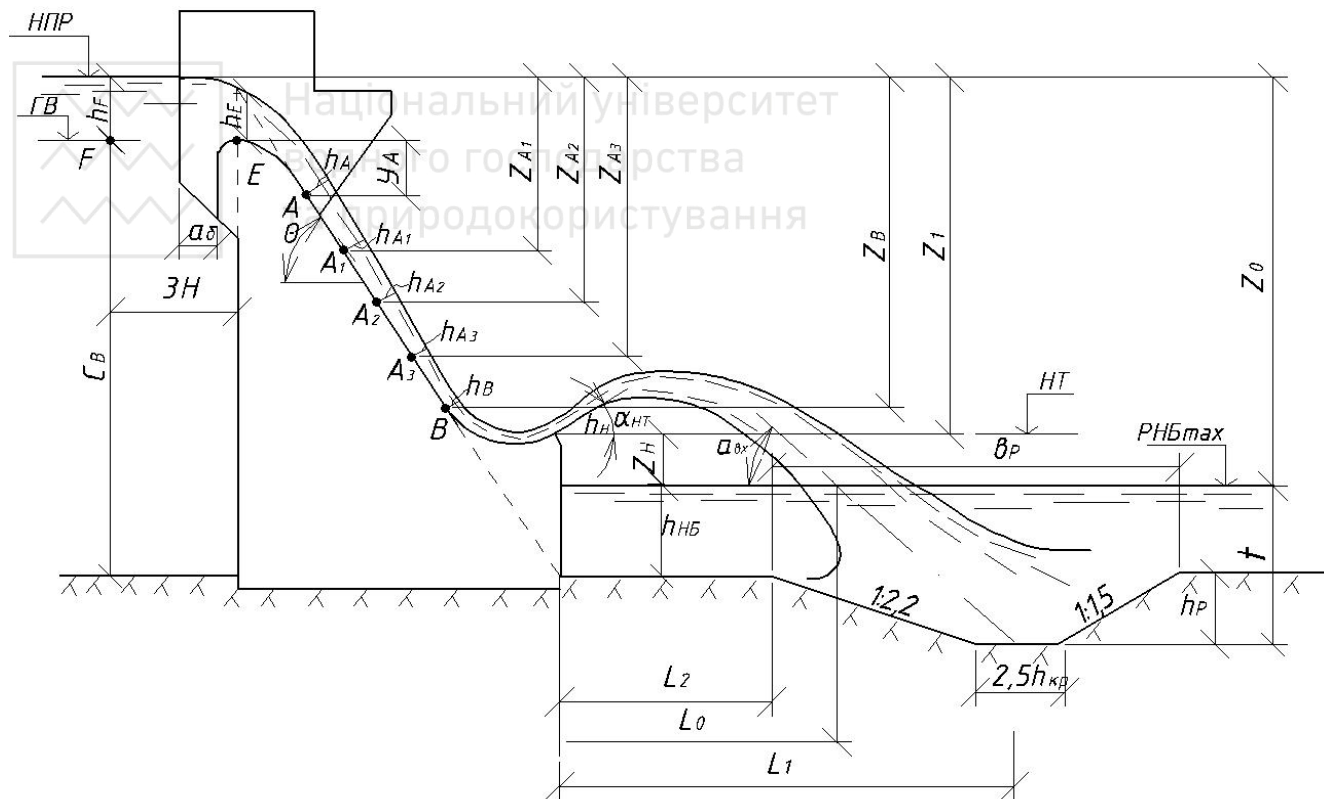
Рис. 3.15. Схема до гідравлічного розрахунку водозливної греблі
