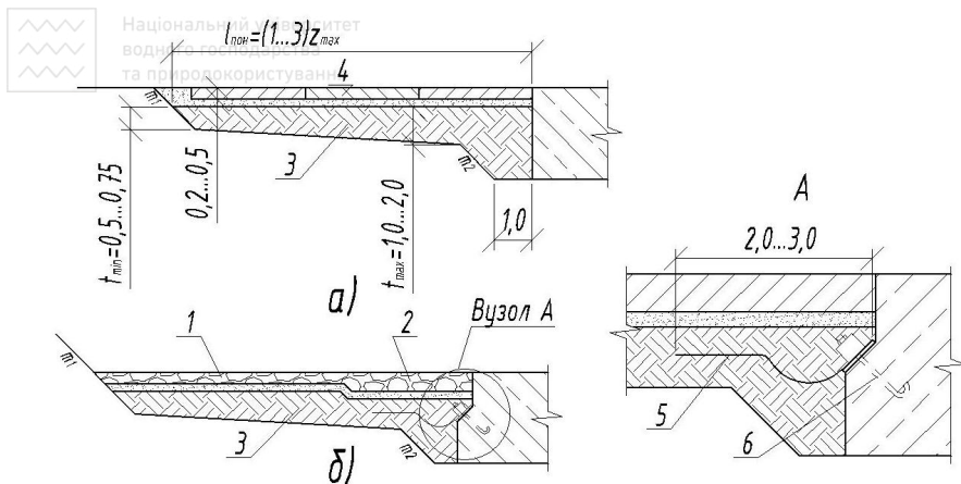
Рис. 4.9. Приклади гнучких глиняних понурів
