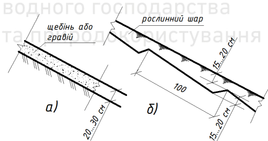
Рис. 1.13. Кріплення низового укосу: а) відсіпка щебеню; б) залуження
