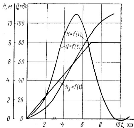
Рис. 5.2. Гідравлічна характеристика шлюзу
