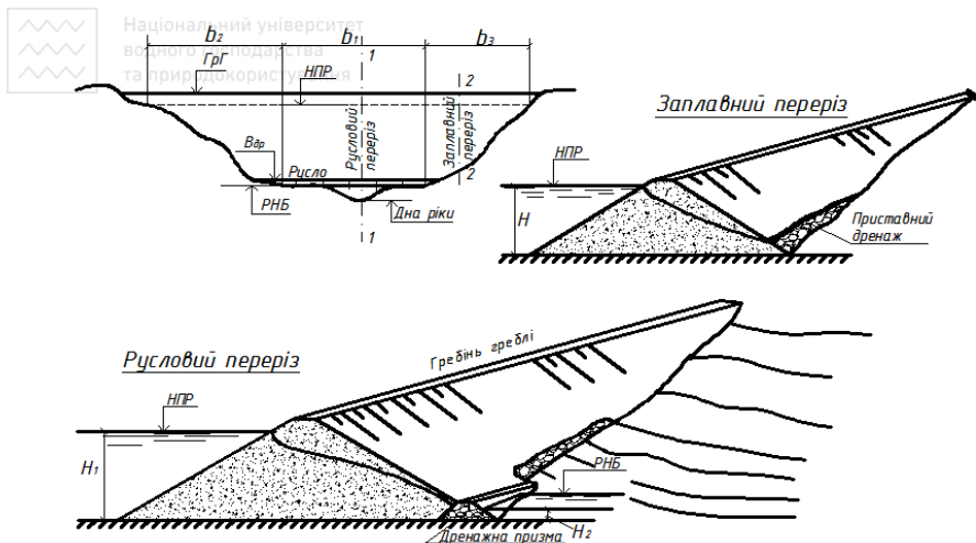
Рис. 1.20. Поздовжній профіль та поперечні перерізи тіла греблі
