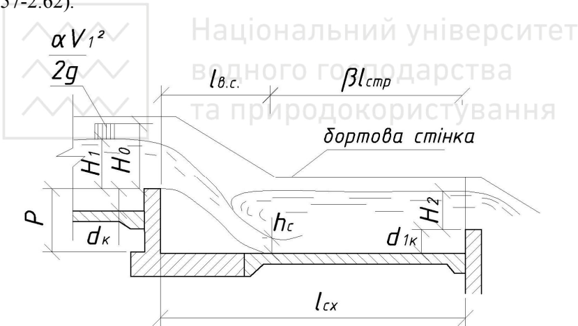
Рис. 2.21. Другий східць перепаду
