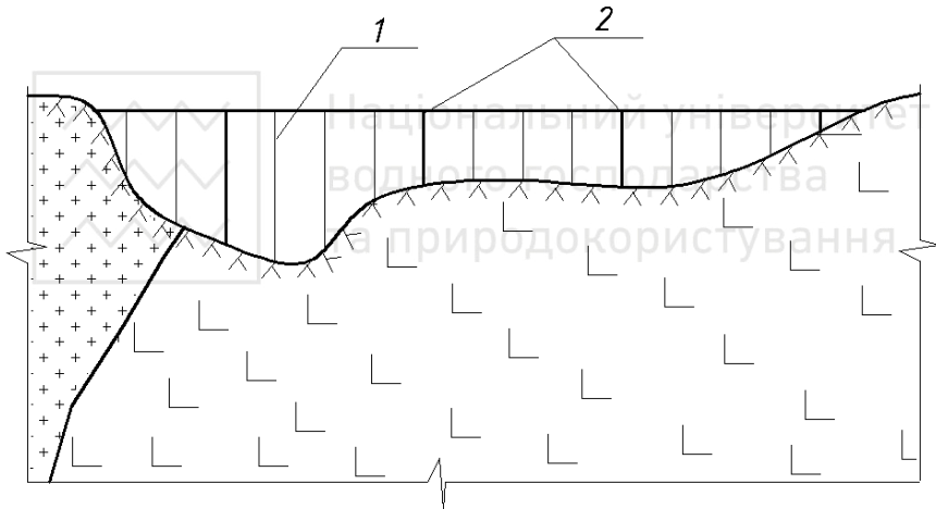
Рис. 3.4. Розміщення постійних температурних швів в греблі:
