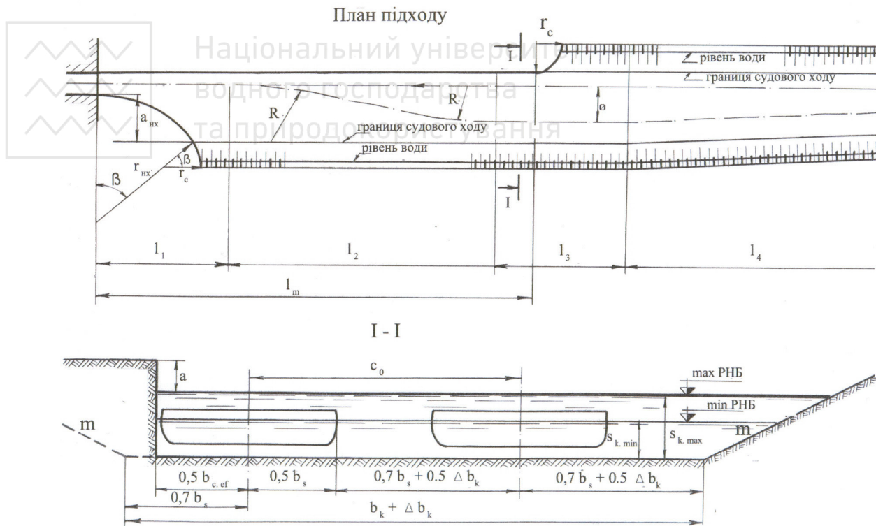
Рис. 5.5. План підходу і поперечний переріз каналу
