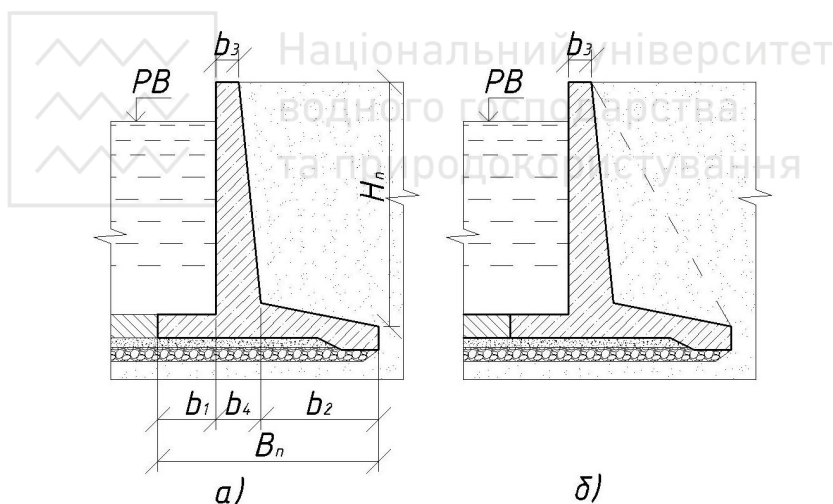
Рис. 4.16. Підпiрнi стiнки спрягаючих споруд а) кутикового типу; б) контрфорсного типу
