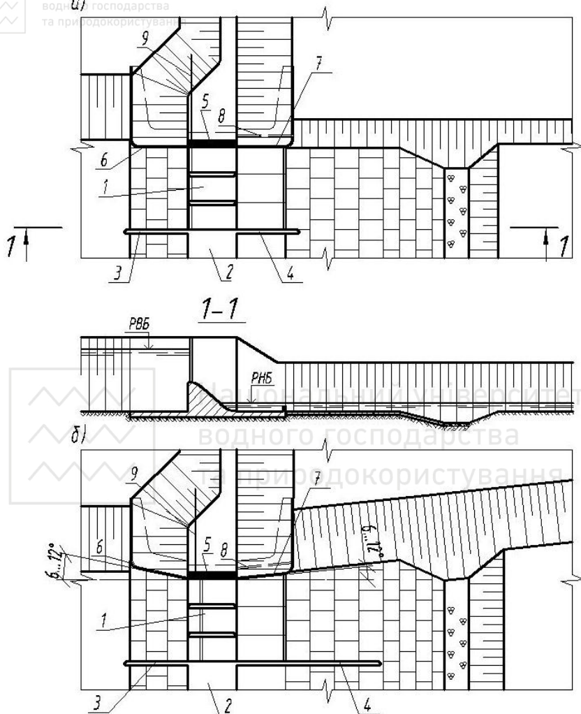
Рис. 4.14. Приклади компоновки спрягаючих споруд
