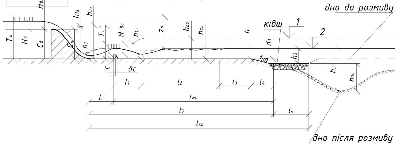
Рис. 4.17. Розрахункова схема поздовжнього профілю ділянки спряження б'єфів
