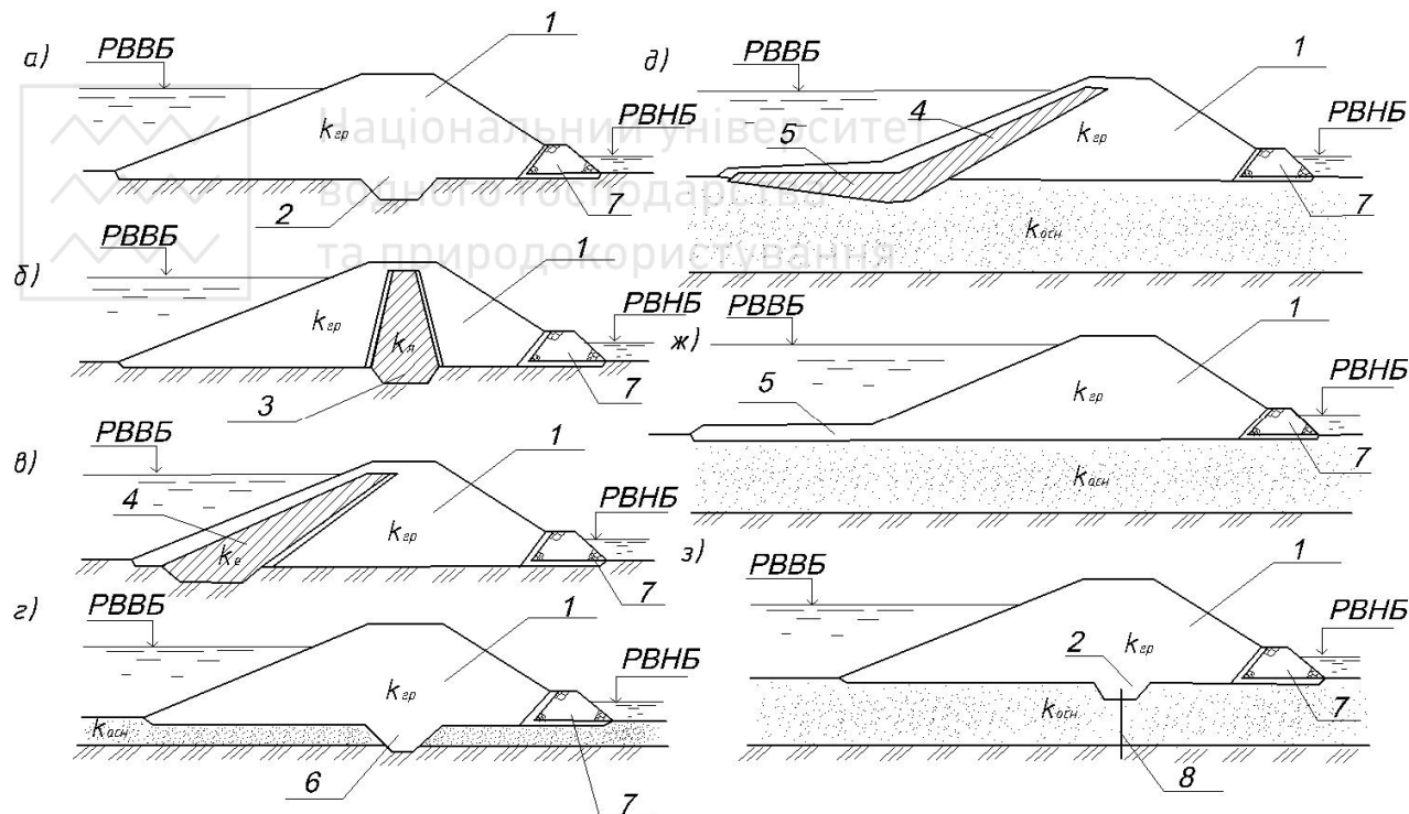
Рис. 1.15. Типи земляних насипних гребель 1 – тіло греблі, 2 – зуб, 3 – ядро, 4 – екран, 5 – понур, 6 – замок, 7 – дренаж, 8 – шпунт, PBBБ – рівень води верхнього б'єфу, PBNБ – рівень води нижнього б'єфу
