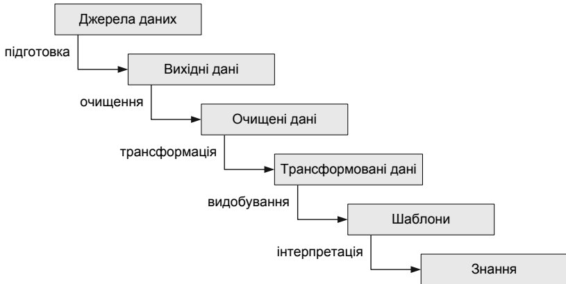
Рис. 4.3. Етапи KDD
