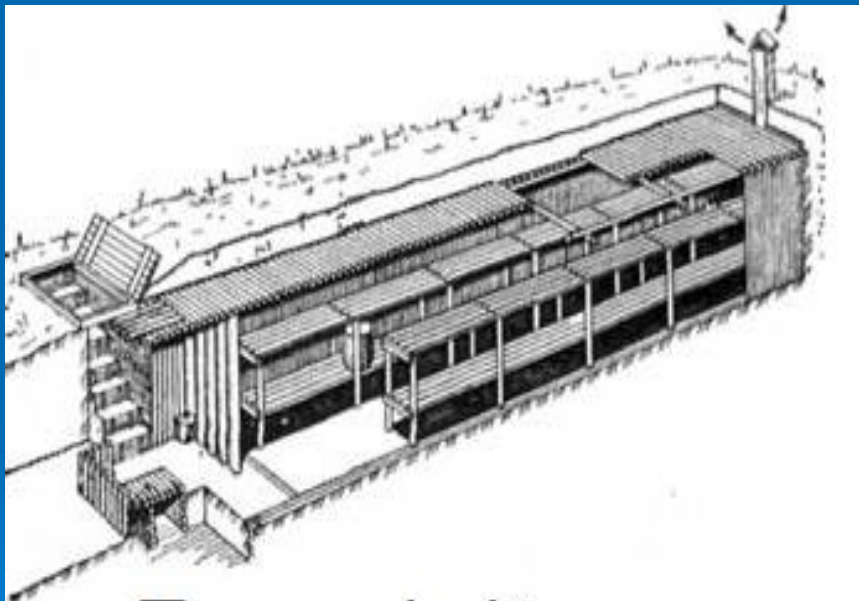
Протирадіаційне укриття з тонких колод або жердин
