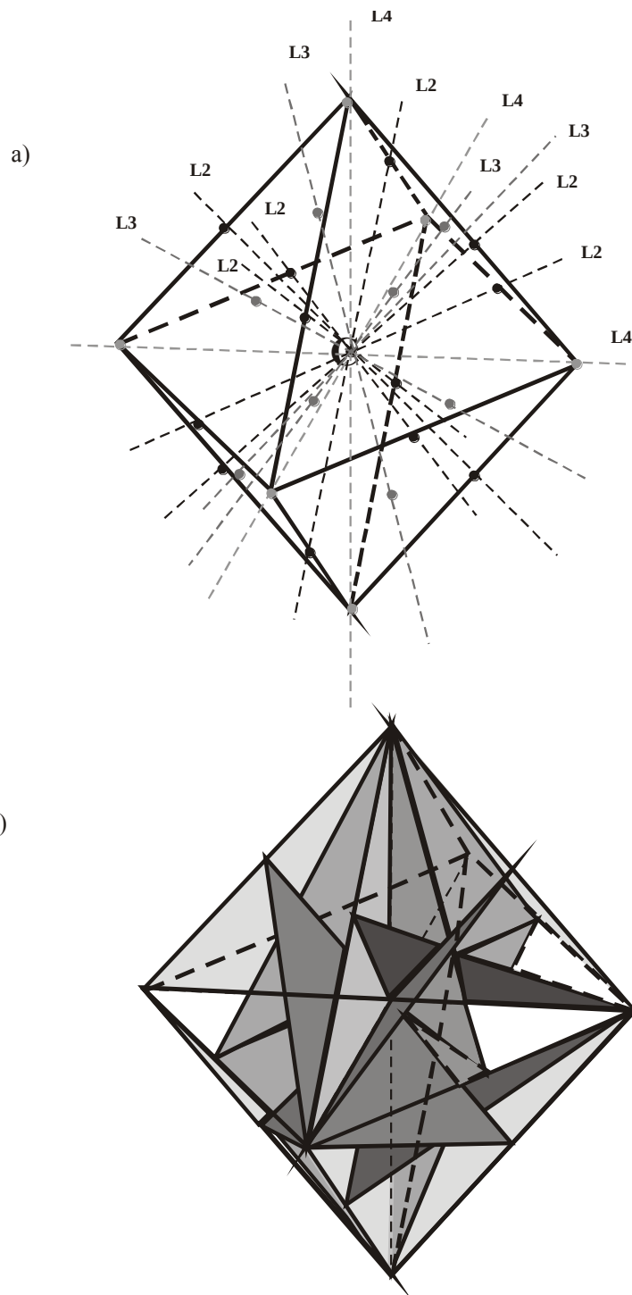
Рисунок 1.4 – Елементи симетрії октаедра
