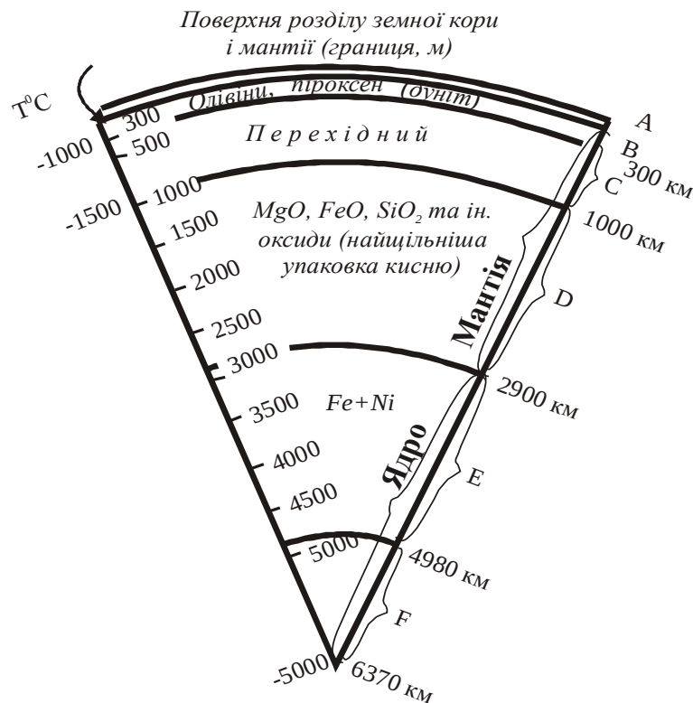
Рисунок 1.3 - Розріз земної кулі (по А.А. Виноградову): А - земна кора; В,С,Д - верхня, середня і нижня мантії; Е,Ф - зовнішнє і внутрішнє ядро
