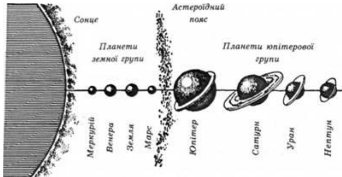
Рисунок 1.1 – Будова Сонячної системи
