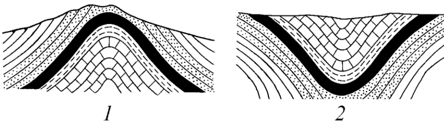
Рисунок 3.3 Антиклінальна (1) і синклінальна (2) складки
