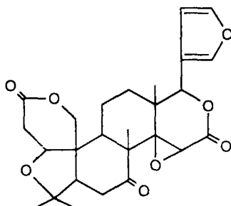
Лимонін
