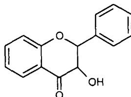
5 Флаванол
