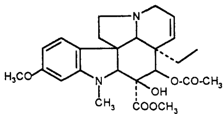
Віндолін
