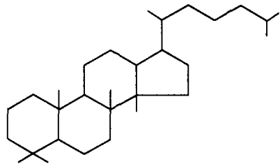
Дамаран
