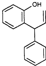
Неохалкон
