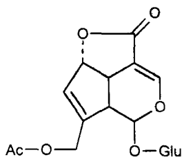
Асперулозид
