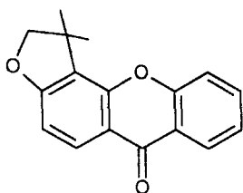
Фураноксантон
