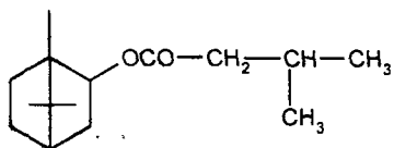
Борнілізовалеріанат
