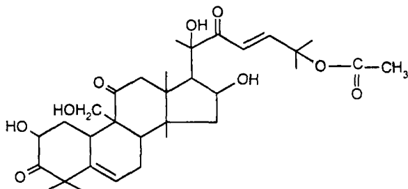
Кукурбітацин А
