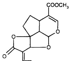
Плюмерицин
