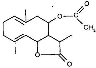
Ацетилбалхинолід
