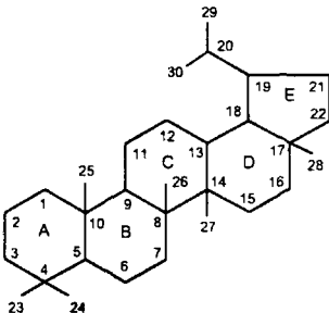
Лупан
