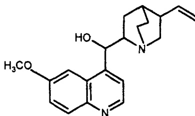
Хінін
