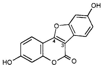
Куместрол
