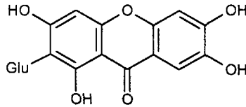
Мангіферин
