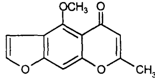
Віснагін
