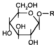
\beta -Глюкопіранозид
