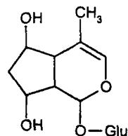
Деуціон
