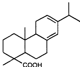
Левопімарова кислота
