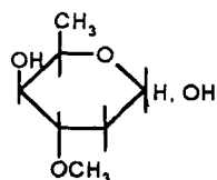
L-Олеандроза
