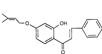
Кордоїн
