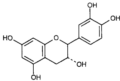
(-)-Катехін
