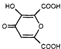
Меконова кислота
