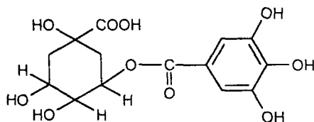
Теоралін
