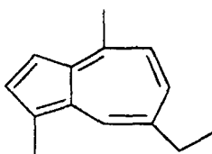
Хамазулен
