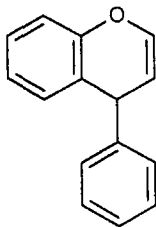
Неофлавіон
