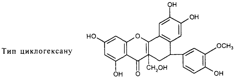
Неогіднокарпін
