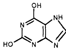
лактимна форма
