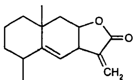
Алантолактон
