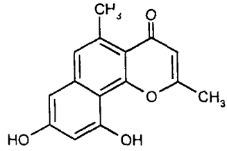
Елеутеринол
