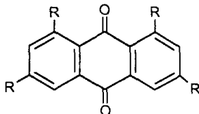
Антрахінони
