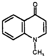
Ехінопсин
