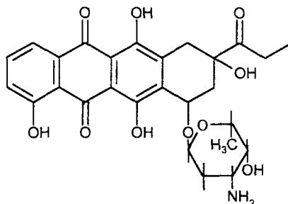
Карміноміцин
