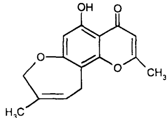
Птерокилін
