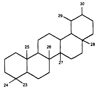
Урсан
