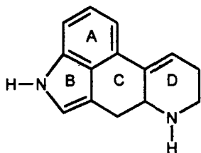
Ерголін
