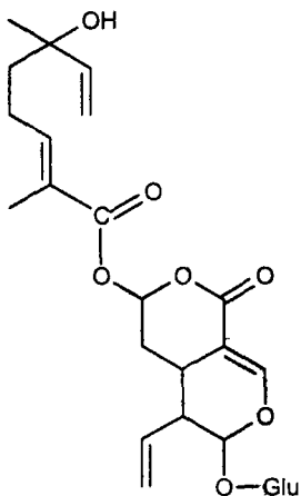
Ментіафолін
