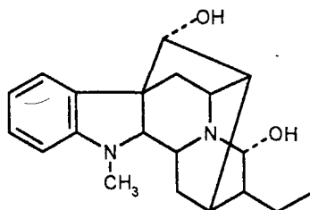
Аймалін
