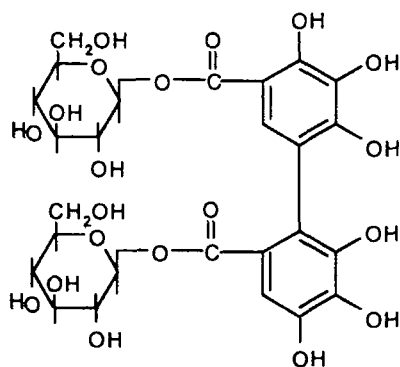
Альнітанін
