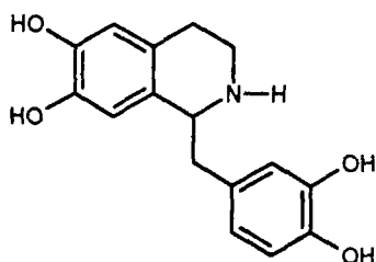
Норлауданозолін
