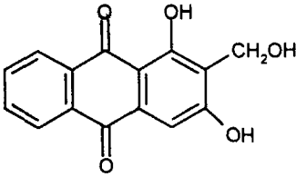
Луцидин
