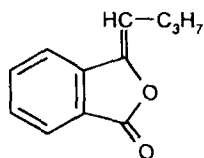
Кнідієвий лактон
