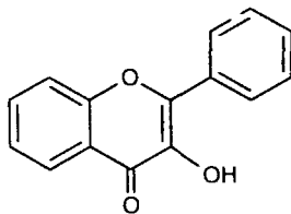
7 Флавоно́л
