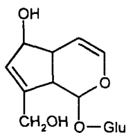
Аукубін
