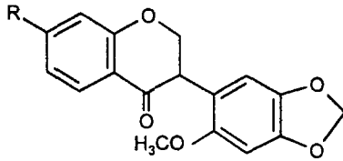
Оногенин (R=OH) Онозид (R=O—Glu)
