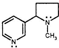
Нікотин
