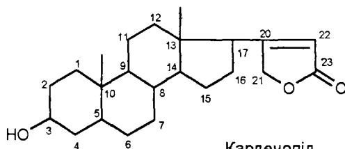
Карденолід
