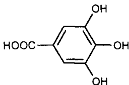
Галова кислота
