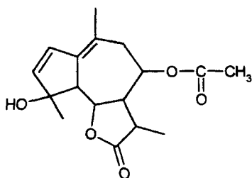
Матрицин
