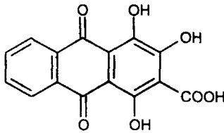
Пурпурин-3-карбонова кислота
