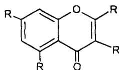
Хромони
