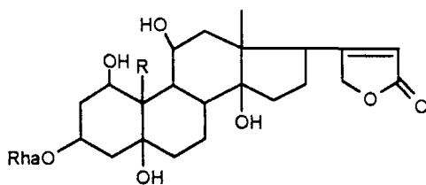
G-Строфантин
