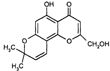
Птерохроманол
