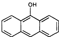
Антранол
