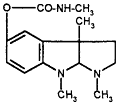
Фізостигмін
