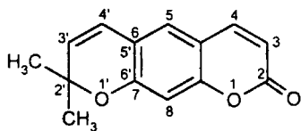
2',2'-Диметилксантилетин
