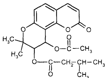
Дигідросамідин
