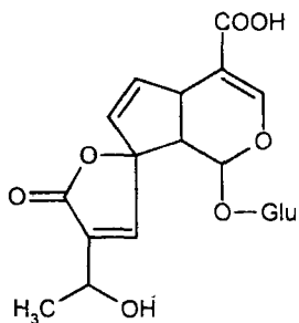
Плюмерид
