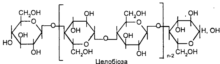
Будова целюлози
