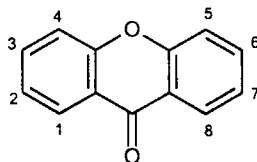
Ксантон (дибензо-γ-пірон)
