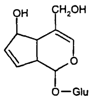
Декалозид
