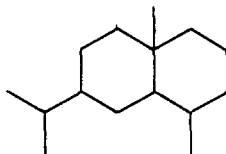
Евдесман
