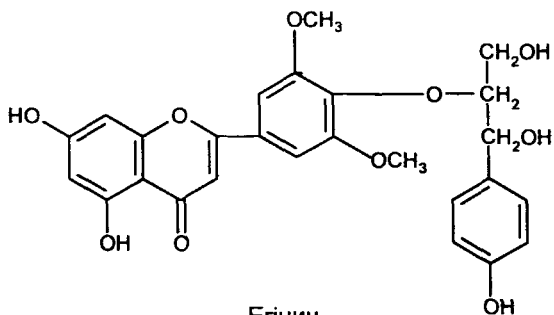
Егіцин
