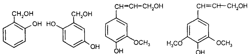
Саліциловий спирт
