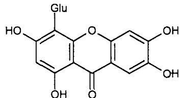
Ізомангіферин
