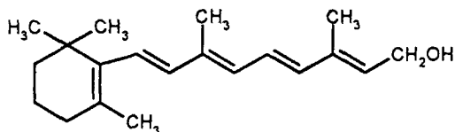
Вітамін А
