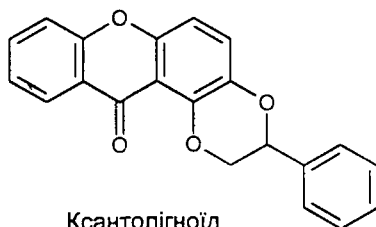
Ксантолігноїд
