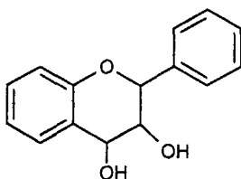
2. Флаван-3,4-діол (лейкоантоціанідин)
