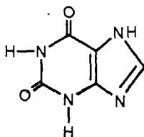
лактамна форма
