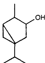
Туйол
