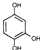
Гідроксигідрохінон
