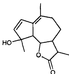
Артабсин
