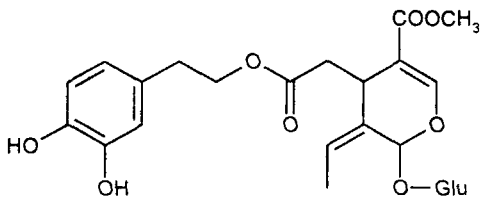
Олеуропеїн
