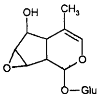
Деуціозид (менцелозид)
