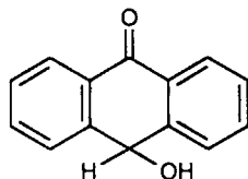
Оксиантрон
