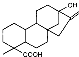
Стевіол
