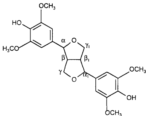
Сирінгорезиноп
