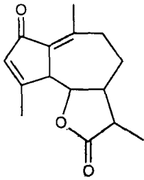
Ахілін
