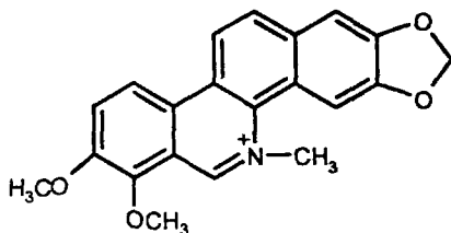
Хелеритрин
