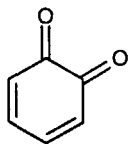
1,2-Бензохінон
