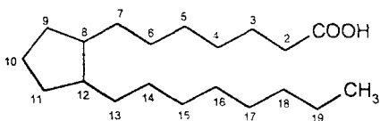
Простанова кислота
