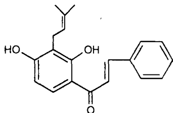
Ізокордоїн
