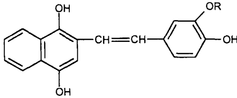
Піцеатанол
