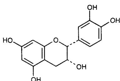
(-)-Епікатехін
