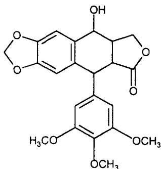
Подофілотоксин
