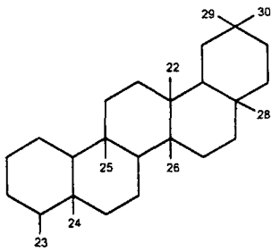
Фріделан
