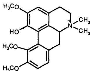
Магнофлорин
