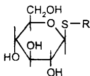
Тиоглікозид
