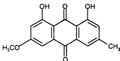
Фісціон
