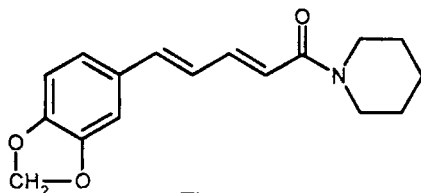
Піперин
