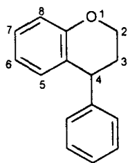
Неофлаван
