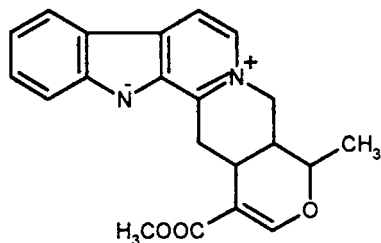
Серпентин
