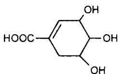
Шикімова кислота
