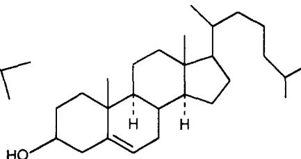
Холестерин
