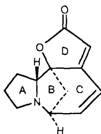
Норсекуринін
