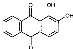
Алізарин
