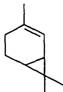
\Delta^4 -Карен
