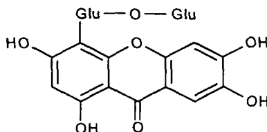
Глюкоізомангіферин
