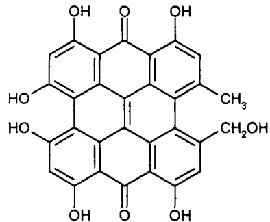
Псевдогіперіцин
