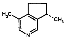
Актинідин
