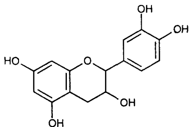
(+)-Епікатехін
