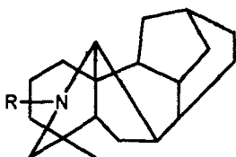
Аконітини
