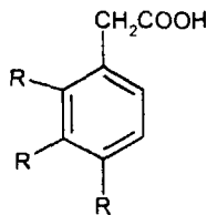
Фенілоцтові кислоти
