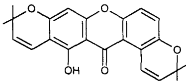
Товолтезин
