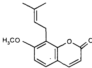
Остол
