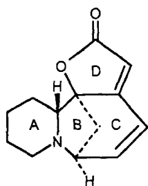
Секуринін
