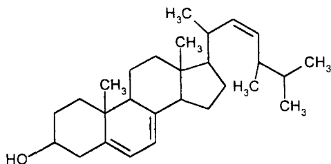
Ергостерин
