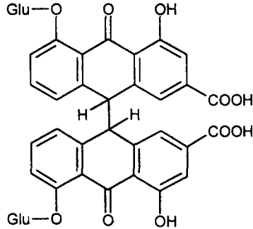
Сенозиди А і В
