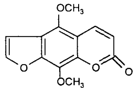
Ізопімпінілін
