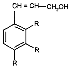
Гідроксикоричні спирти
