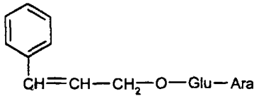
Розавін
