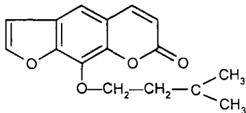
Імператорин
