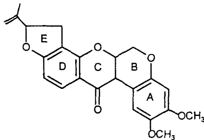
Ротенон, або хроmanoхроманон
