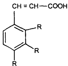
Гідроксикоричні кислоти
