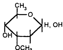
D-Цимароза
