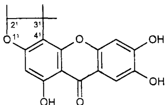
Ангулярний фураноксантон з Allanblackia floribunda
