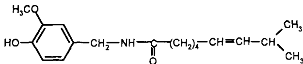
Капсаїцин
