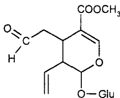
Секологанін
