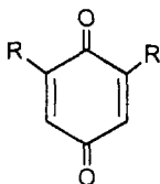
Бензохінони
