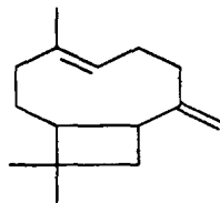
Каріофілен
