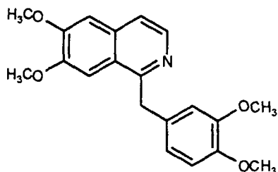
Папаверин
