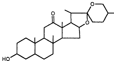
Гекогенін
