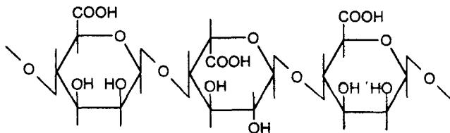
Альгінова кислота
