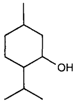
Ментол
