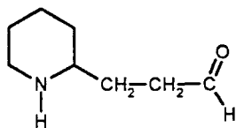
Пелетьєрин
