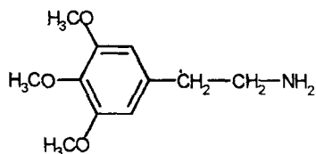
Мескалін
