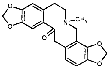
Протопін
