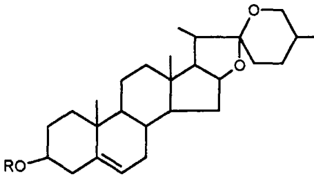
Діосгенін
