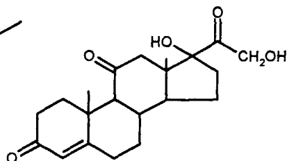
Кортизон
