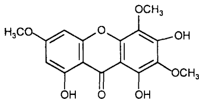
1,6,8-тригідрокси-3,5,7-триметоксикантон
