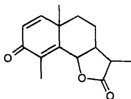
α-Сантонін
