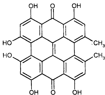
Гіперіцин
