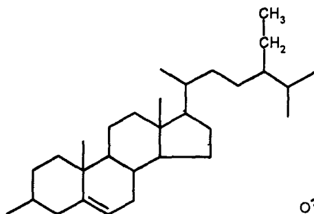
\beta -Сітостерол
