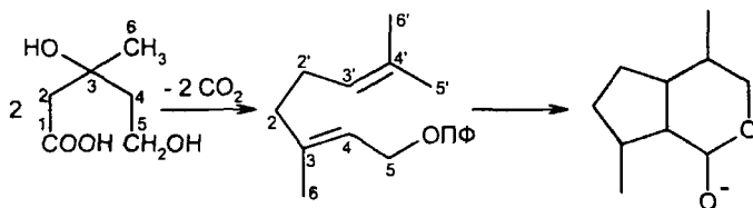
Мевалонова кислота
