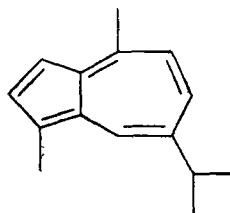
Гвайазулен
