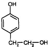
Тирозол
