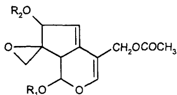
Валтрат
