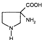
Кукурбітин
