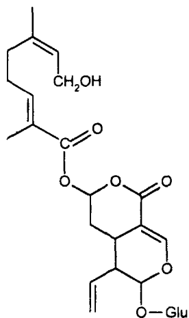
Фоліаментин
