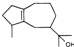
Гвайол
