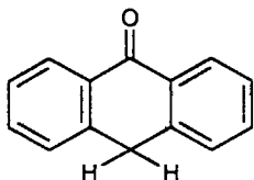
Антрон
