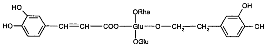
Ехінакозид
