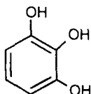
Пірогалол
