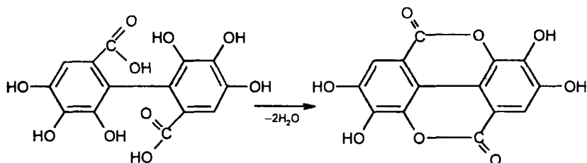
Гексаоксидифенова кислота
