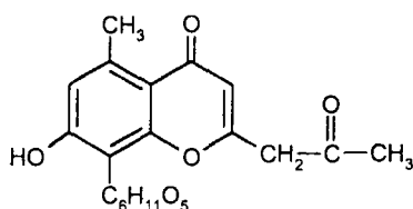
Алоезин
