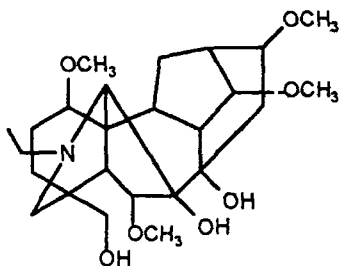
Лікоктонін
