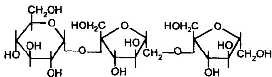
6-Кестоза
