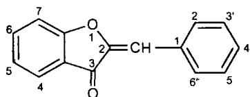
8 Аурон
