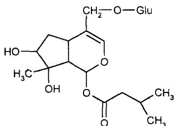
Валерозидат
