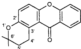
Ангулярний піраноксантон
