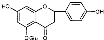
Саліпурпозид
