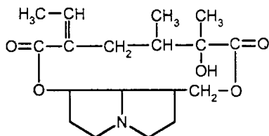
Платифілін
