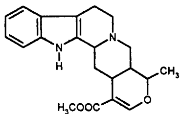
Аймаліцин
