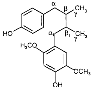
Дигідрогваяретова кислота
