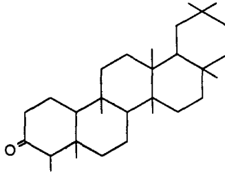
Фіделін
