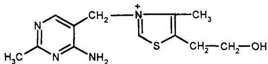
Тіамін
