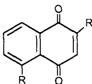
Нафтохінони
