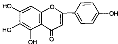
Скутелеяреїн (5,6,7,4'-тетраоксифлаво́н)
