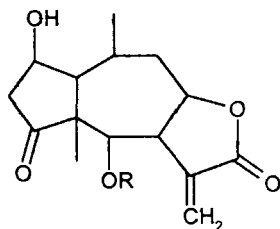
Арніфолін
