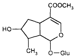
Логанін
