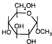
Метил- \alpha - D -глюкопіранозид
