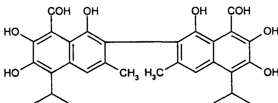
Госипол
