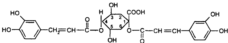
Цинарин
