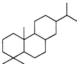
Тип абістану
