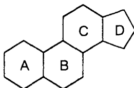
Стеран
