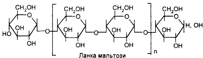
Будова амілози
