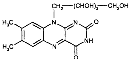
Рибофлавін
