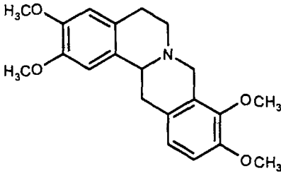
Гіндарин
