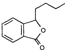
3-Бутилфталід
