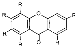
Ксантони
