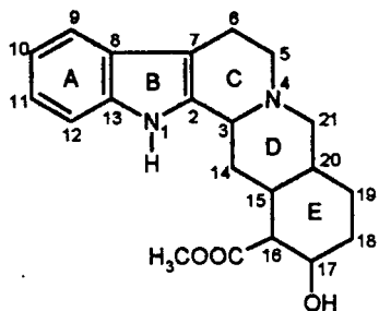
Йохімбін
