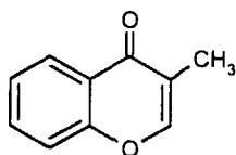
3-Метилхромон
