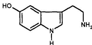
Серотонін
