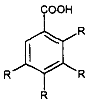
Фенольні кислоти
