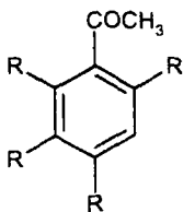
Ацетофенони
