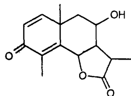
Артемізин
