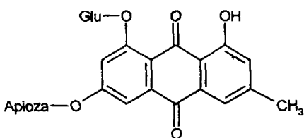
Глюкофрангулін Б
