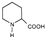
Кислота піперколінова
