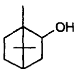
Борнеол
