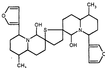
Нуфлеїн (тіобінуфаридин)
