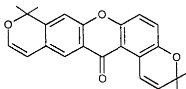
Дипіраноксантон
