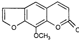
Ксантотоксин
