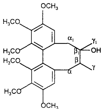
Діарілоктановий тип
