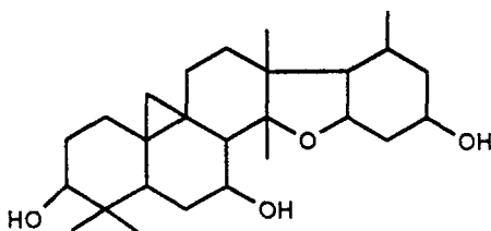
Дазіантогенін
