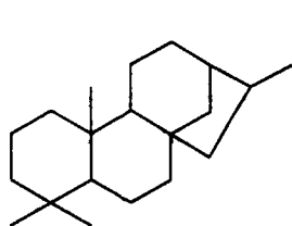
Тип каурану
