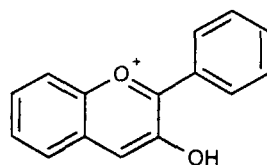
3 Антоціанідин
