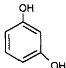
Резорцин
