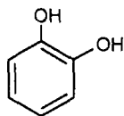
Пірокатехін
