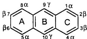
Антрацен
