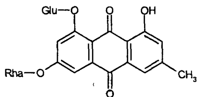
Глюкофрангулін А
