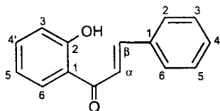
9. Халкон
