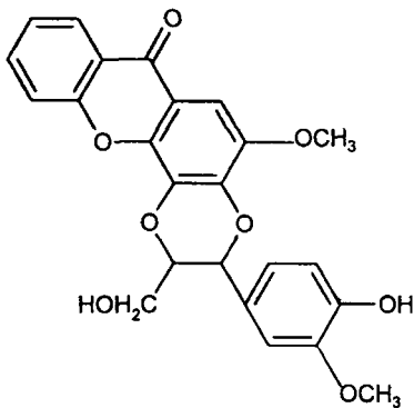
Кількорин
