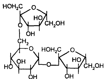
Неокестоза
