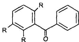
Бензофенони
