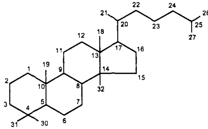
Ланостан
