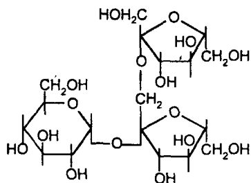
1-Кестоза (ізокестоза)
