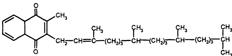
Вітамін K 1
