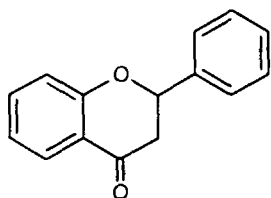
4 Флаванон
