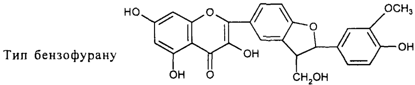
Силікрістин
