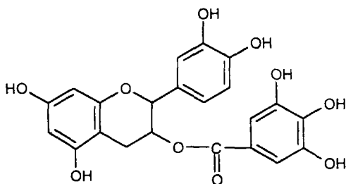
Катехілгалат
