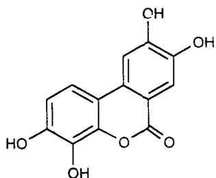
Гідроксильне похідне 3,4-бензокумарину
