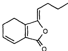
Лігустилід
