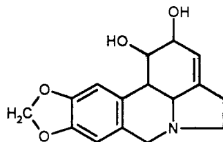
Лікорин
