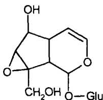
Каталпол
