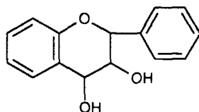
Флаван-3,4-діол
