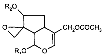
Дигідровалтрат
