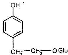
Салідрозид
