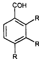
Фенольні альдегіди
