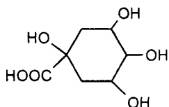
Хінна кислота
