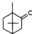
(-)-Камфора
