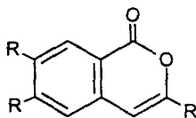
Ізокумарини
