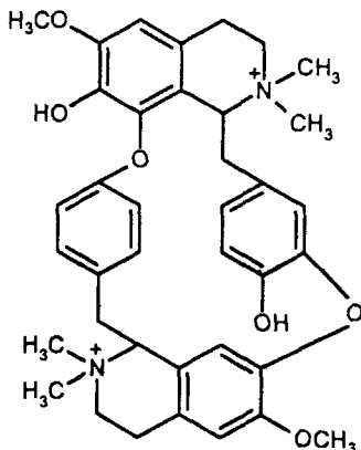
d-Тубокурарин
