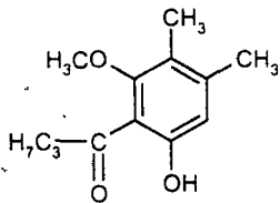
Аспідинол
