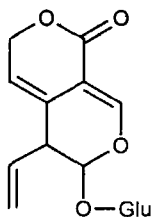
Генціопікрозид (генціопікрин)
