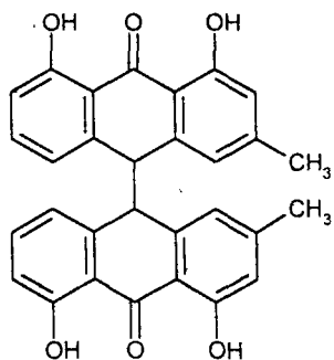
Хризофанолдіантрон
