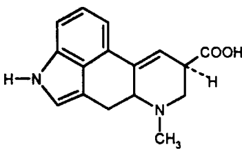
D-Лізергінова кислота
