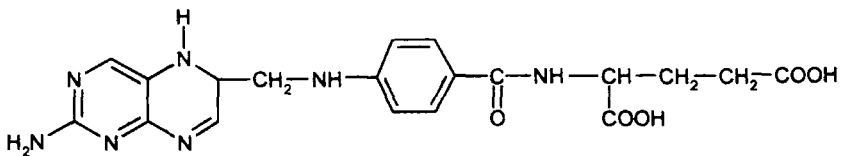
Фолієва кислота
