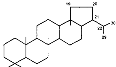
Гопан
