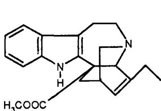
Катарантин
