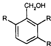
Фенольні спирти
