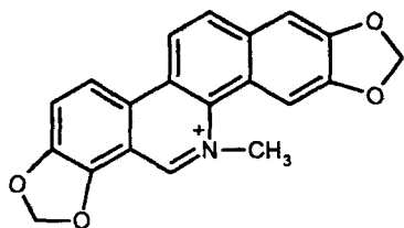
Сангвінарин
