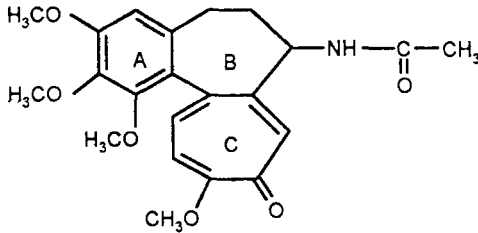
Колхіцин
