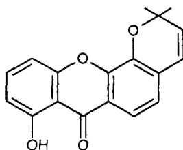
1-окси-5,6:2',3'-пірано-6''-диметилксантон з Calophyllum brasiliense
