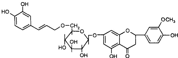
Гнафалозид А
