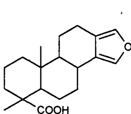
Ламбертинова кислота
