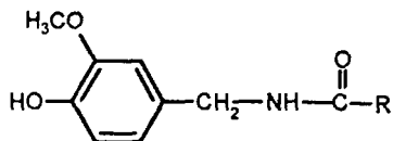
Капсаїциноїди
