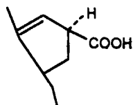
D-Ізолізергінова кислота
