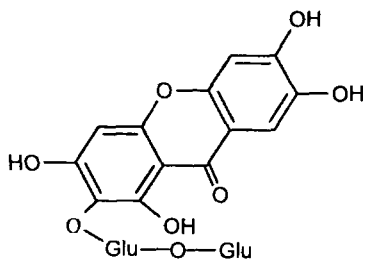
Глюкомангіферин
