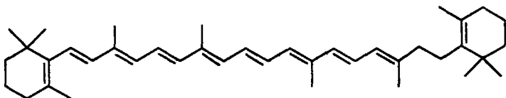
\beta -Каротин
