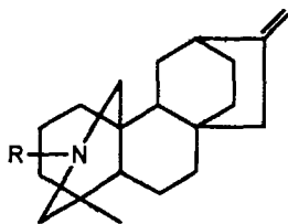
Атизини
