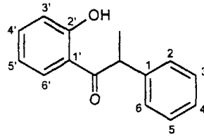
Ізодигідрохалкон
