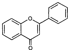
6. Флаво́н
