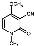
Рицинін
