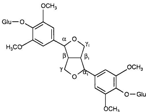
Елеутерозид Е
