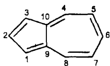
Азулен
