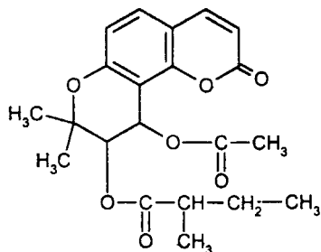
Віснадін
