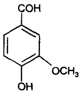
Ванілін
