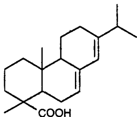
Абіетинова кислота
