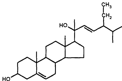
Стігмастерол
