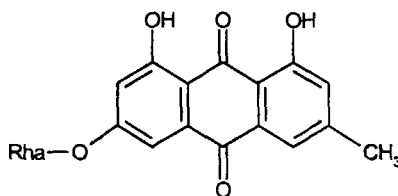
Франгулін А
