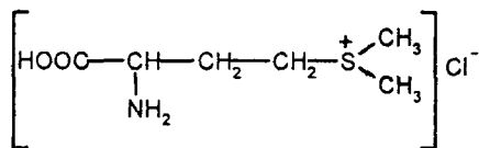
Метилметіонінсульфоній хлорид
