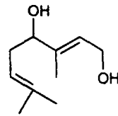
Розирідол
