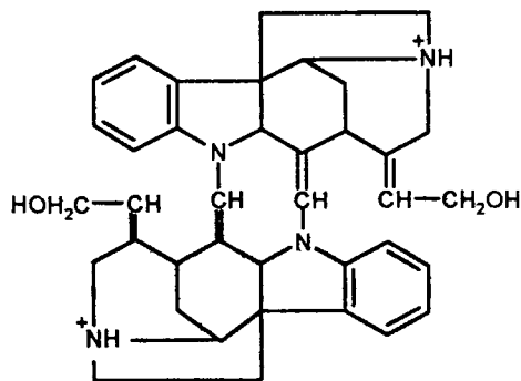
Токсиферин С
