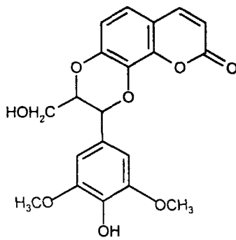
Дафнетичин
