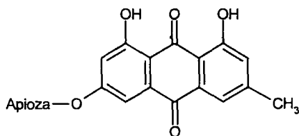
Франгулін Б
