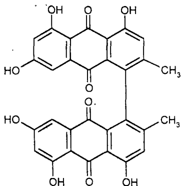
Касіанін
