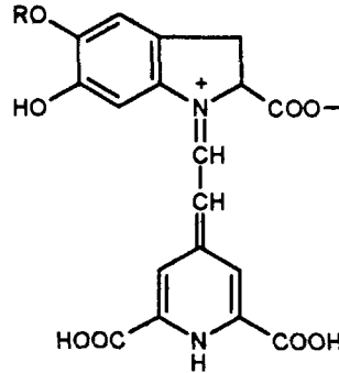
Бетанін R=цукор
