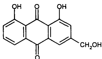
Алое-емодин
