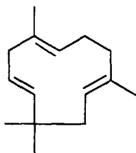
Гумулен
