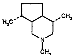
Скитанін
