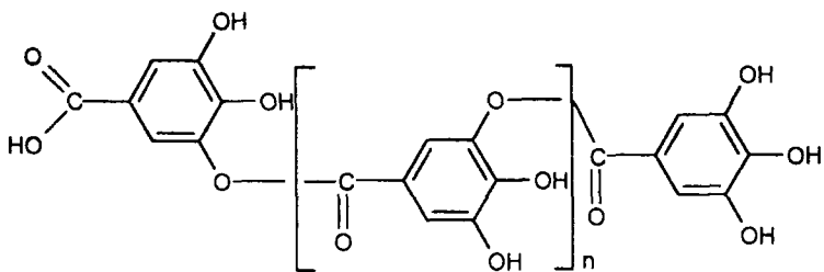
Полігалова кислота
