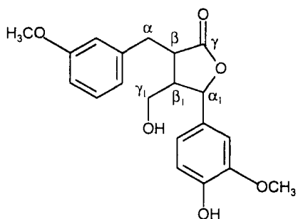
Ларицирезиноп
