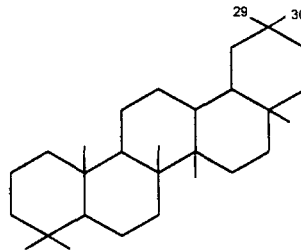
Олеанан
