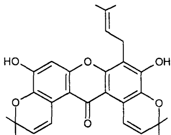
Товофелін
