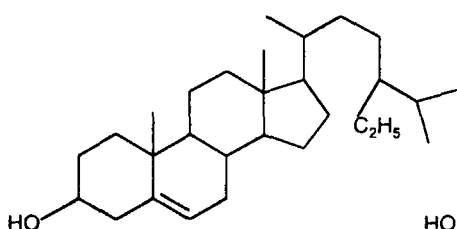
Ситостерин
