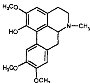
Глауцин
