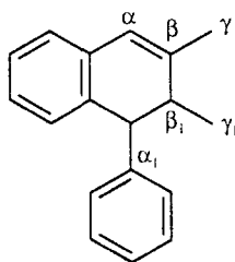
Дигідр.нафталіновий тип
