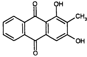
Рубіадин
