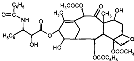
Паклітаксел (таксол)
