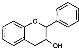
1 Флаван-3-ол (катехин)
