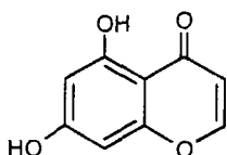
5,7-Дигідроксихромон
