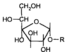
\alpha -Глюкофуранозид
