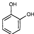
Пірокатехін
