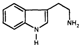
Триптамін
