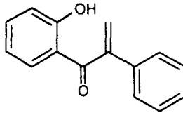
Ізохалкон
