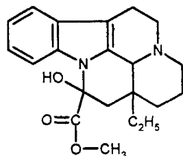
Вінкамін
