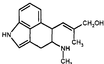
Ханоклавін
