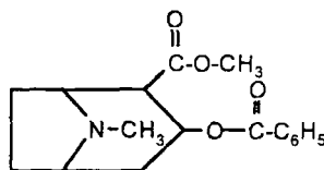
Кокаїн
