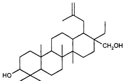
Арнідіол
