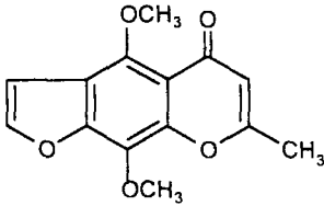
Келін
