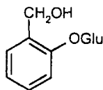
Саліцин
