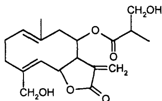
Аркціопікрин
