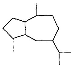
Гвайан
