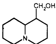
Нор-пупінан
