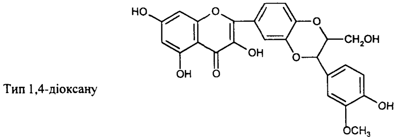
Силібін
