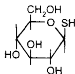
Тиоглюкоза
