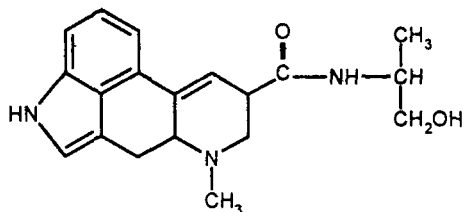
Ергометрин
