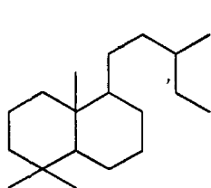
Тип лабдану
