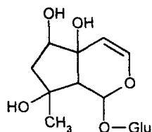
Гарпагід
