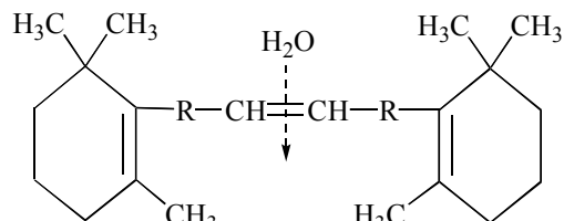
\beta -Каротин
