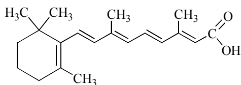
Транс-ретиноєва кислота
