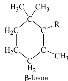
\beta -Іонон
