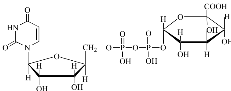
Уридиндифосфоглюкуронова кислота
