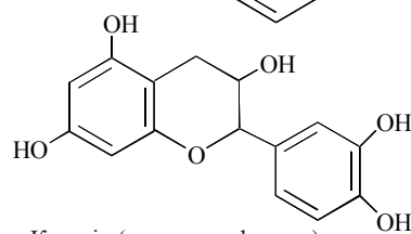
Катехін (пентаоксифлаван)
