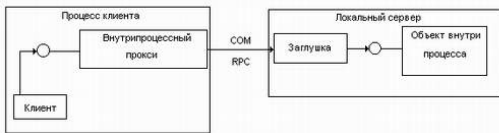
Рисунок 13.4 - Схема взаимодействия клиента с сервером в разных процессах на одном компьютере
