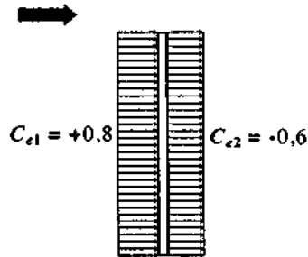
Схема 2. Будівлі с двосхилими покриттями
