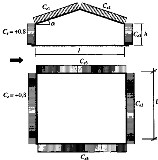
Схема 2. Будівлі с двосхилими покриттями
