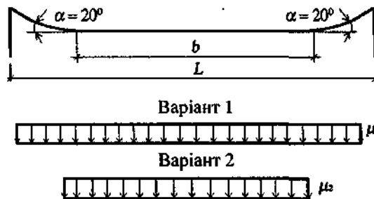
Схема 12. Висячі покриття циліндричної форми
