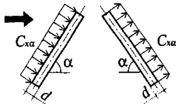
Схема 19. Ванти та нахилені трубчасті елементи, розташовані у площині потоку
