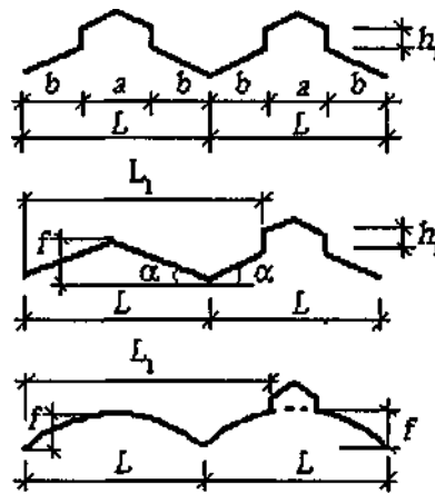
Схема 7. Дво- і багатопролітні будівлі з двосхилими і склепінчастими покриттями з поздовжнім ліхтарем
