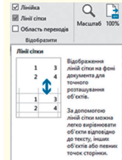
Рис. 3. Вкладка Лінії
