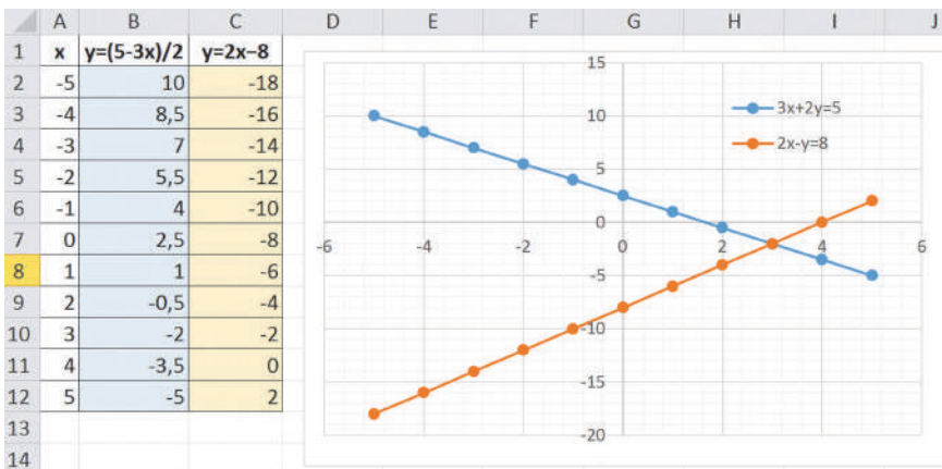
Рис. 1. Приклад графічного розв'язання системи лінійних рівнянь
