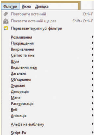
Рис. 1. Фільтри GIMP
