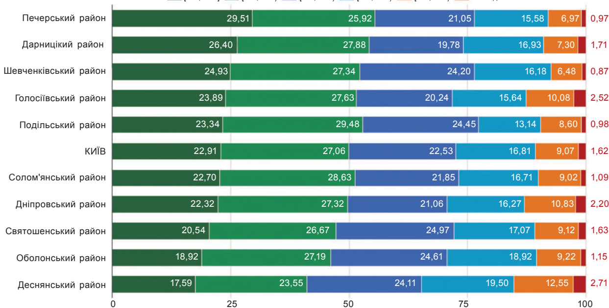
Рис. 4. Гістограма статистичного аналізу результатів ЗНО в місті Києві
