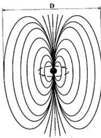
Рисунок. Очень условная графическая модель соотношения между первичным точечным вихрем и генерируемым им вихревым полем. Величина D стремится к бесконечности
