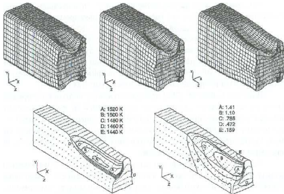
Рисунок 6.2 – Результати моделювання процесу сортової прокатки
