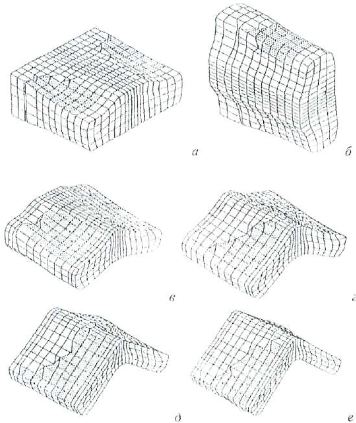
Рисунок 6.1 – Приклад результатів моделювання прокатки кутового профілю за допомогою системи CORM1L
