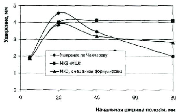
Рисунок 6.3 – Залежність розширення від ширини штаби, умови прокатки: A_0 = 10 мм; H_0 = 6 мм; R = 100 мм; \tau = 0,8
