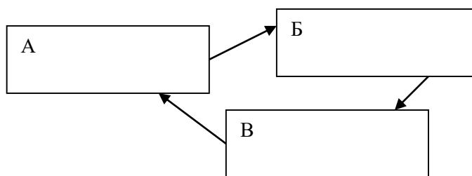
Рисунок 2.3 – Схема документообігу.....
