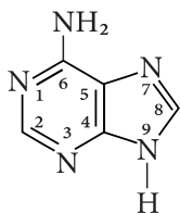
аденін (А) 6-амінопурін
