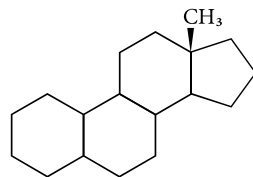
естран
