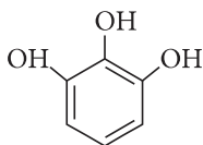
Пірогалол
