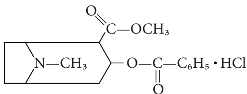
Кокаїну гідрохлорид
