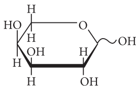
L -арабінопіраноза
