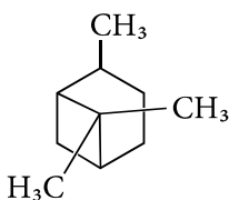
пінан
