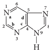
пурін
