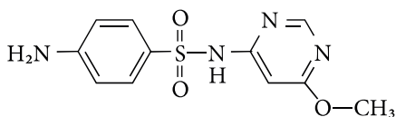
сульфамометоксин
