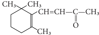
\beta -іонон
