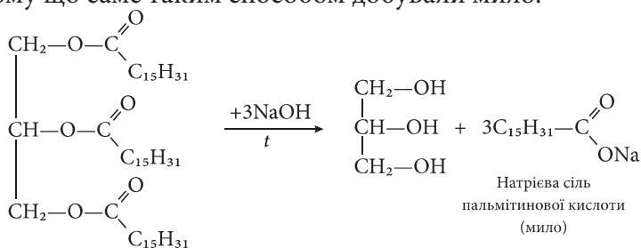
Трипальмітат гліцеролу
