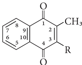
2-Метил-1,4-нафтохінон
