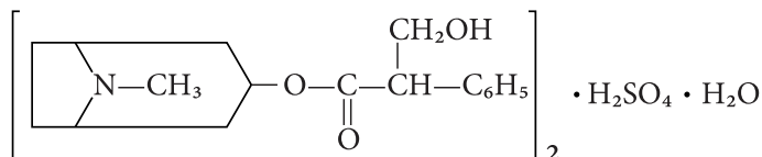
Атропіну сульфат
