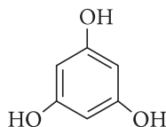
Флороглуцин
