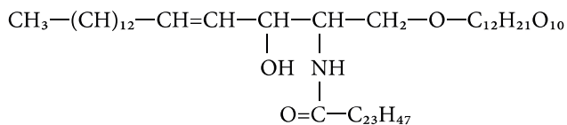
глобозидт (лактозилцерамід)
