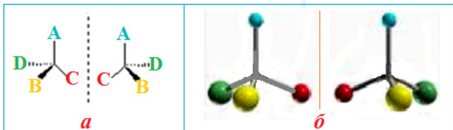
Рисунок 1.3 — Дзеркальні зображення sp^3 -гібридизованого асиметричного (хірального) атома Карбону з чотирма різними замісниками А, В, С і D: а) графічна формула; б) кульково-стрижнева модель
