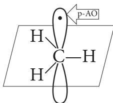
метил-радикал
