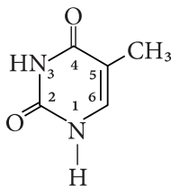
тимін (Т) 5-метилурацил 5-метил-2,4-діоксопіримідин
