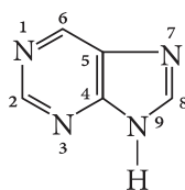
пурін
