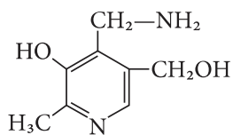
піридоксамін
