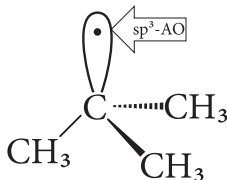
трет -бутил-радикал
