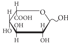
L -ідуоронова кислота
