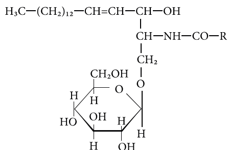
глюкоцереброзид
