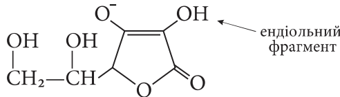
аскорбат-іон
