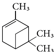
\alpha -пінен
