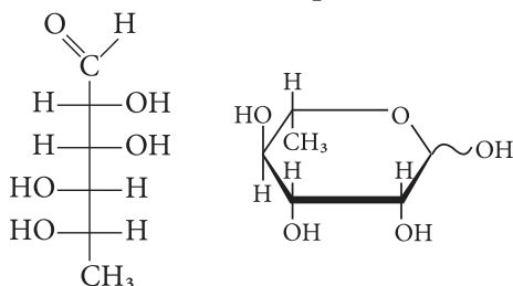
L -рамноза
