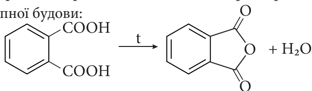
фталева кислота
