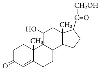
кортикостерон
