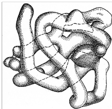
Третинна структура молекули білка міоглобіну
