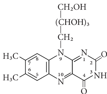
Рибофлавін
