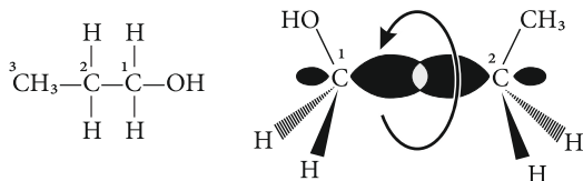
1-Пропанол. Обертання навколо \sigma -зв'язку
