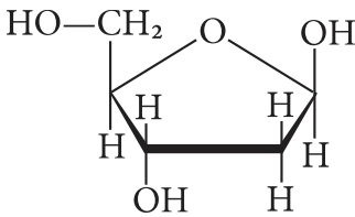
\beta -D-дезоксирибофураноза
