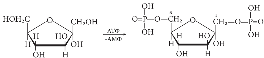
1,6-дифосфат- \alpha -D-фруктофураноза
