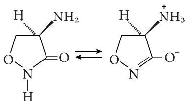
циклосерин (D-4-аміно-3-ізооксазолідинон)
