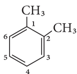
1,2-диметилбензен (орто-ксилол)
