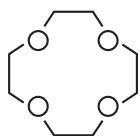
12-краун-4
