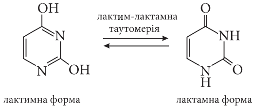
Урацил (2,4-дигідроксипіримідин)
