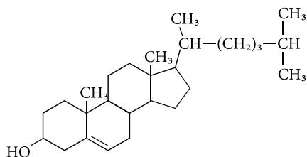
холестерин
