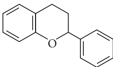
Флаван
