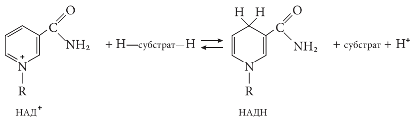
нікотинамід (вітамін РР)
