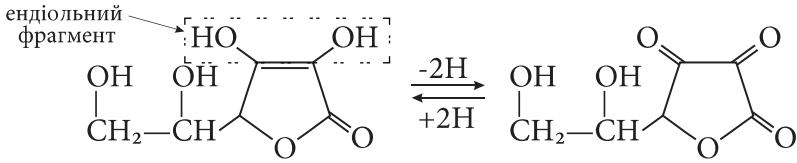
аскорбінова кислота
