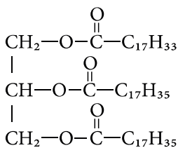
олеодистеарин
