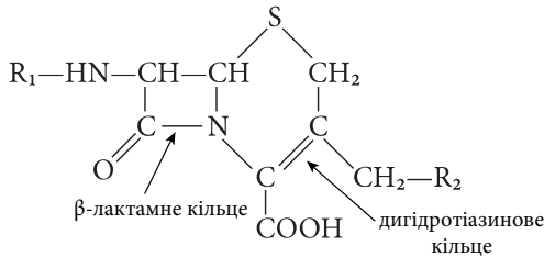
Загальна формула цефалоспоринів
