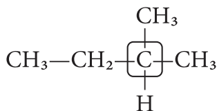
диметилетилметан
