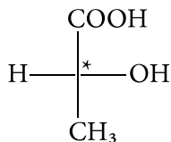
D(-)-молочна кислота
