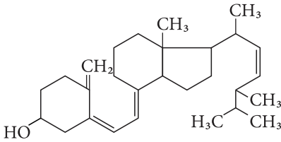
Вітамін D 2 (ергокальциферол)
