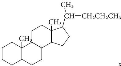
холан
