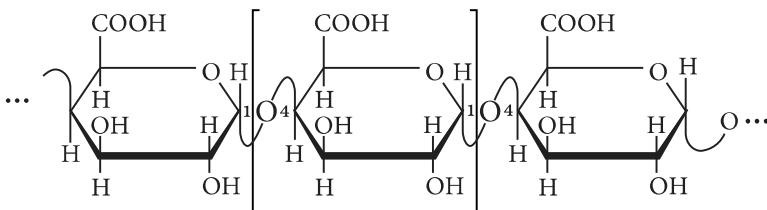
Фрагмент молекули пектової кислоти α-1,4-глікозидний зв'язок
