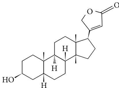
дигітоксигенін
