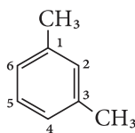
1,3-диметилбензен (мета-ксилол)
