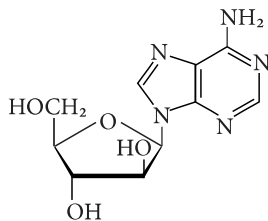
9-β-D-арабінофуранозиладенін
