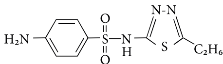
етазол
