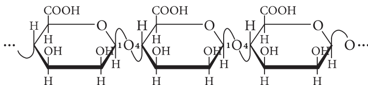
Фрагмент молекули альгінової кислоти β-1,4-глікозидний зв'язок
