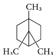
камфан
