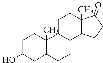
андростерон
