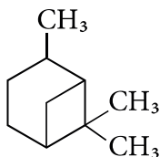
пінан
