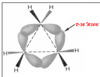
Утворення \tau -зв'язків в молекулі циклопропану
