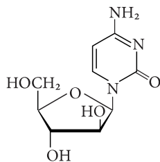
1-β-D-арабінофуранозилцитозин
