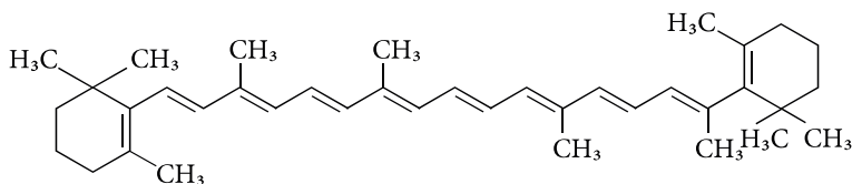
\beta - каротин
