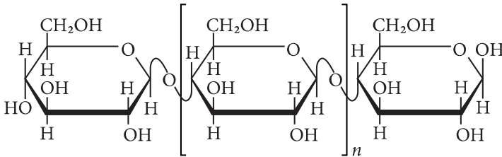
Целюлоза
