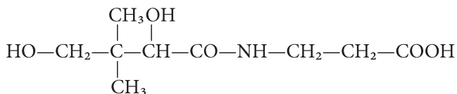
Пантенова кислота
