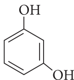
Резорцин 1,3-дигідроксибензен мета -ізомер
