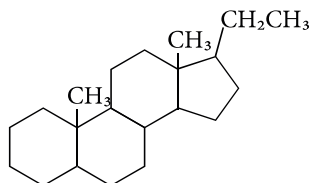
прегнан
