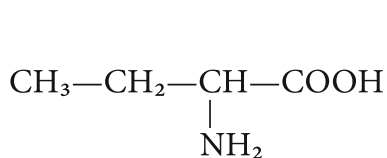
2-амінобутанова кислота
