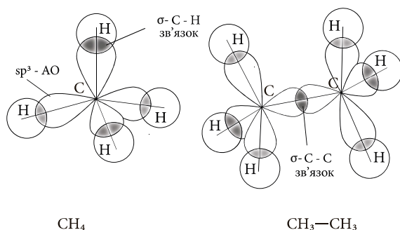
Рис. 3.1. Орбітальна будова метану та етану.
