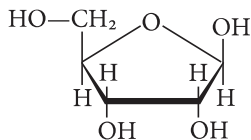
\beta - D -рибофураноза
