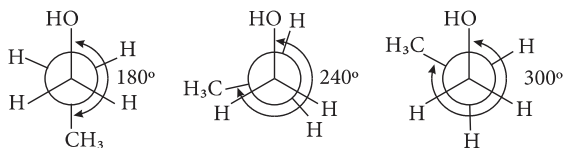
IV. Загальмована (анти)
