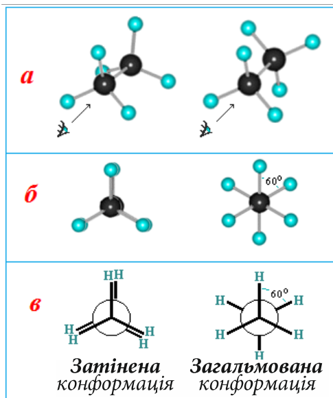
Рис. 1.2 — Конформації молекули етану: а) кульково-стрижнева модель; б) вигляд вздовж зв'язку C–C; в) проекційні формули Ньюмена.
