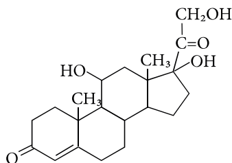
гідрокортизон
