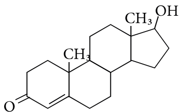
тестостерон
