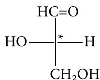
L- гліцероловий альдегід
