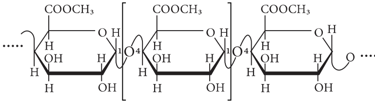
Фрагмент молекули пектинової кислоти α-1,4-глікозидний зв'язок
