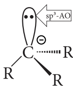
карбаніон
