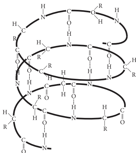
Вторинна структура молекули білка
