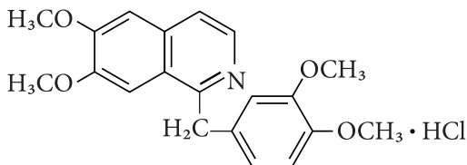
Папаверину гідрохлорид
