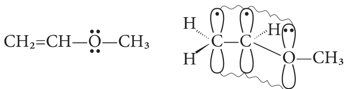
вінілметиловий етер
