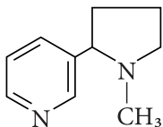
Нікотин
