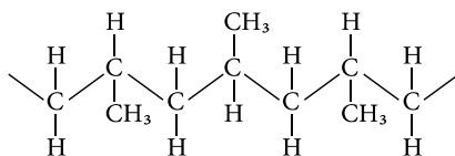
стереорегулярний синдіотактичний поліпропілен
