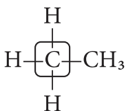
метилметан
