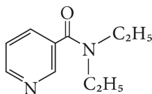
кордіамін
