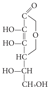
L-Аскорбінова кислота
