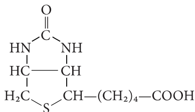
Біотин
