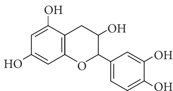
Катехін (пентаоксифлаван)
