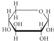
\alpha -D-ксилопіраноза (деревний цукор)
