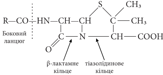
Загальна формула пеніцилінів
