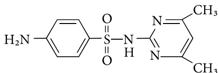
сульфадимезин
