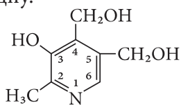
піридоксин (піридоксол)
