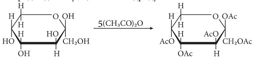
\beta -D-фруктопіраноза
