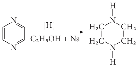
піразин
