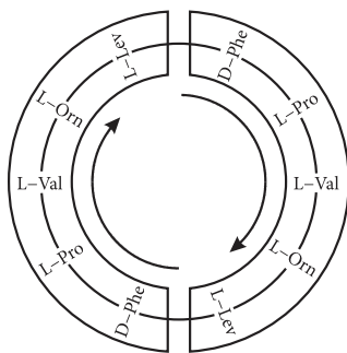
Граміцидин С
