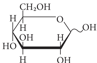
D -глюкопіраноза
