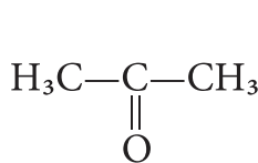
пропанон
