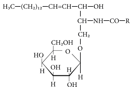
галактоцереброзид
