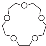
15-краун-5
