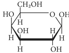
\beta -D-галактопіраноза
