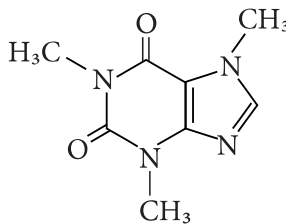
Кофеїн
