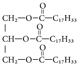
триолеїн
