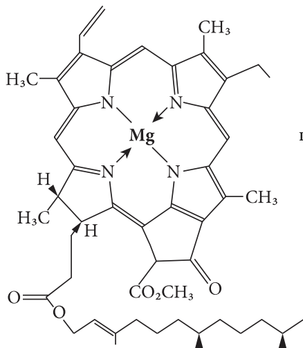
хлорофіл
