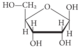
\beta -D-рибофураноза
