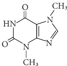
Теобромін
