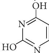
Лактимна форма
