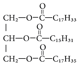
олеопальмітостеарин
