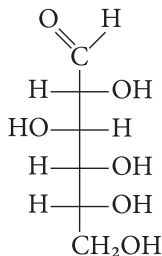
D -глюкоза
