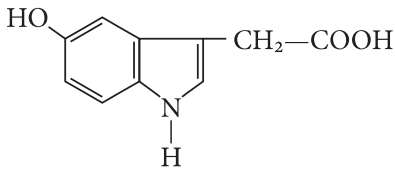
5-гідроксиокси- \beta -індолілоцтова кислота
