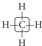
метан
