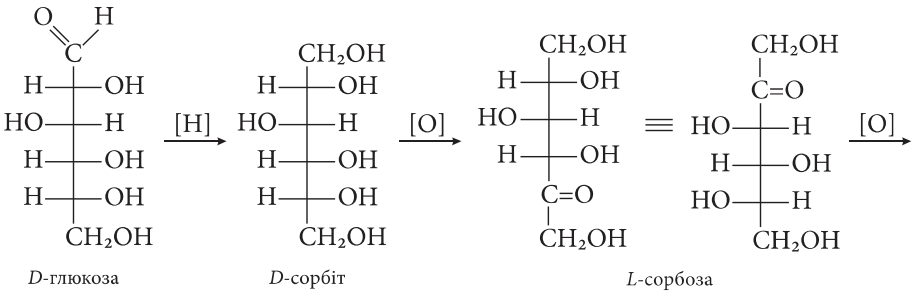
D -глюкоза
