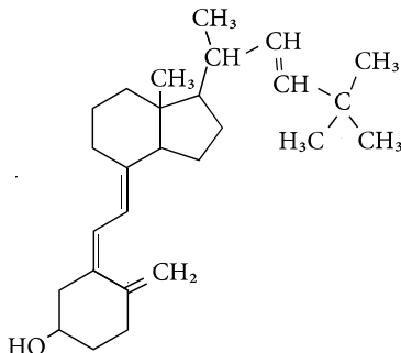
вітамін D_2
