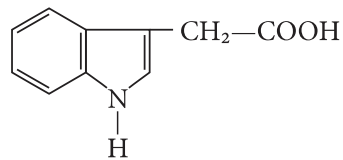
\beta -індолілоцтова кислота
