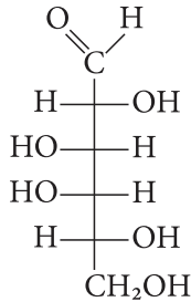
D-галактоза
