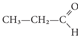
пропаналь
