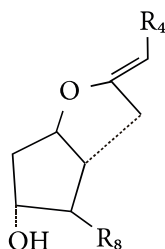
PGI
