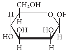
\beta -D-манопіраноза
