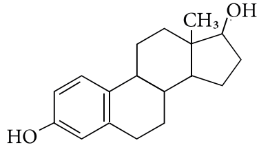
естрадіол
