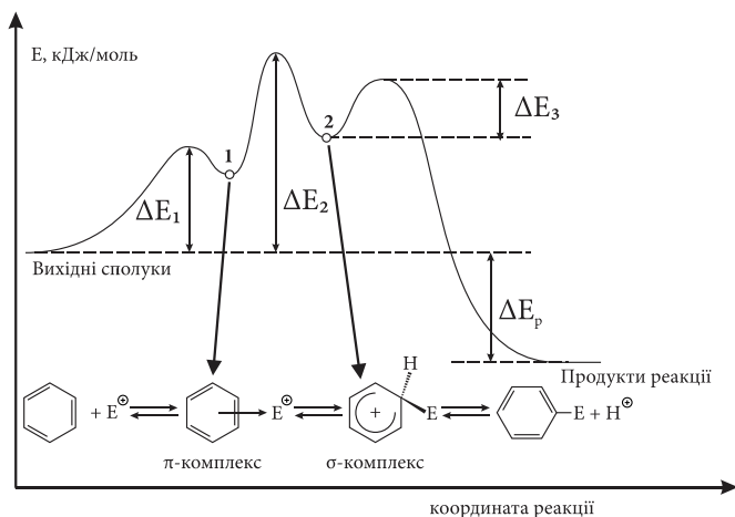
Енергетична діаграма реакції електрофільного заміщення
