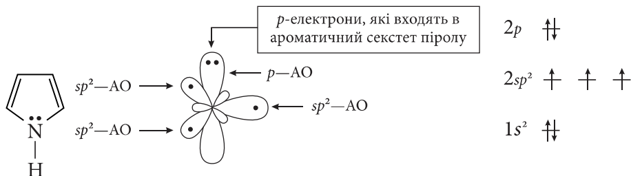
Розподіл електронів пірольного атома нітрогену по орбіталях
