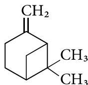
\beta -пінен
