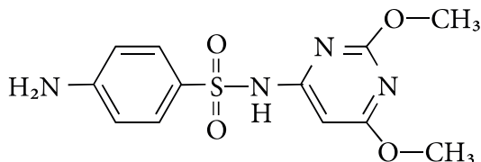
сульфадиметоксин
