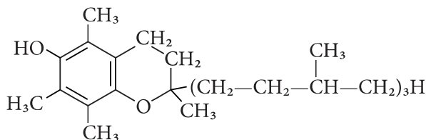
Вітамін Е (α-токоферол)
