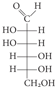
D-маноза
