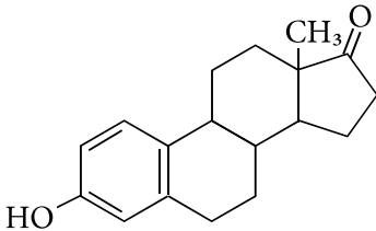
естрон
