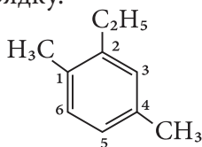
2-етил-1,4-диметилбензен
