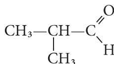
ізомасляний альдегід
