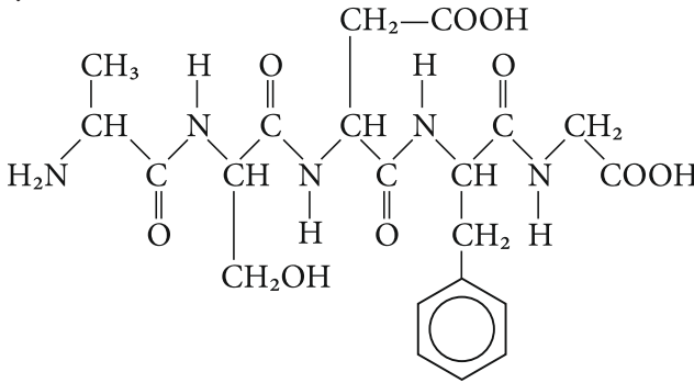
аланіл-серил-аспарагіл-фенілаланіл-гліцин Ala-Ser-Asp-Phe-Gly
