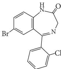
феназепам
