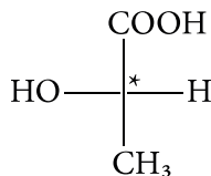
L(+)-молочна кислота
