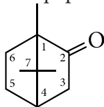
камфора
