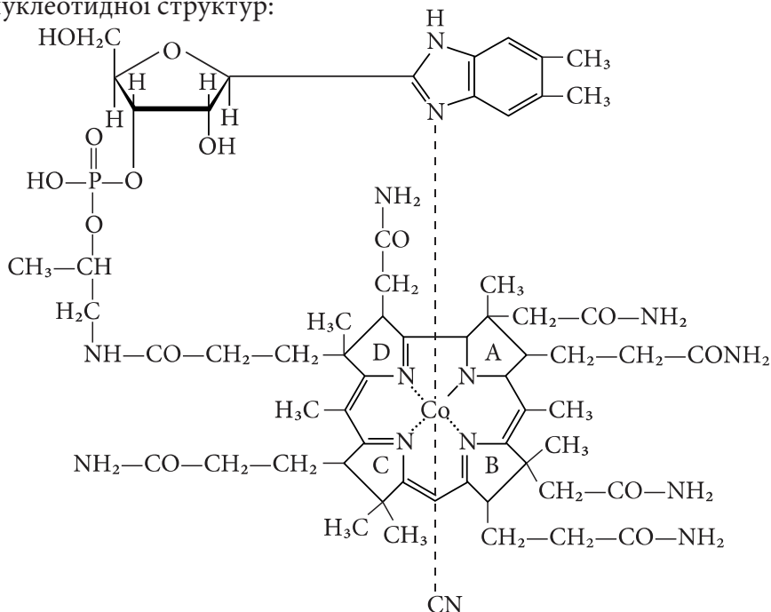
Вітамін В 12 (ціанкобаламін)
