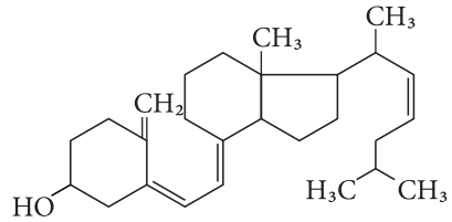
Вітамін D 3 (холекальциферол)
