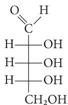
D -рибоза
