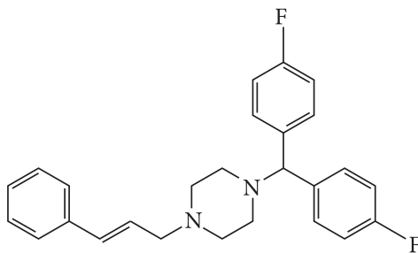
флунаризин
