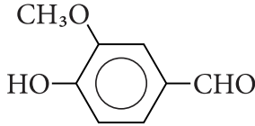
ванілін
