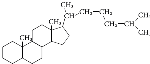
холестан
