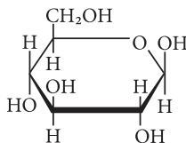
\beta - D -глюкопіраноза
