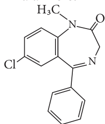
діазепам
