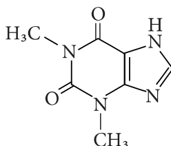
Теофілін
