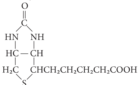
біотин
