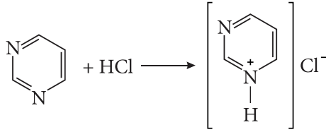
піримідиній хлорид
