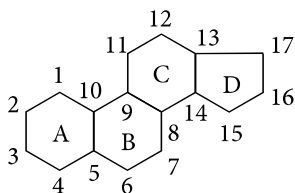
стеран
