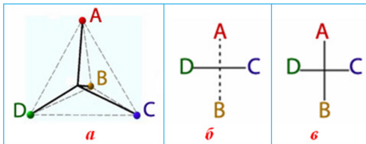
Рисунок 1.4 — Графічне зображення асиметричного атома C^* , сполученого з різними замісниками А, В, С і D: а) об'ємне зображення; б) формула Фішера, в якій пунктирною лінією показано розміщення верхнього А і нижнього В замісників за площиною креслення; в) звичайна формула Фішера
