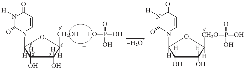
Уридин
