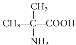
2-аміно-2-метилпропанова кислота
