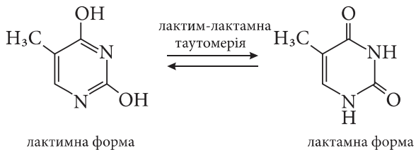
Тимін (2,4-дигідрокси-5-метилпіримідин)
