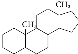
андростан
