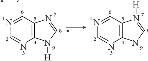
9H-пурин
