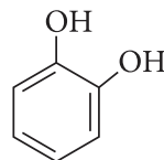
Пірокатехін 1,2-дигідроксибензен орто -ізомер
