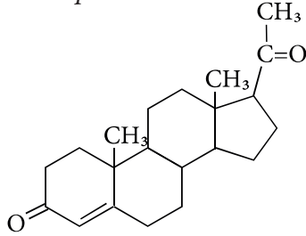
прогестерон
