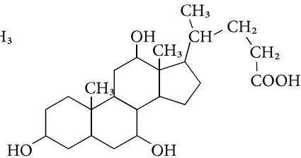
холева кислота
