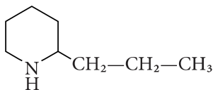
Коніїн
