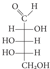
L -арабіноза
