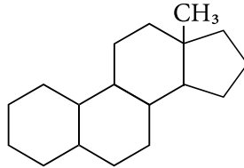
естран
