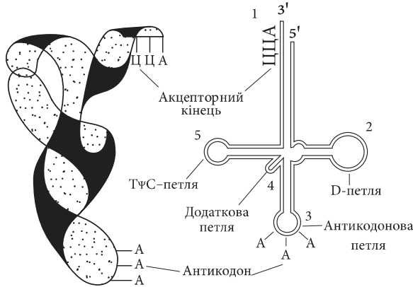
Вторинна (праворуч) та третинна (ліворуч) структури тРНК
