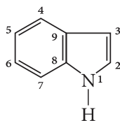
індол
