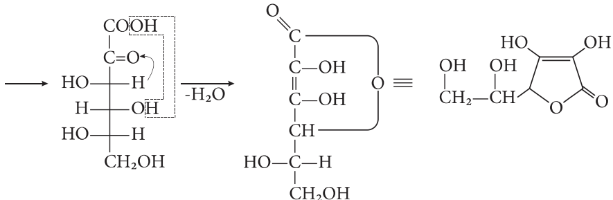
2-кето- L -гулонова кислота
