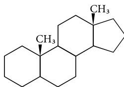
андростан
