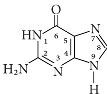
гуанін (Г) 2-аміно-6-оксопурін
