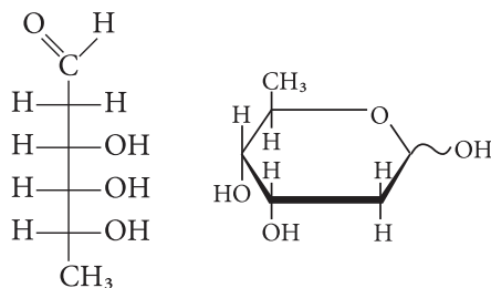
D -дигітоксоза
