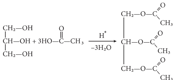
триацетат гліцеролу
