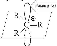
карбокатион
