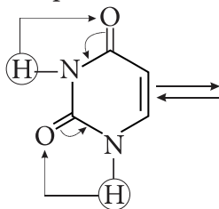
Лактамна форма
