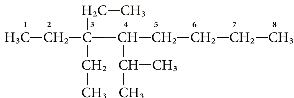
3,3-діетил-4-ізопропілоктан
