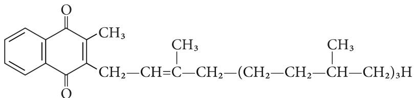
Вітамін К 1
