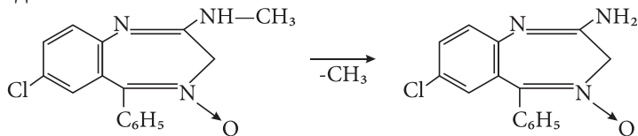
хлордіазепоксид
