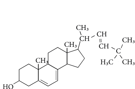
ергостерин
