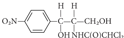
левоміцетин
