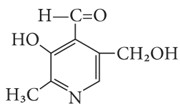
піридоксаль
