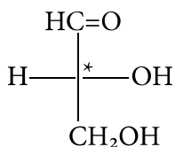
D- гліцероловий альдегід
