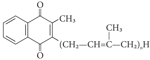
Вітамін К 2 (n=6;7;9)
