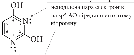
урацил (2,4-дигідроксипіримідин)
