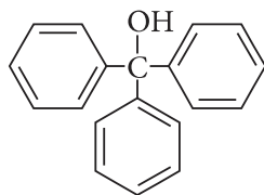
трифенілметанол
