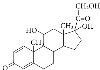
преднізолон
