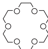
18-краун-6
