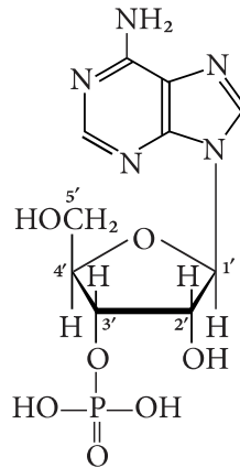
Аденозин-3'-монофосфат
