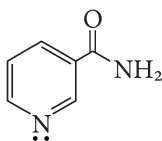
нікотинамід (вітамін РР)
