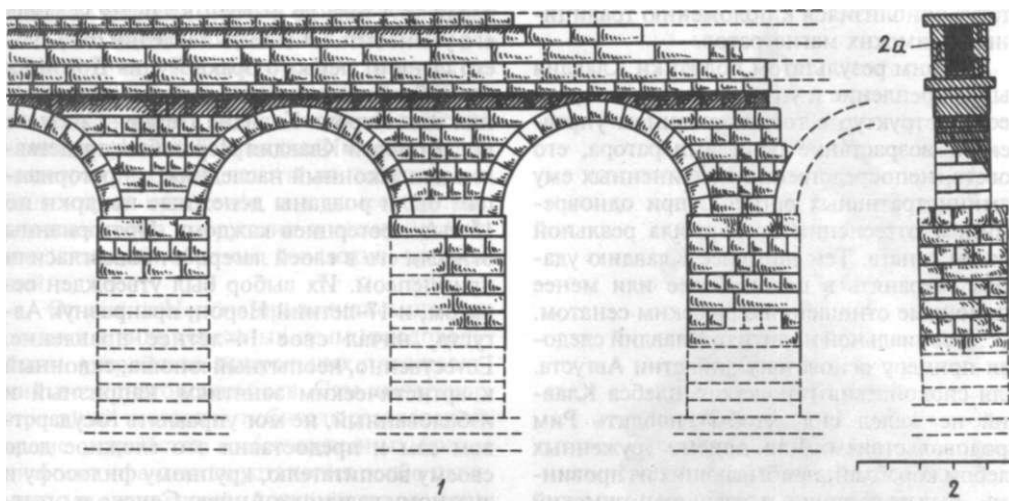
Римский акведук. I в. н. э.:
