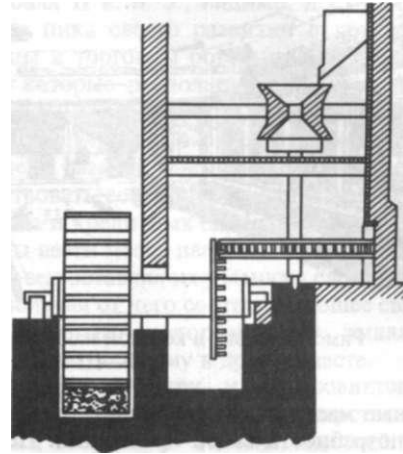
Водяная мельница. I в. н. э. Реконструкция по трактату Витрувия
