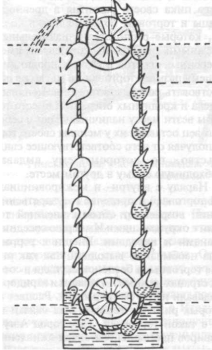
Механизм для подачи воды на более высокий уровень. Реконструкция. I в. н. э. Италия
