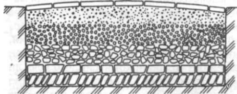
Схематическое изображение римской дороги. Разрез
