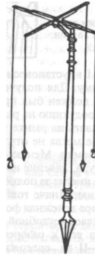
Римская грома — специальный землемерный инструмент. Реконструкция. I в. н. э.
