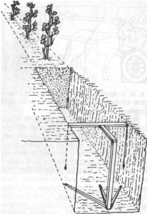
Глубокий плантаж для посадки виноградных лоз. Реконструкция. I в. н. э. Италия.
