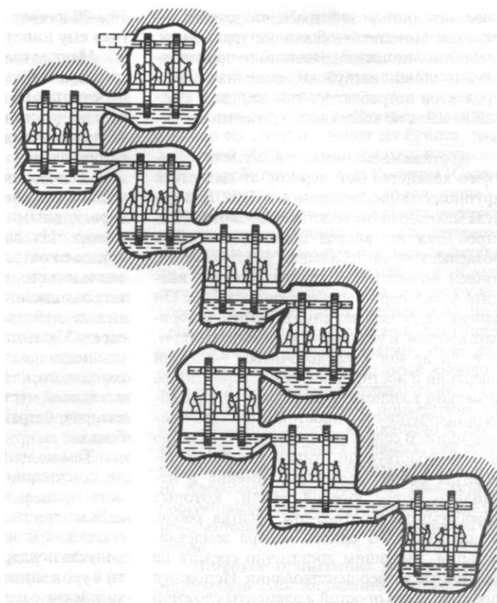
Механические приспособления для откачки воды из шахт. I в. до н. э. — II в. н. э. Реконструкция
