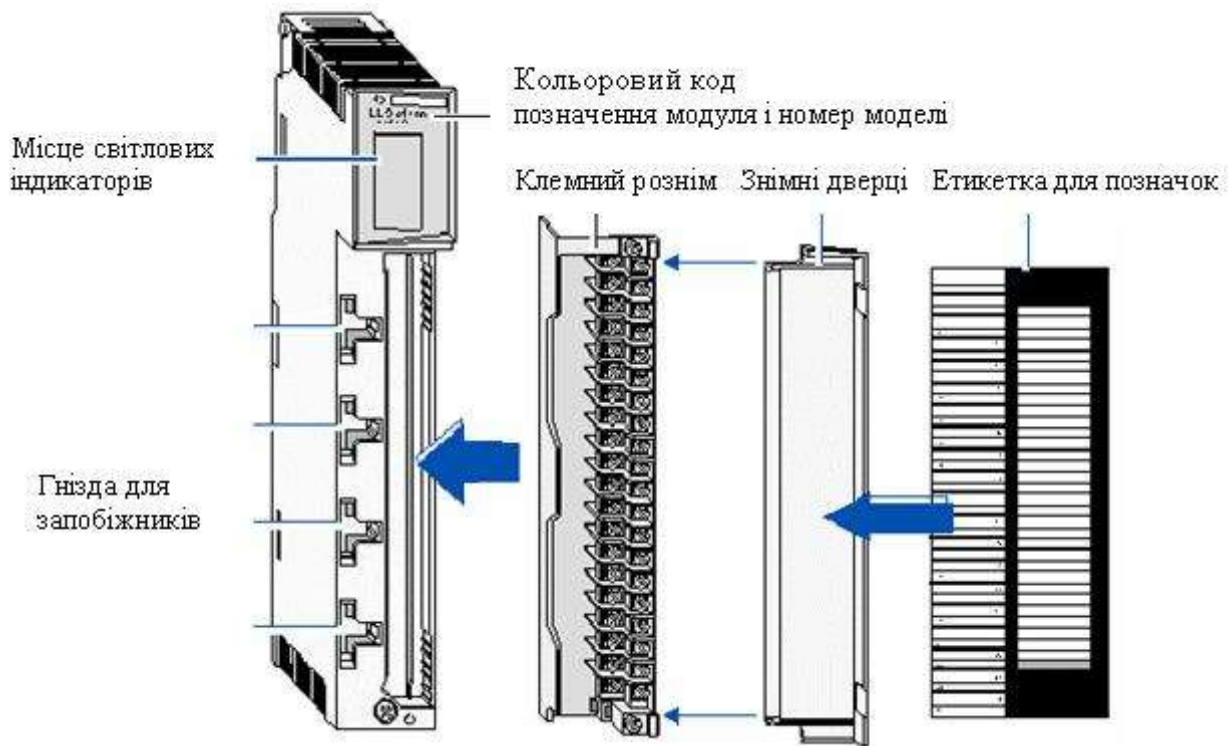
Рисунок 8.4 – Модуль вводу-виводу
