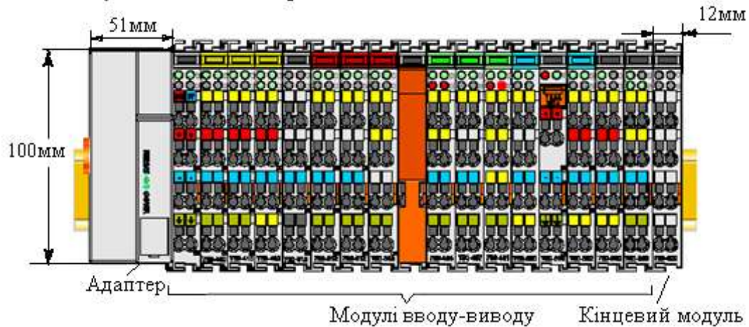
Рисунок 6.2 – Fieldbus вузол
