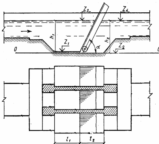
Рис.3.1 – Схема установки ґрат
