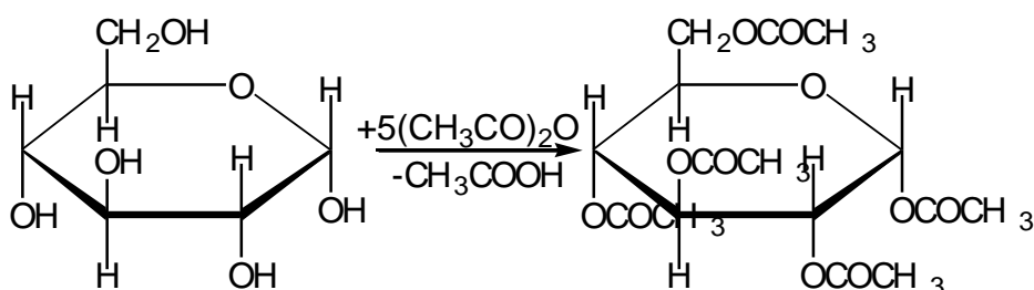
\alpha -Д-глюкопіраноза
