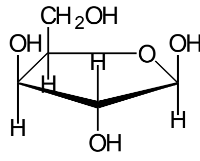
\beta -D-глюкофураноза
