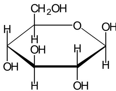
\beta -D-глюкопіраноза
