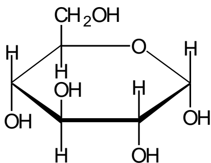
\alpha -D-глюкопіраноза
