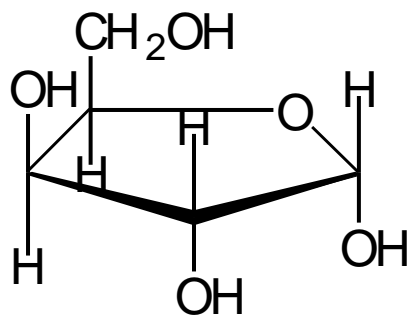
\alpha -D-глюкофураноза
