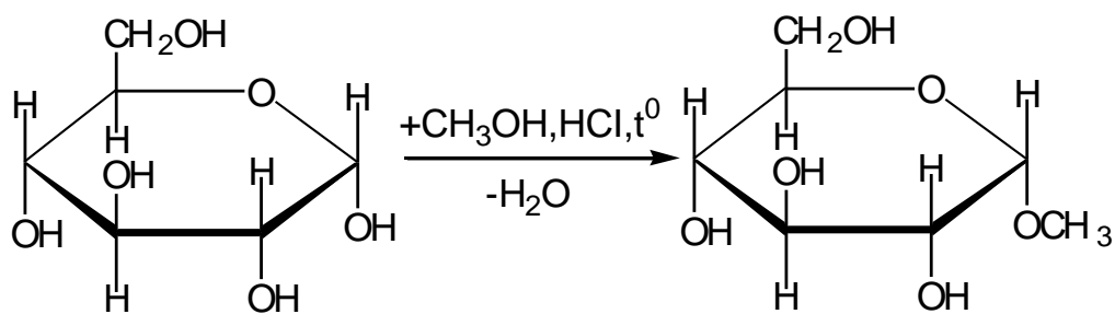
\alpha -Д-глюкопіраноза
