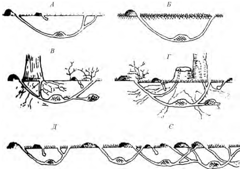
Рис. 5.5. Муридний тип норіння: A, Б, В, Г – муридний підтип, Д, Е – мікротинний підтип; A, Б – прості літні нори хатньої та лісової миші; В – осіння нора лісової миші; С – нора жовтогорлого мишака; Д, Е – поодинокі нори та колоніальні поселення рудої норці; ———— – нори у ґрунтовому горизонті, ———— – нори під корою та в середині стовбурів дерев і пенеків, ———— – викиди ґрунту (мишовини), ———— – гніздові камери, ———— – кормові камери (комори), ———— – тимчасові сховища.
