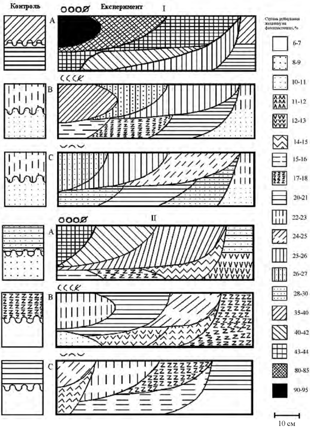
Рис. 5.2. Поширення зони впливу екскреції сарни на протеолітичну активність ґрунту: I – суглинний ґрунт у заплаві липово-ясеневій діброві; II – піщаний ґрунт у сухуватому борі на арені; A – через місяць, B – через 6 місяців, C – через 10 місяців; ○○○○, ◀▶▶▶, ~~~ – місце розміщення екскреції та їх стан відповідно часу експозиції.
