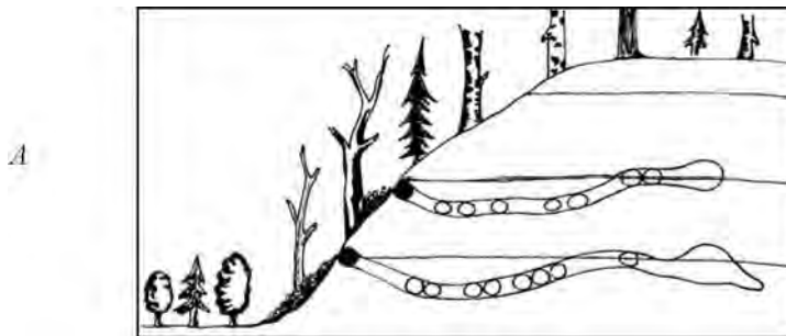
Рис. 5.7. Бобровий тип норіння: A – весняна проста нора бобра, B – схематичний план будови складної постійної нори групи бобрів, B – нора хохулі; – гніздові камери, – віддушини, – нори та відморки, – рештки ґрунту з нір ссавців, – нора з підпором водного горизонту.
