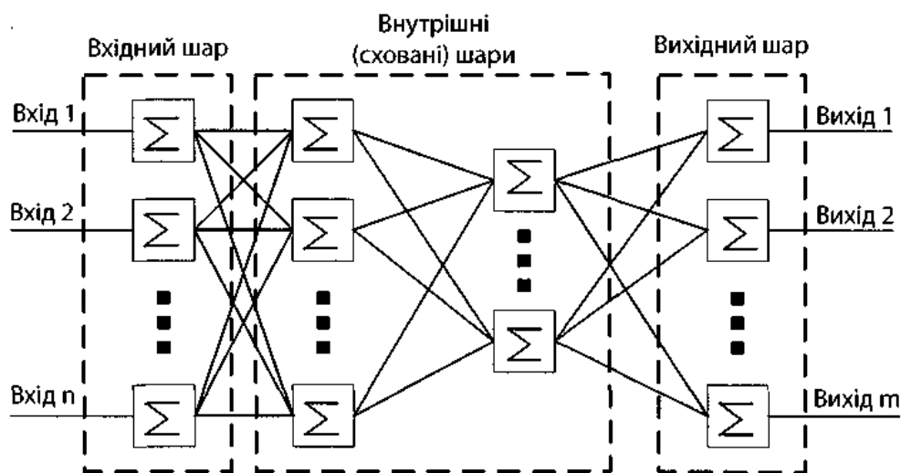
Рис. 2.9.1. Структура нейромережі
