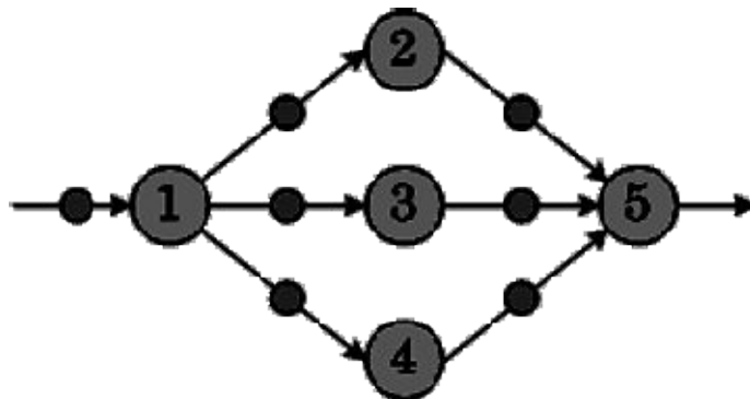
Рис. 3.8.10. Неймережа з одним входом, одним виходом і трьома елементами в прихованому шарі
