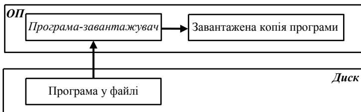
Рис. 1.4. Завантаження програми
