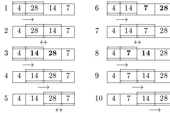
Рис. 6.1. Сортвання масиву за методом бульбашки
