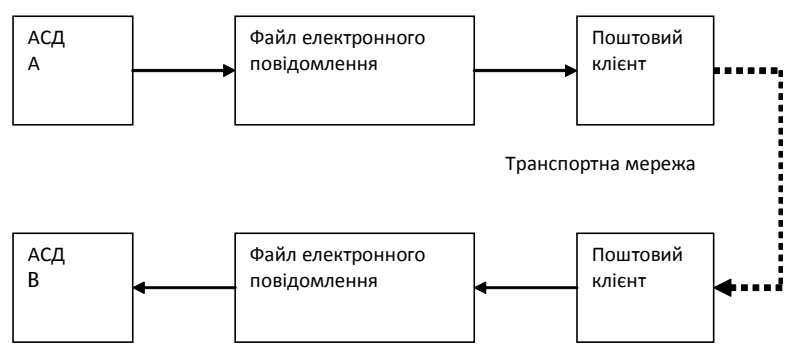
Рис. 16.8. Архітектура е-взаємодії різних автоматизованих систем
