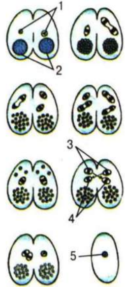
Мал. 8. Кон'югація в інфузорії-туфельки: 1 – малі ядра; 2 – великі ядра; 3 – мігруючі ядра; 4 – стаціонарні ядра; 5 – ядро, яке утворилося в результаті злиття мігруючого та стаціонарного
