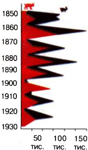
Мал. 135. Взаємопов'язані коливання чисельності популяцій хижаків і здобичі (рисі та зайця)
