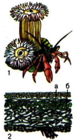
Мал. 122. Мутуалізм: 1 – актинія на черепащі рака-самітника; 2 – лишайник (а – клітини водорості, б – грибниця)
