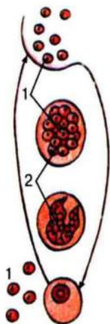
Мал. 2. Множинний поділ клітини малярійного плазмодія: 1 – клітини паразита; 2 – еритроцити
