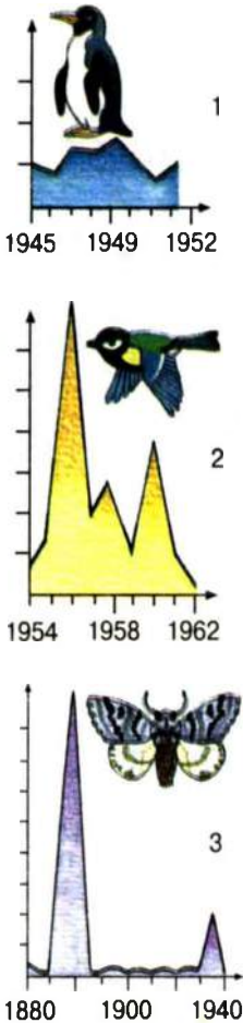
Мал. 130. Багаторічні коливання чисельності популяцій: 1 – пінгіна (особин колонії); 2 – синиці великої (пар на 10 га); 3 – соснового шовкопряда (зимуючих личинок на 100 м 2 )
