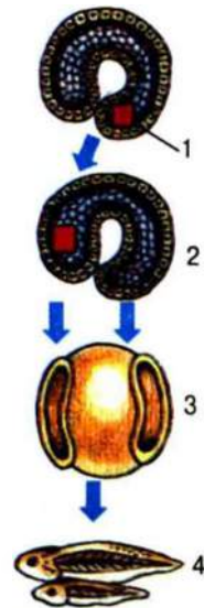
Мал. 23. Взаємовплив частин зародка, що розвивається: 1 – ділянка, що пересаджується; 2 – стадія гастрული; 3 – стадія нейрули; 4 – розвиток додаткового зародка
