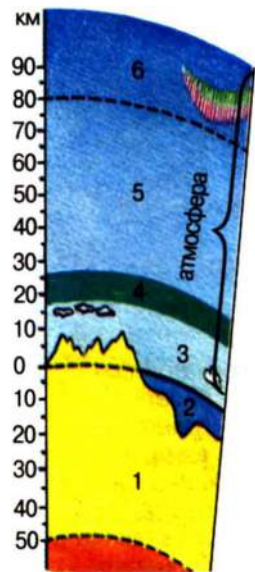
Мал. 149. Оболонки планети Земля: 1 – літосфера; 2 – гідросфера; 3 – тропосфера; 4 – озоновий екран; 5 – стратосфера; 6 – північне сяйво
