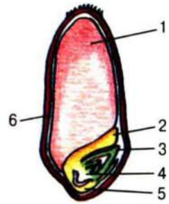
Мал. 22. Будова насінини пшениці: 1 – ендосперм; 2 – сім'ядоля; 3 – брунька; 4 – стебло; 5 – корінь; 6 – оплсдень, що зростає з насінною шкіркою
