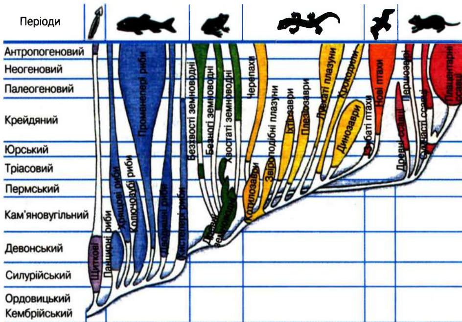
Мал. 165. Філогенетичне дерево хребетних
