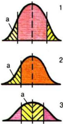
Мал. 175. Форми природного добору: 1 – стабілізуючий; 2 – рушійний; 3 – розриваючий (а – загибель особин)
