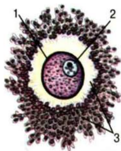
Мал. 11. Будова яйцеклітини ссавців:
