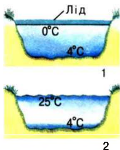
Мал. 114. Температурний режим прісного озера помірної зони: 1 – зима; 2 – літо
