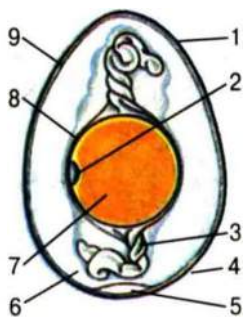
Мал. 10. Будова яйцеклітини курки:
