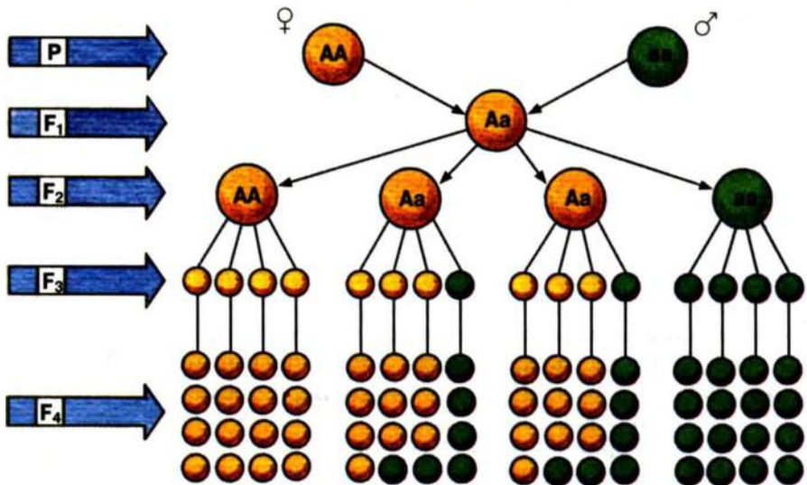
Мал. 37. Хід моногібридного схрещування гороху посівного: жовтий колір насіння – домігантний (A), зелений – рецесивний (a) стан ознаки
