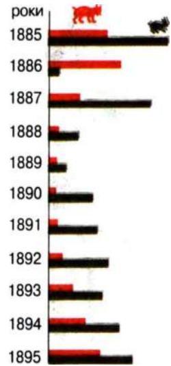
Мал. 131. Багаторічні спряжені коливання чисельності популяцій рисі та зайця
