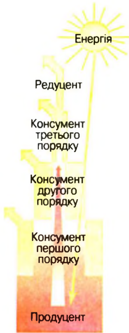
Мал. 142. Потік енергії в екосистемах
