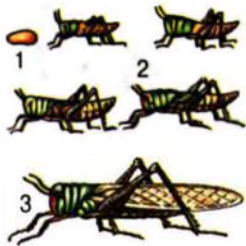
Мал. 26. Непрямої розвитку комах з неповним перетворенням (сарана): 1 – яйце; 2 – личинки різних стадій; 3 – доросла комаха
