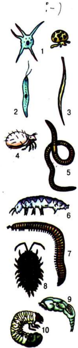
Мал. 117. Мешканці ґрунту: 1 – амеби; 2 – джгутиконосець; 3 – нематода; 4 – кліщ; 5 – дощовий черв'як; 6 – ногохвістка; 7 – багатоніжка-квісяк; 8 – мокриця; 9 – коловертка; 10 – личинка хруща
