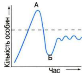
Мал. 139. Графік коливання чисельності популяції: А – спалах чисельності; Б – приведення густоти популяції у відповідність до умов середовища життя під дією регулюючих механізмів
