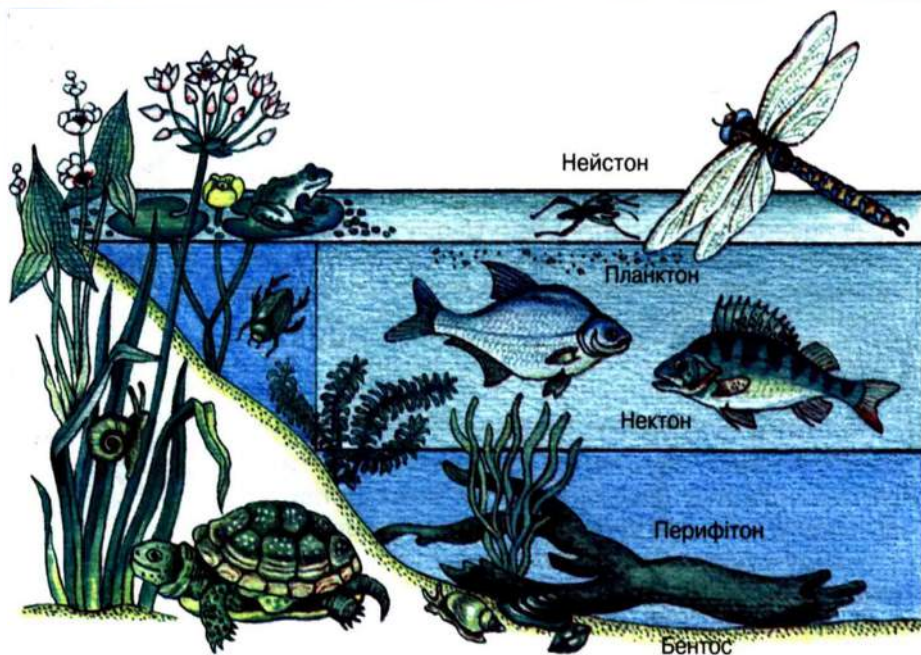
Мал. 113. Структура біоценозу озера
