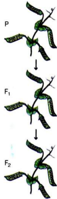
Мал. 36. Одержання чистих ліній у результаті самозапилення
