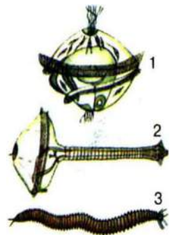
Мал. 25. Непрямий розвиток (багатошетинковий черв'як nereis): 1 – личинка; 2 – личинка, що розвивається; 3 – дорослий черв'як
