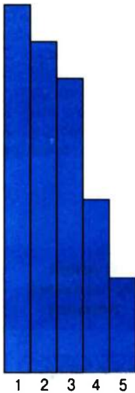
Мал. 180. Схема зниження ступеня інтеграції на різних рівнях живої матерії:
