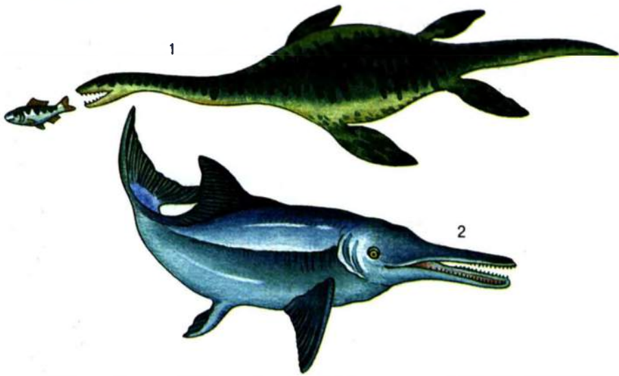
Мал. 203. Плезіозавр (1) та іхтіозавр (2)
