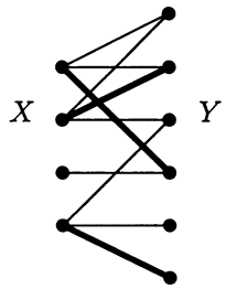
Двудольный граф с паросочетанием
