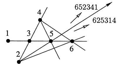
Касательный переход
