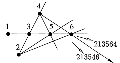
Обыкновенный переход
