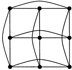
Граф S_3
