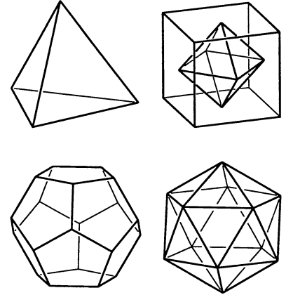
Пять платоновых тел
