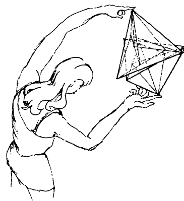
«Касание симплексов»
