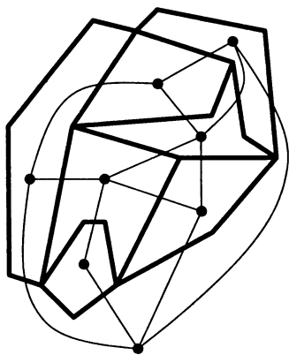
Граф, двойственный карте
