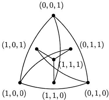
Граф G_2 : его вершинами являются все семь ненулевых троек (x, y, z) .
