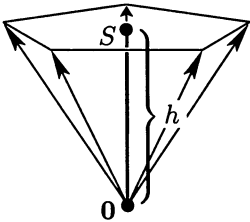
Зонт Ловаса
