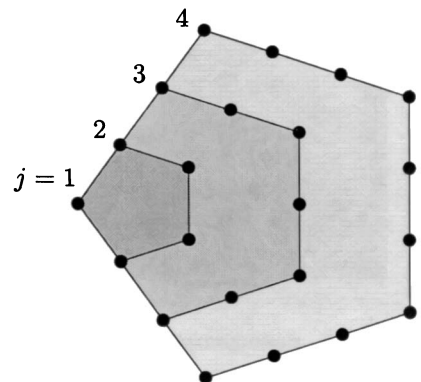
Пентагональные числа
