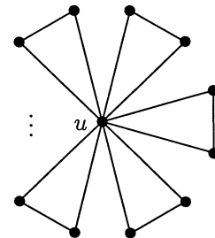
Граф-мельница
