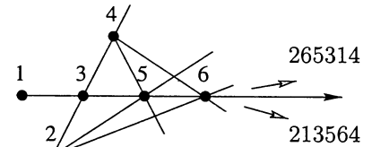
Пересекающий переход
