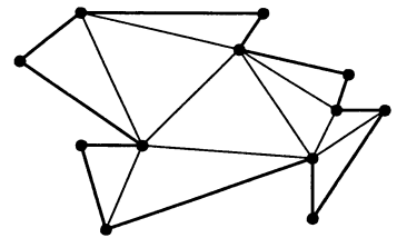
Триангуляция музея
