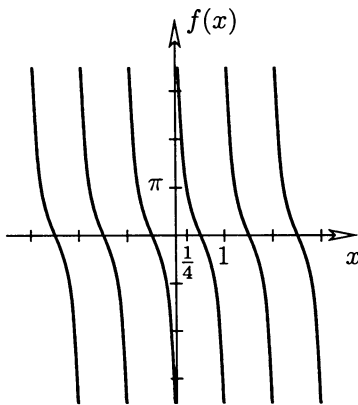
Функция f(x) = \pi \operatorname{ctg} \pi x
