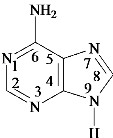
Аденін (6-амінопурин)
