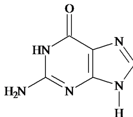
Гуанін (2-аміно-6-оксопурин)
