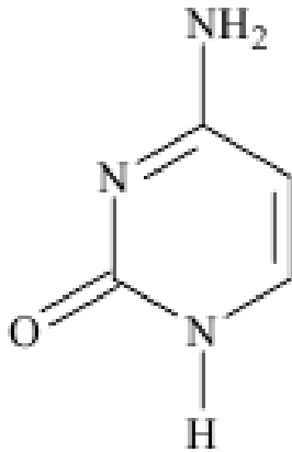
Цитозин (2-оксо-4-амінопіримідин)
