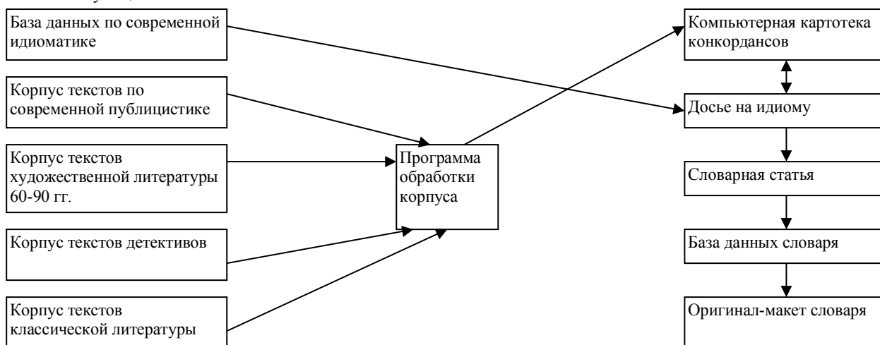
Рис. 3. Схема компьютерного обеспечения проекта Фразеологического словаря современного русского языка
