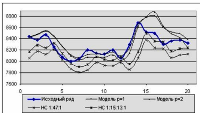
Рис. 6.9. Результати прогнозів адаптивних моделей і отриманих нейронних мереж з використанням STATISTICA Neural Networks
