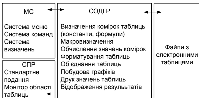
Рис. 4.12. Архітектура ІСППР на основі електронних таблиць
