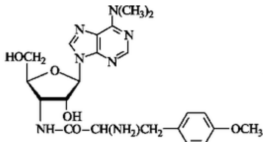
пурамицин
