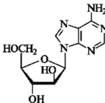
9-β-D-арабинофуранозиладенин
