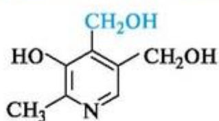
пиридоксол (пиридоксин)
