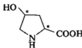
4-гидроксипролин
