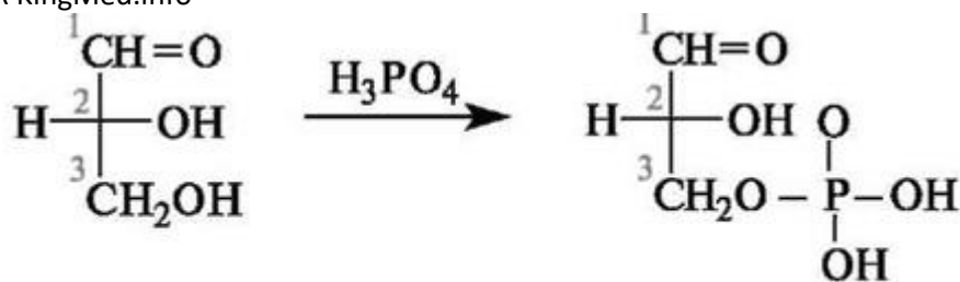
D-глицериновый альдегид
