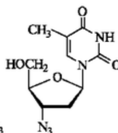
азидотимидин
