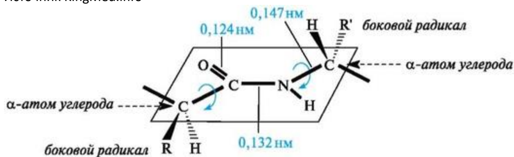
Рис. 12.1. Плоскостное расположение пептидной группы -CO-NH- и \alpha -атомов углерода аминокислотных остатков
