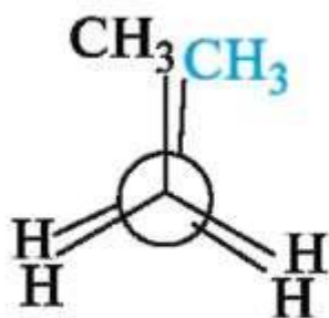
заслоненная
