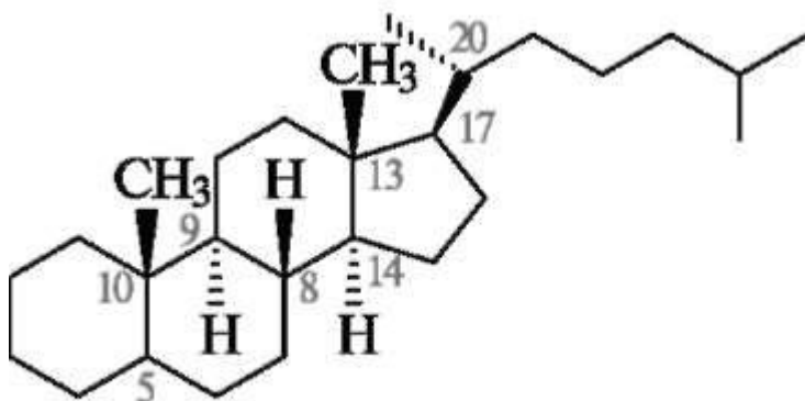
холестан
