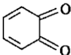
1,2-бензохинон
