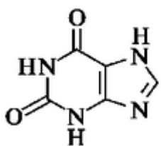
КСАНТИН
