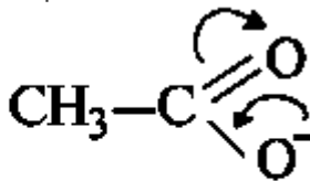
ацетат-ион
