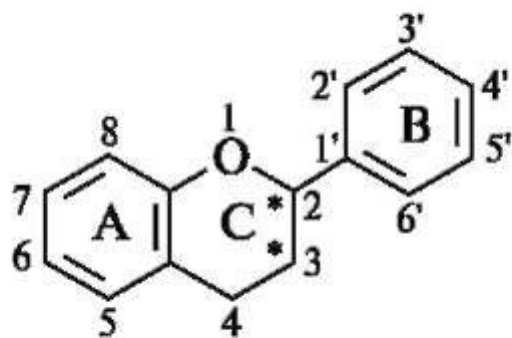
ФЛАВАН
