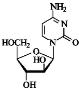
1-β-D-арабинофуранозилцитозин
