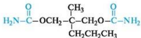
мепротан (мепробамат)
