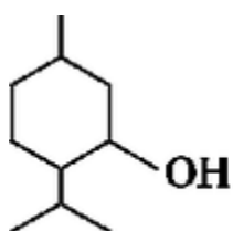
ментол
