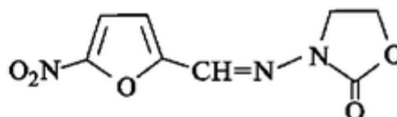
фуразолидон
