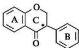
изофлаваноны
