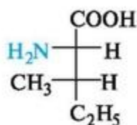
L-изолейцин
