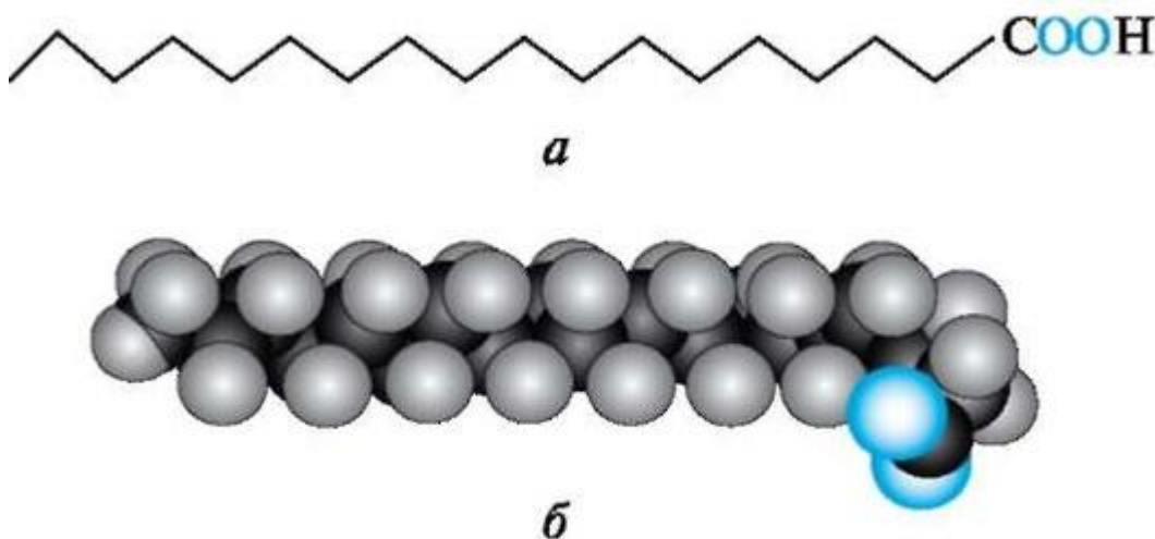
Рис. 7.6. Скелетная формула (а) и молекулярная модель (б) стеариновой кислоты
