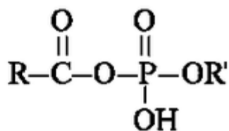
замещенный ацилфосфат
