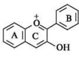
антоцианидины
