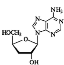
кордицепин
