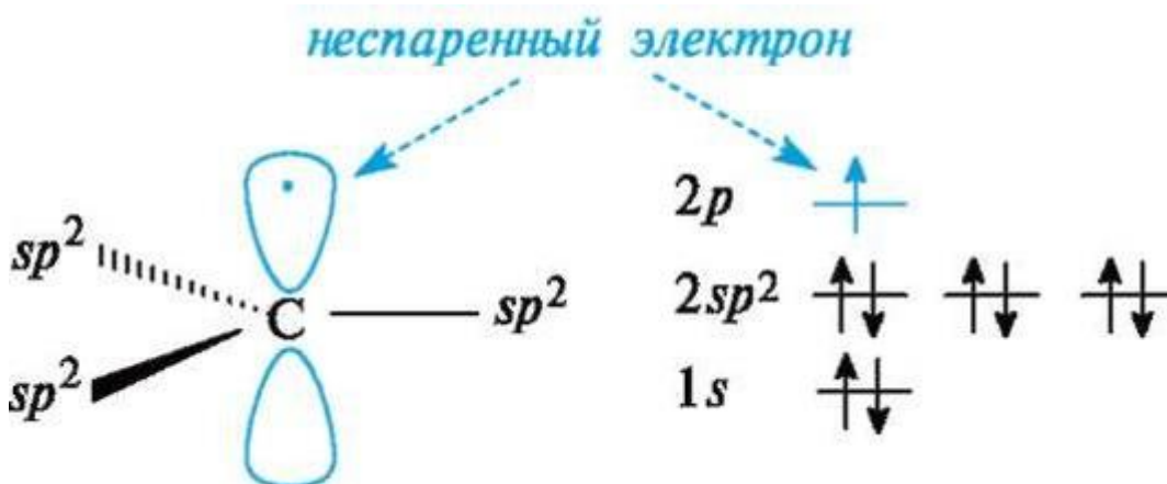
Рис. 3.1. Распределение электронов по орбиталям в свободном радикале. Высокая реакционная способность свободных радикалов объясняется их стремлением достроить внешний электронный уровень до устойчивого октета. Алкильные радикалы - короткоживущие частицы. Их относительная устойчивость соответствует ряду: третичный > вторичный > первичный.
