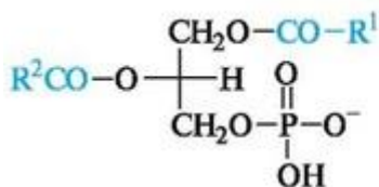
L-фосфатидовые кислоты
