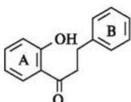
дигидрохалконы
