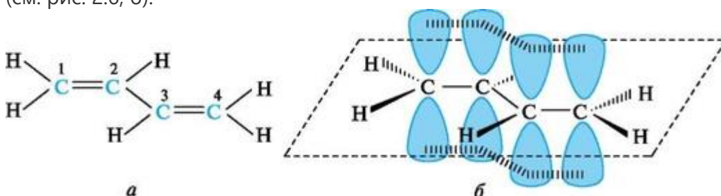
Рис. 2.6. Атомно-орбитальная модель молекулы бутадиена-1,3
