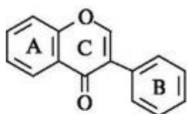
изофлавоны
