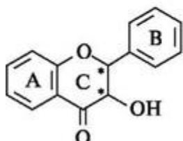
флаванонолы
