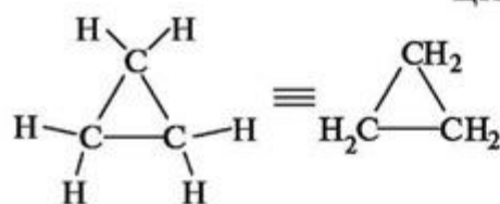
циклопропан
