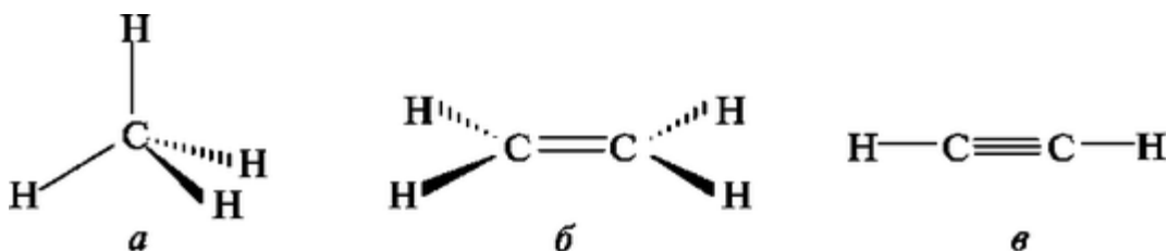
Рис. 2.3. Стереохимические формулы метана (а), этилена (б) и ацетилена (в)
