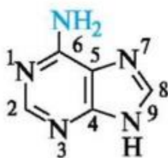
аденин Ade
