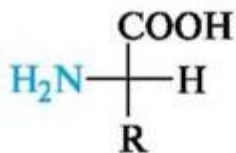
L-аминокислота
