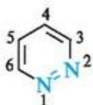
пиридазин (1,2-диазин)
