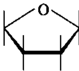
фуранозный цикл
