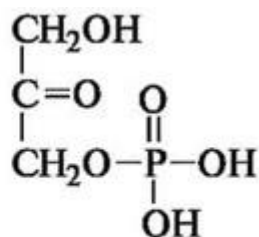
дигидроксиацетонфосфат
