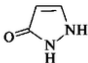
пиразолон
