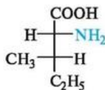
D-аллоизолейцин
