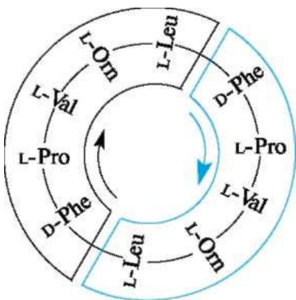
грамицидин С
