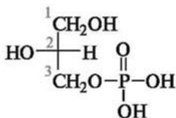
L-глицеро-3-фосфат
