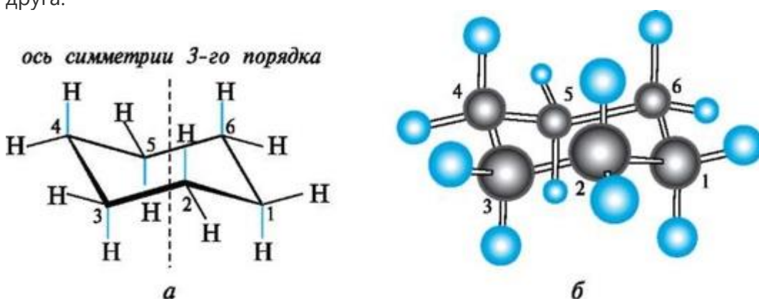
Рис. 7.7. Циклогексан в конформации кресла: a - скелетная формула; б - шаростержневая модель
