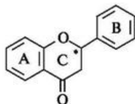
флаваноны
