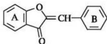
ауроны
