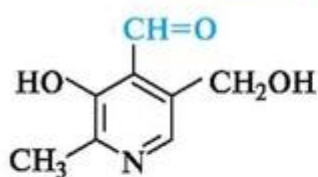
пиридоксаль
