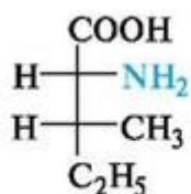
D-изолейцин
