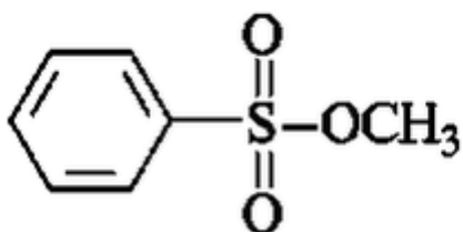
метилбензолсульфонат
