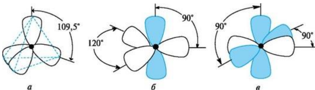
Рис. 2.2. Виды гибридизации атома углерода. Точка в центре - ядро атома (малые доли гибридных орбиталей для упрощения рисунка опущены; цветом показаны негибридизованные p -АО)
