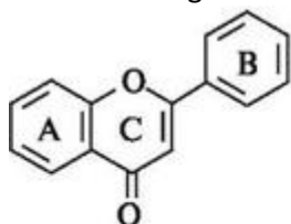
флавоны
