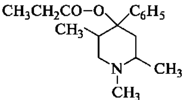
промедол
