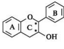
флаван-3-ола
