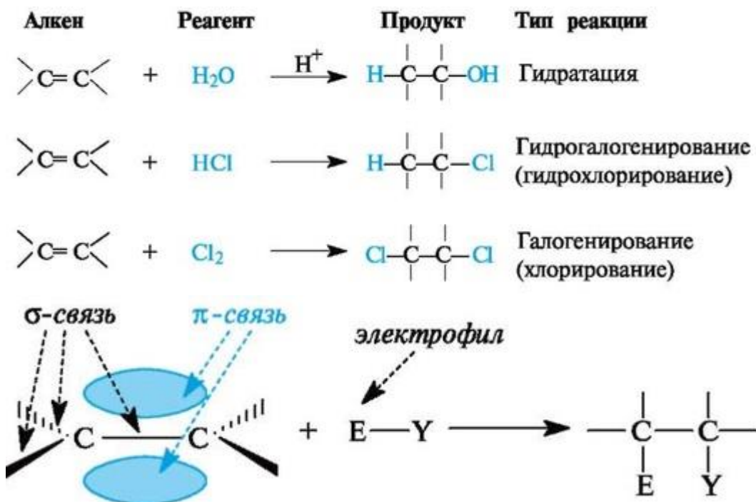
Рис. 3.3. Электрофильное присоединение с участием π-связи
