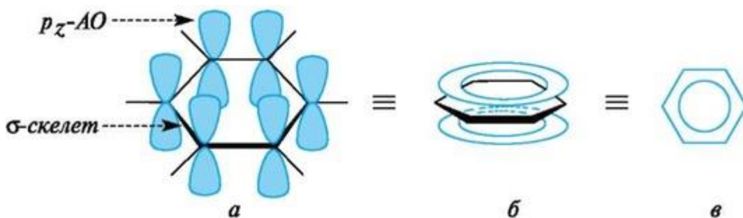
Рис. 2.8. Атомно-орбитальная модель молекулы бензола (атомы водорода опущены; объяснение в тексте)
