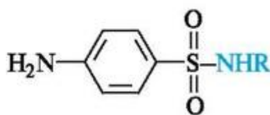
замещенный сульфаниламид
