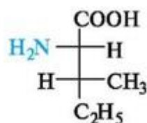
L-аллоизолейцин
