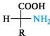
D-аминокислота
