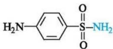
сульфаниламид (стрептоцид)
