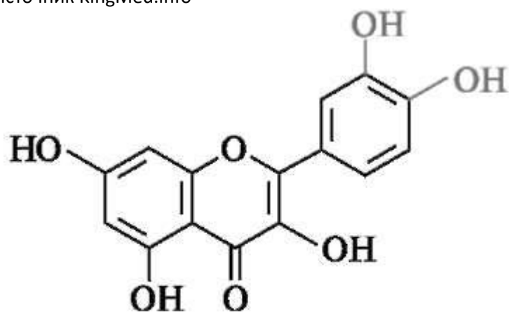
кверцетин
