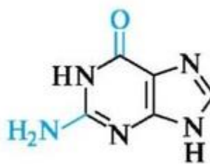
гуанин Gua
