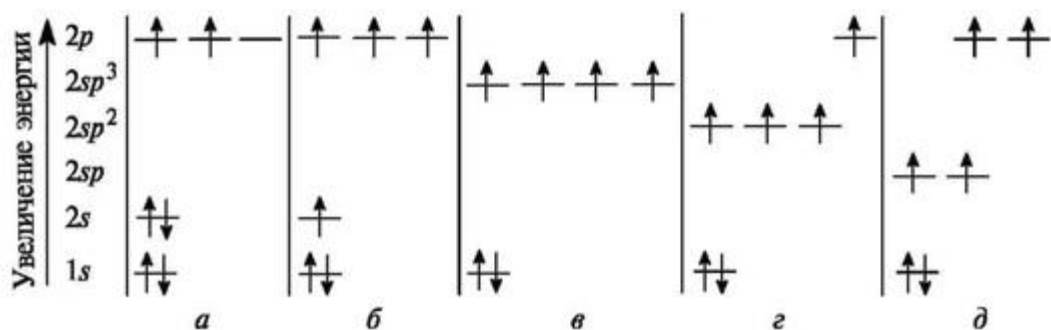
Рис. 2.1. Распределение электронов по орбиталям у атома углерода в основном (а), возбужденном (б) и гибридных состояниях (в - sp^3 , з - sp^2 , д - sp )
