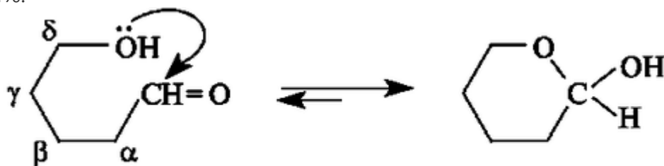
5-гидроксипентаналь
