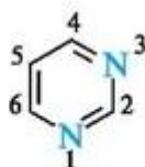
пиримидин (1,3-диазин)
