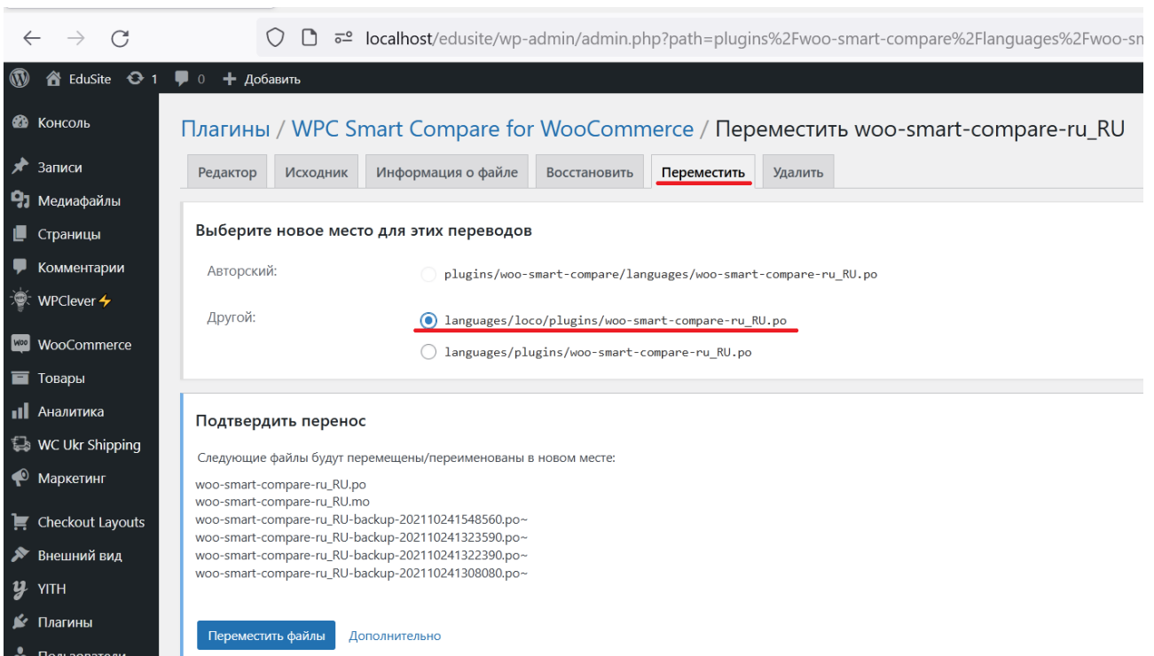
Рис. 112. Переміщення файлу перекладу у користувацький каталог
