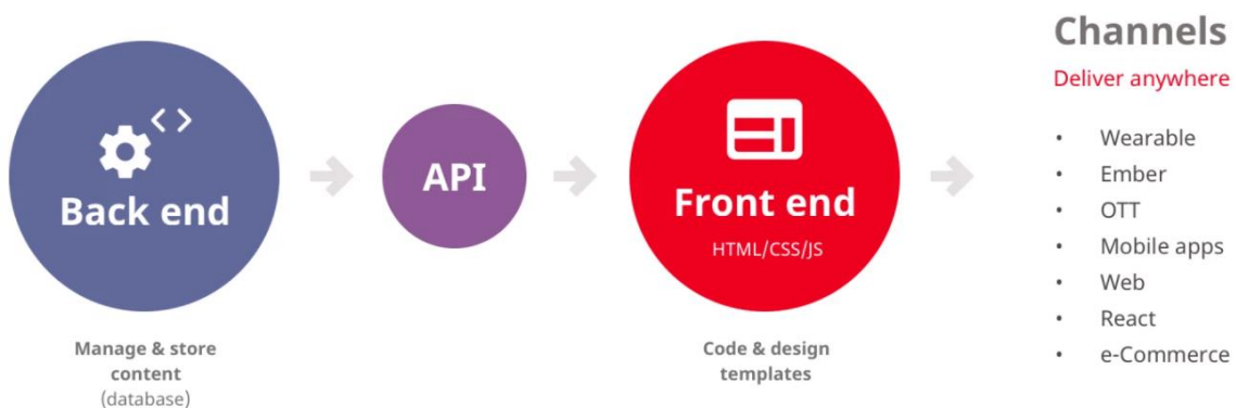
Рис. 2. Загальна архітектура розділених (decoupled) CMS
