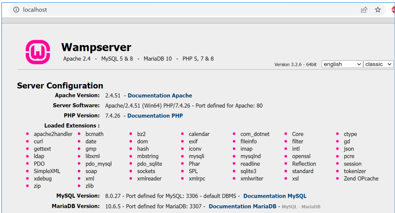
Рис. 5. Початкова сторінка WAMPServer
