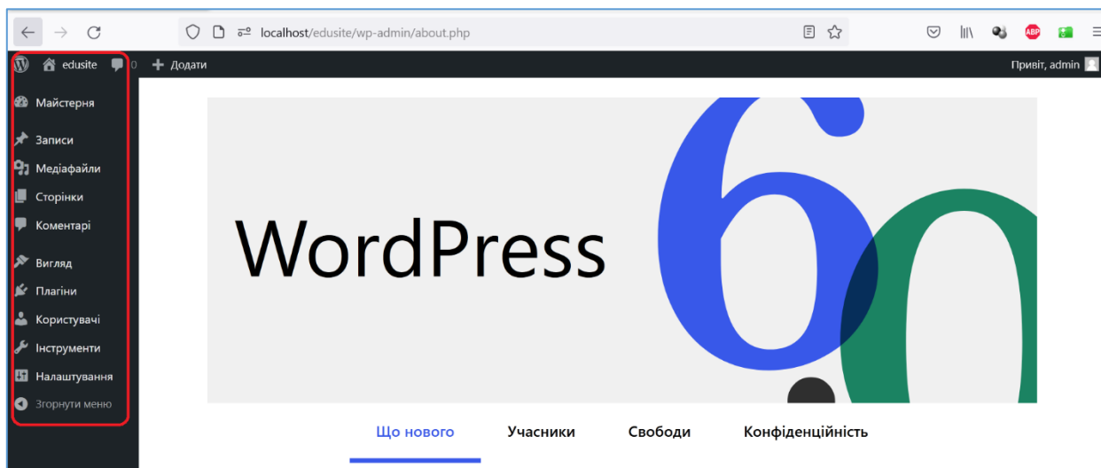
Рис. 16. Адмінпанель WordPress
