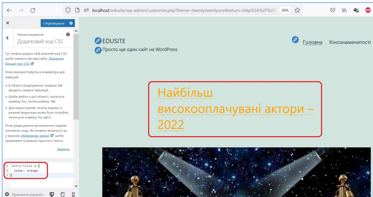
Рис. 38. Перевизначення CSS-класу
