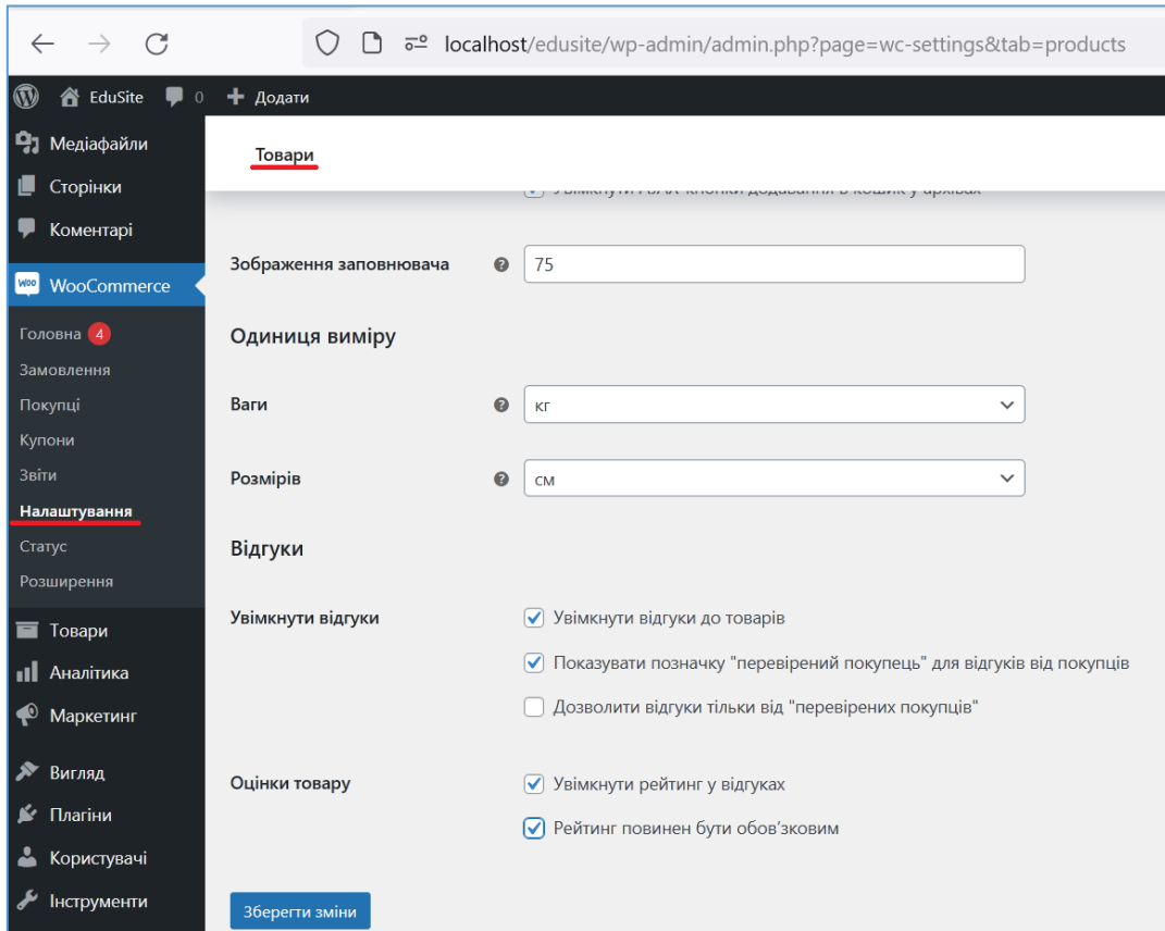
Рис. 52. Налаштування товарів
