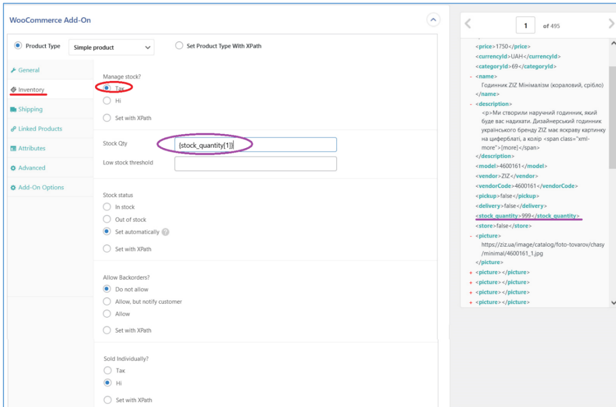
Рис. 90. Налаштування управління запасами в розділі Invenory
