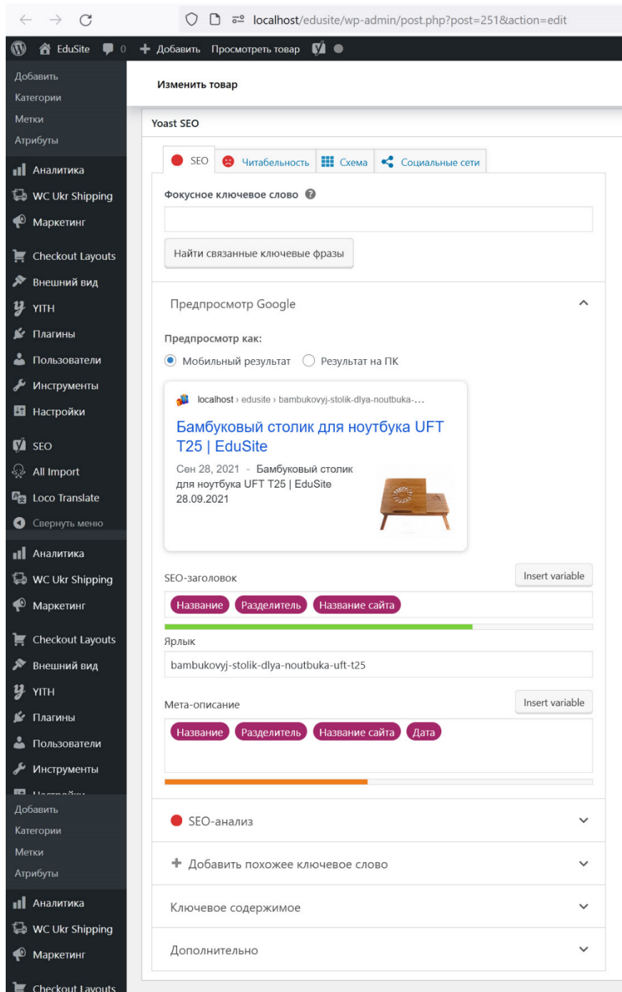
Рис. 136. Елементи управління заповнення інформації SEO на сторінці товару
