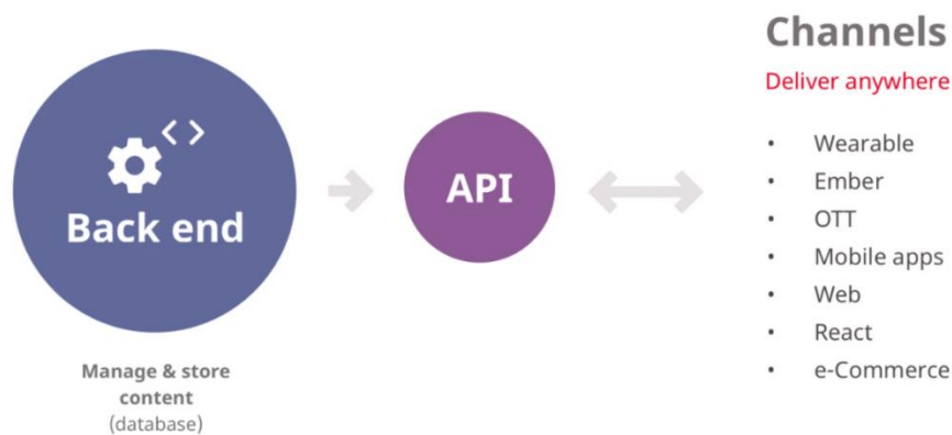
Рис. 3. Загальна архітектура безголових (headless) CMS
