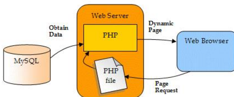
Рис. 14. Загальна структура внутрішньої організації системи керування контентом
