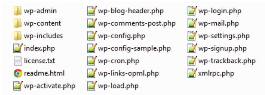
Рис. 15. Файлова структура WordPress
