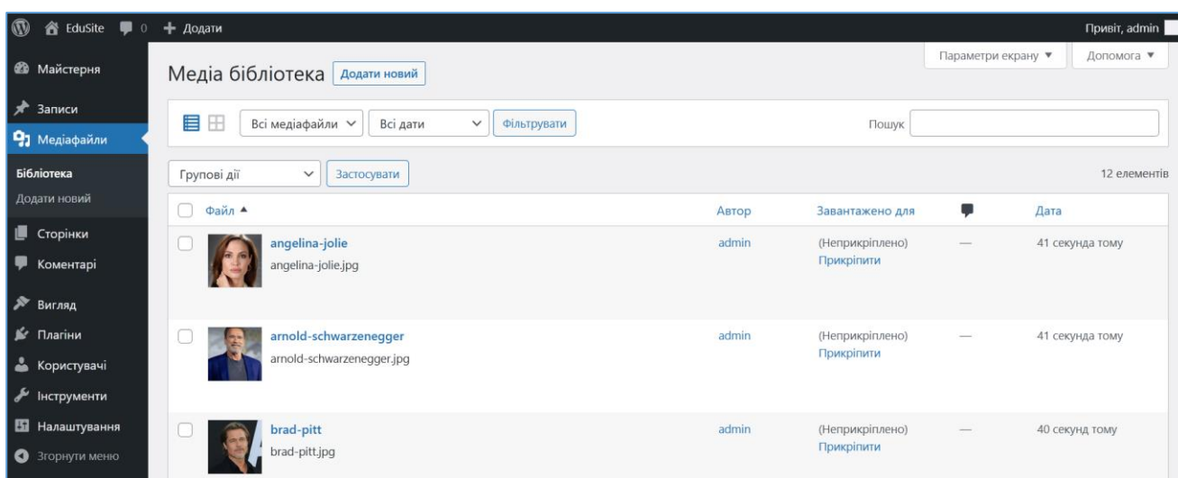
Рис. 29. Бібліотека медіафайлів
