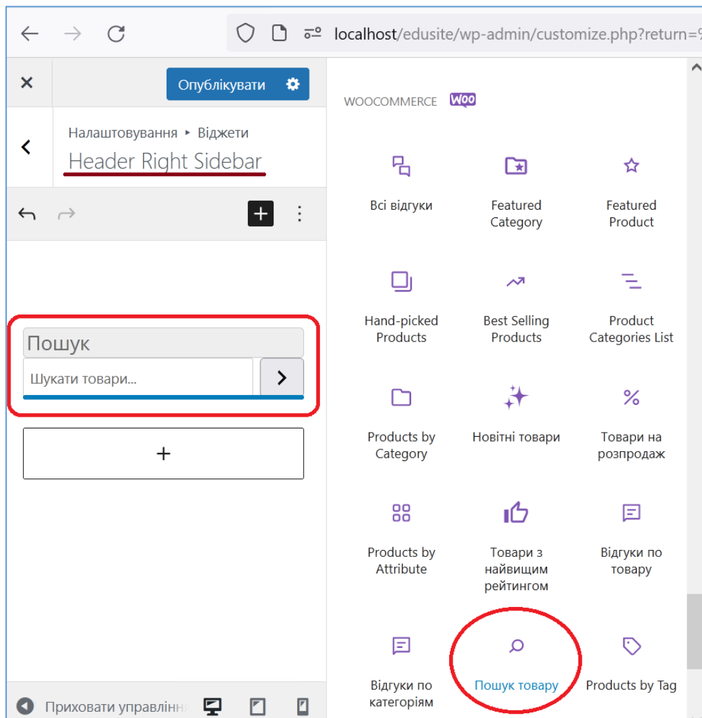
Рис. 48. Додання віджетів
