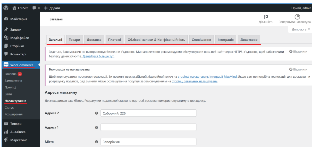
Рис. 50. Налаштування WooCommerce
