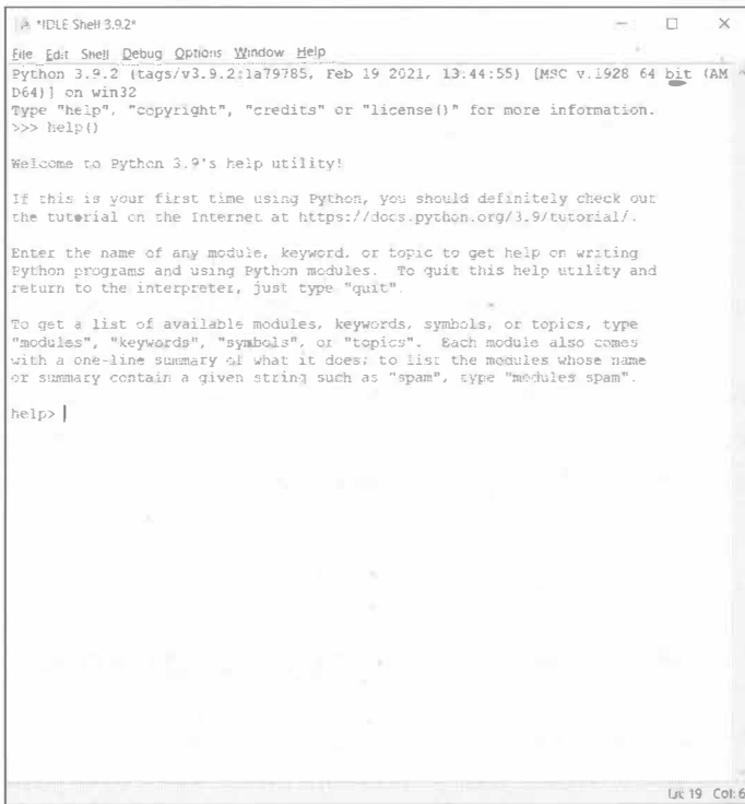
Рис. 1.7. Оболочка IDLE
