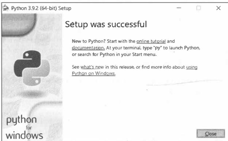
Рис. 1.5. Python 3.9.2 установлен
