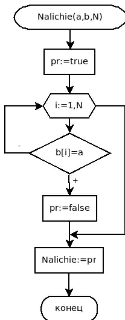
Рисунок 6.31: Блок-схема функции Nalichie
