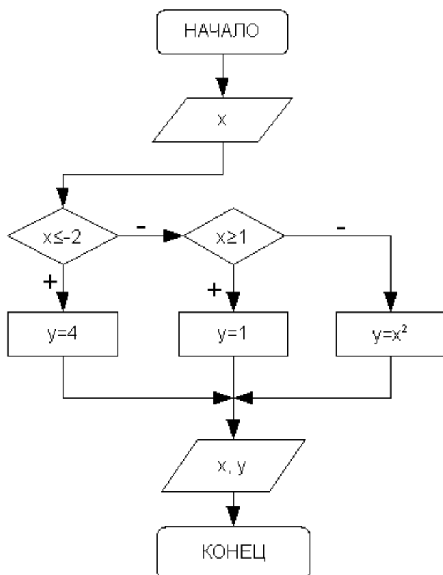
Рисунок 3.11: Блок-схема алгоритма решения задачи 3.1
