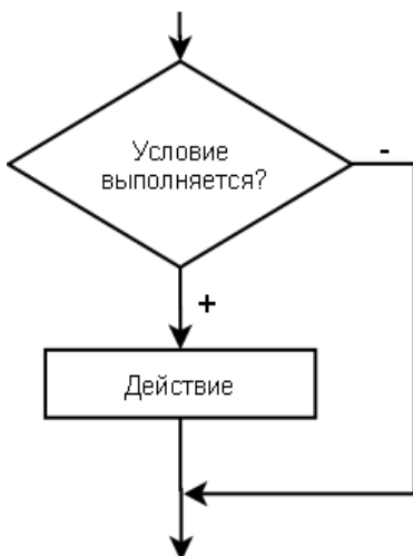
Рисунок 3.9: Алгоритм условного оператора if без альтернативной ветви else
