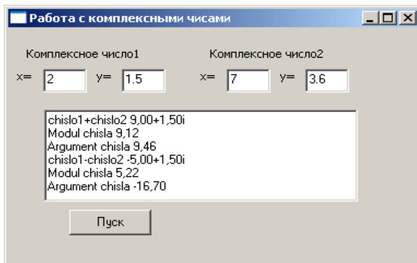
Рисунок 9.4: Пример работы программы к задаче 9.1
