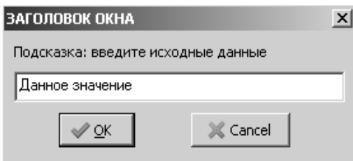
Рисунок 3.38: Окно ввода
