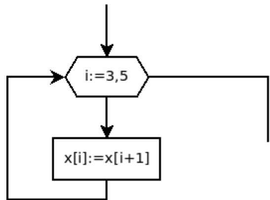
Рисунок 5.28: Алгоритм удаления 3-го элемента из массива
