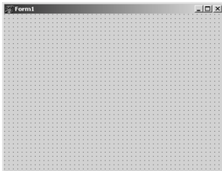
Рисунок 1.14: Окно формы
