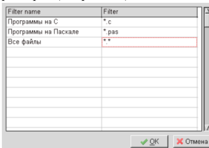
Рисунок 7.2: Редактор фильтров
