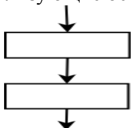
Рисунок 3.5: Линейный процесс
