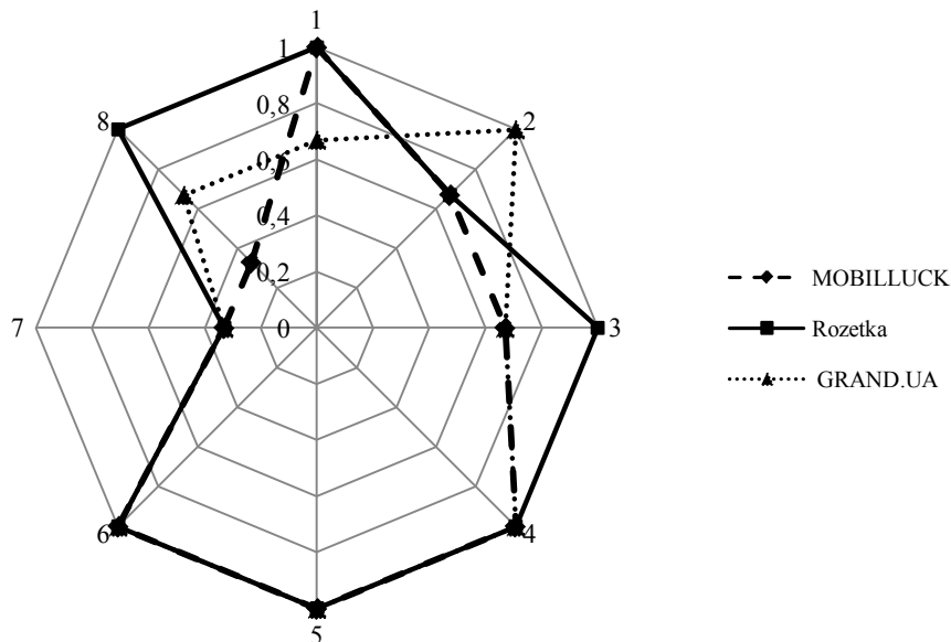
Рисунок 6 – Циклограма конкурентоспроможності
